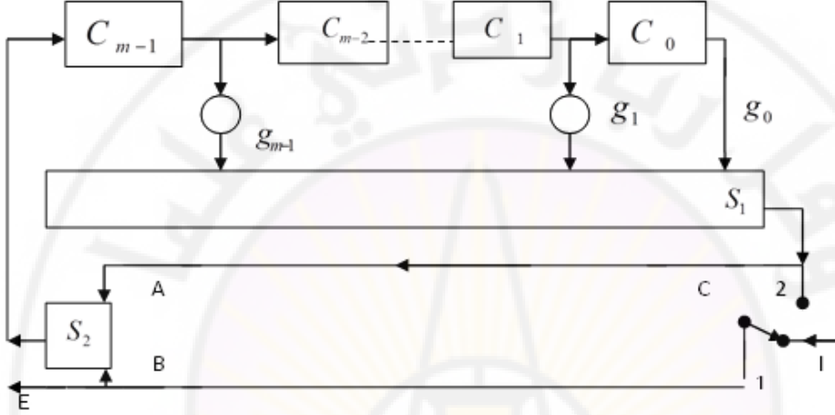
الشكل (5-10) دائرة ترميز بمسجل إزاحة ذي تغذية العكسية
