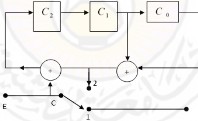
الشكل (5-13) دائرة الترميز
