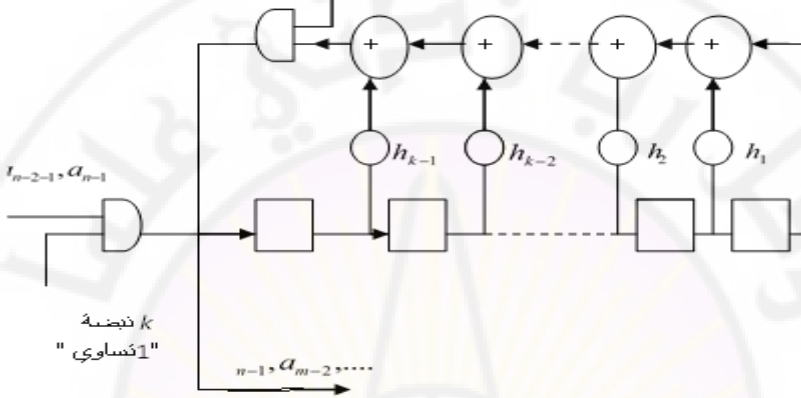
الشكل (5-17). مرمز على أساس كثير الحدود h(x)
