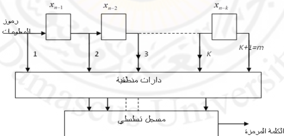
الشكل (6-1) المخطط الصنوقي لرمز انطوائي بمسجل ازاحة
