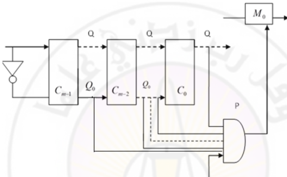
الشكل (5-12) دائرة تحسس الخطأ
