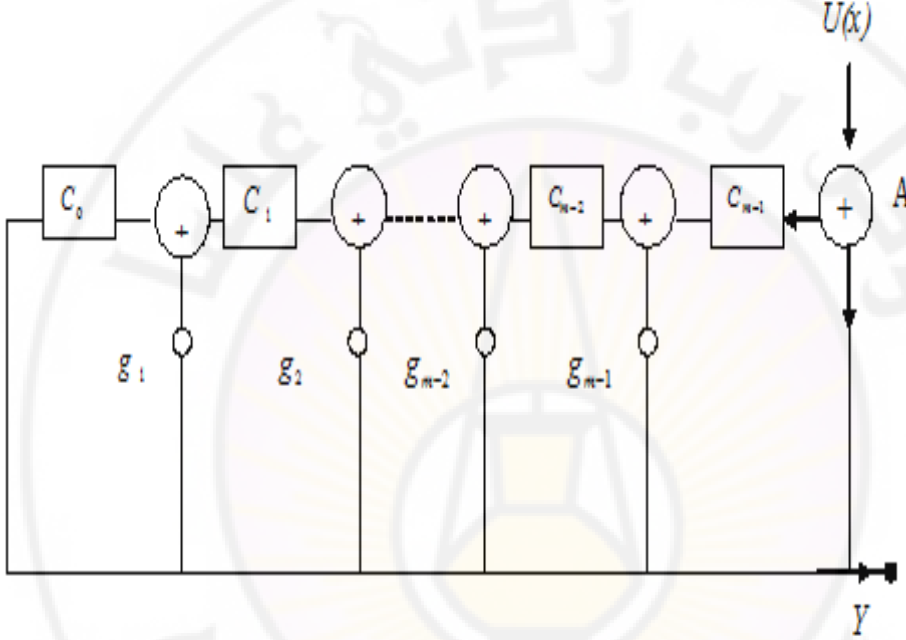
الشكل (3-5) دائرة تقسيم كثير الحدود xmu(x) على g(x)
