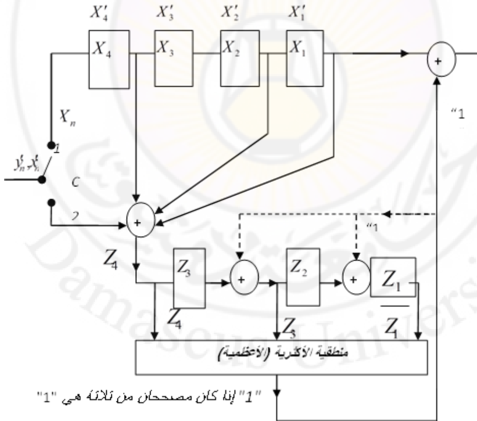
الشكل (3-6) كاشف الترميز الانطوائي
