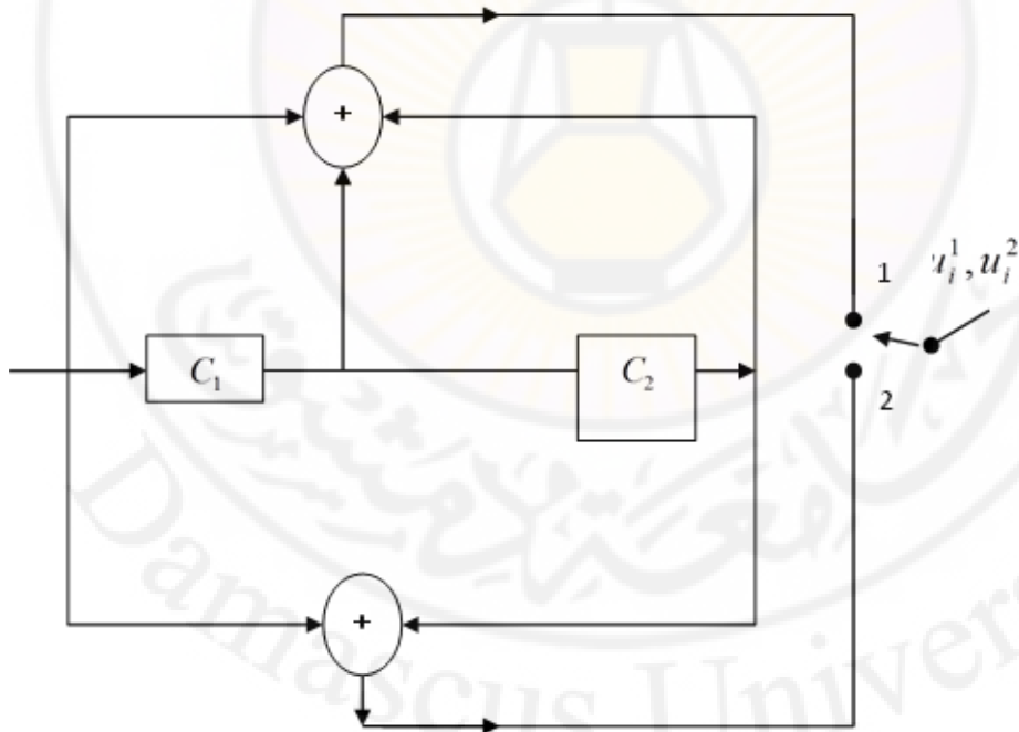
الشكل (4-6) دائرة ترميز غير نظامي m=3, n_0=2
