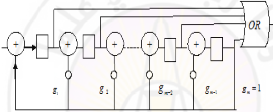
الشكل (5-5) كاشف الترميز بدائرة التقسيم
