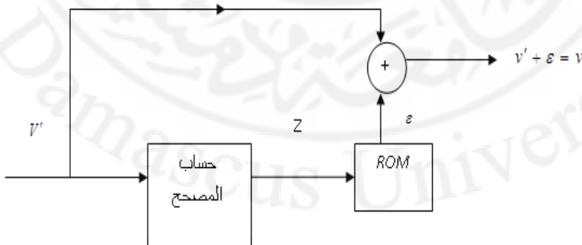
الشكل (5-1) طريقة الترميز على أساس فئات الباقي
