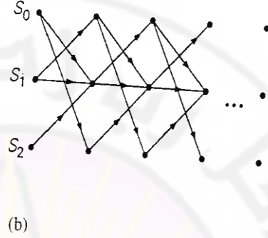
الشكل (3-4) a- مخطط الحالة، b- المخطط الشبكي
