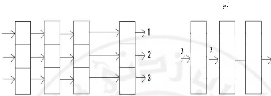
الشكل ( 5 - 19 ) مسجل إزاحة للحقل GF(2^3)
