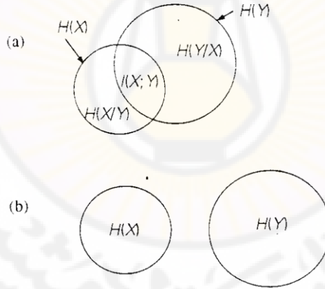
الشكل 1—5 مخطط فين يمثل العلاقات بين جميع أنواع الانتروبية
