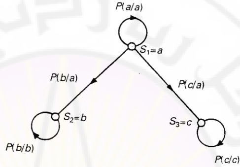
الشكل (3-5) سلسلة ماركوف غير إرغدية
