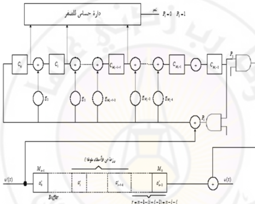
الشكل (5-15) كاشف ترميز تقنية تصحيح رزمة (باكيت) من الأخطاء
