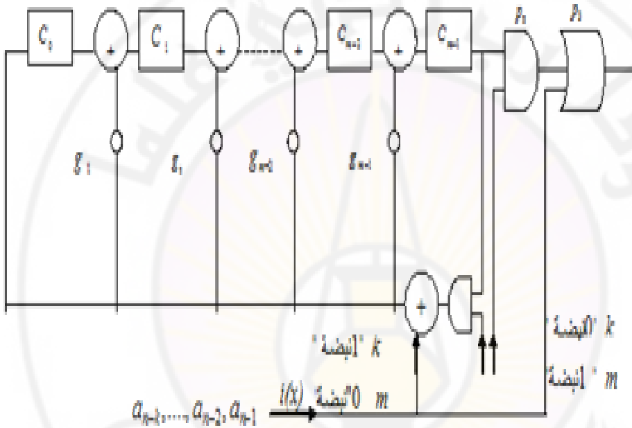
الشكل (4-5) الترميز بدارة التقسيم
