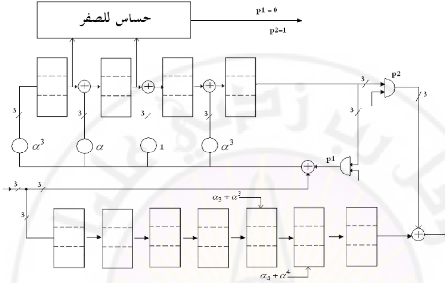
الشكل ( 5-23 ) كاشف ترميز ( R - S )
