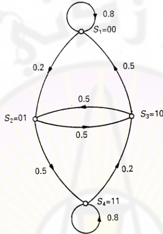
الشكل (3-3) مخطط الحالة للمثال (1-3)
