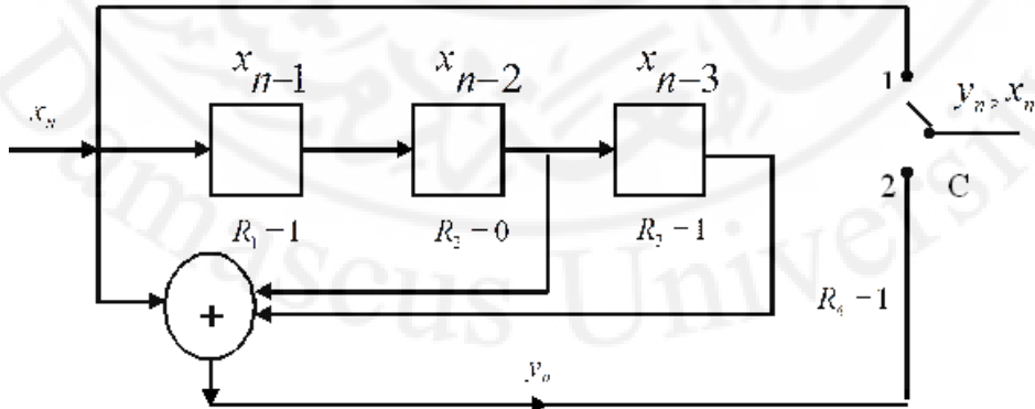
الشكل (2-6) الترميز الانطوائي
