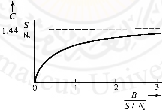
الشكل (5-3) تغيرات سعة القناة مع عرض المجال
