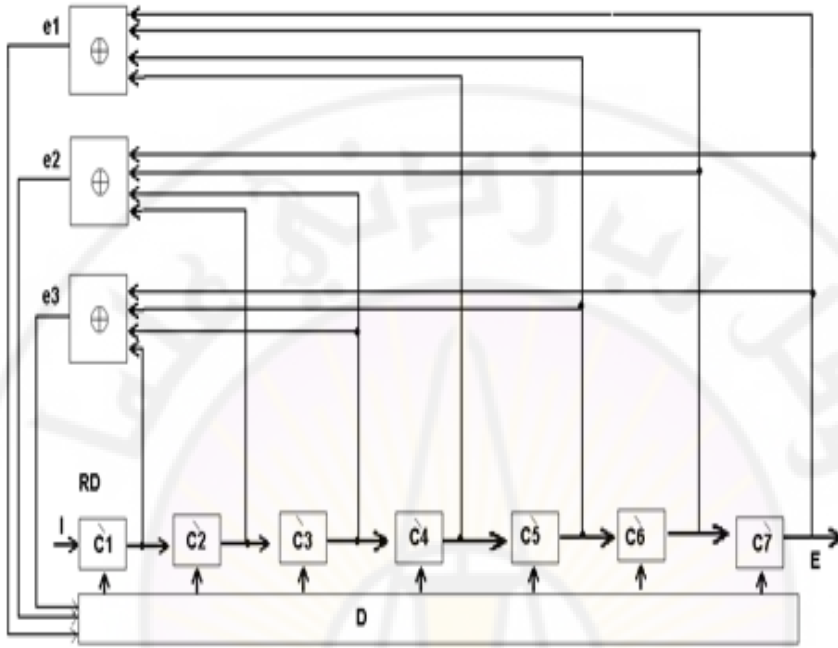
دارة كشف الترميز
