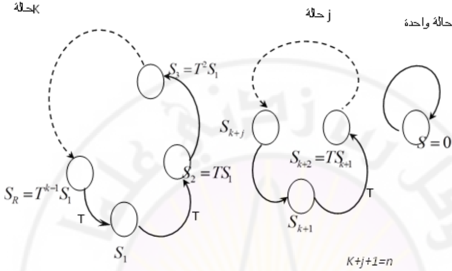
الشكل (5-8) دورات لمسجل إزاحة ذي تغذية عكسية
