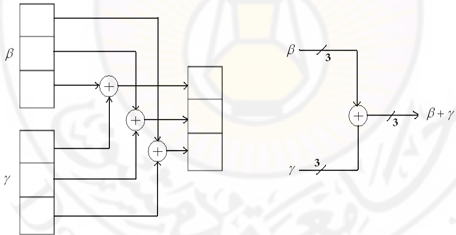
الشكل ( 5 - 20 ) جامع في الحقل GF(2^3)
