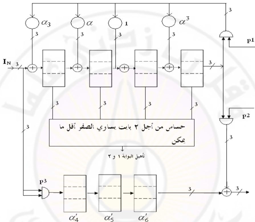
الشكل ( 5 - 24 ) كاشف ترميز لمَرَمَز R - S
