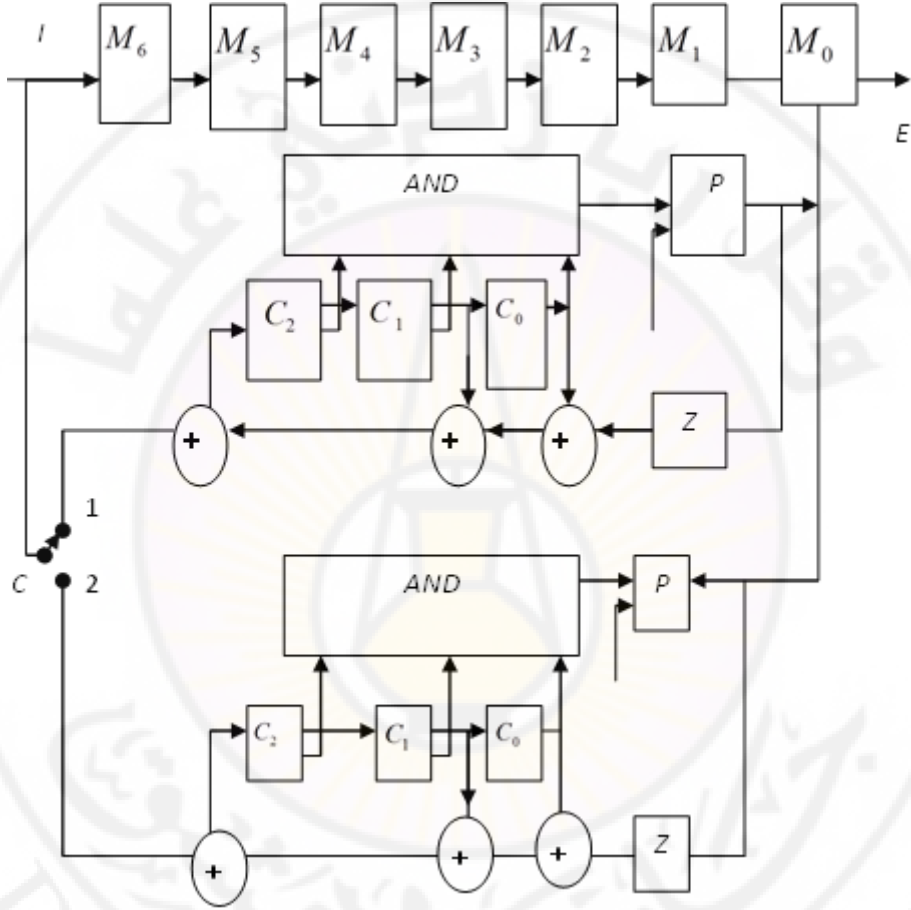
الشكل (5-14) دائرة كاشف الترميز
