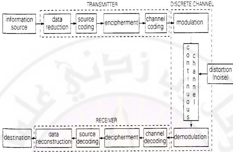
الشكل (1-8) النموذج الدقيق للاتصالات
