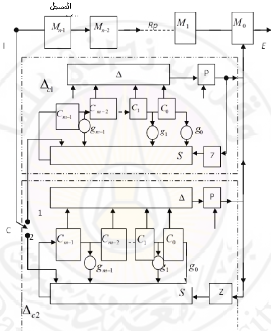
الشكل (5-11) دائرة ترميز بمسجل إزاحة ذو تغذية العكسية
