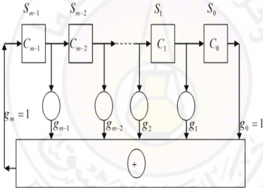
الشكل (7-5) دائرة مسجل إزاحة ذي تغذية عكسية
