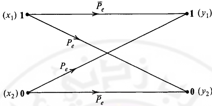
الشكل (7-3) القناة الثنائية المتناظرة
