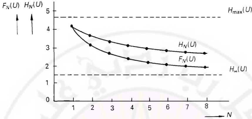
الشكل (3-6) علاقة H_N(U) و F_N(U) مع عدد الأحرف الأبجدية
