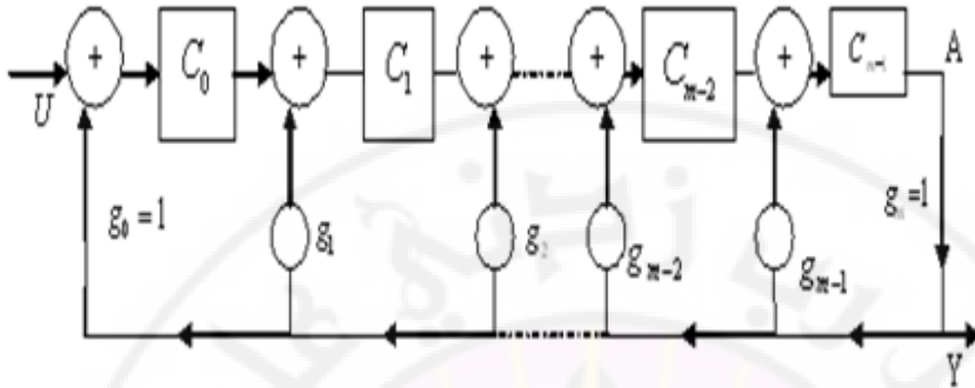
الشكل (5-2) دائرة التقسيم على g(x)
