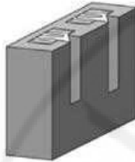
البلوك ماص للصوت - ملوء بالعازل
