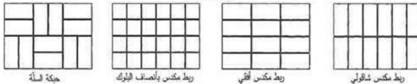
جدران غير حاملة
