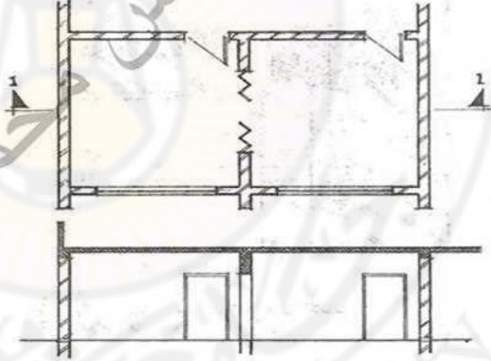
بلوك الجدران الحاملة
