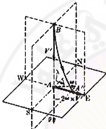
-b- نصف الكرة الشمالي
