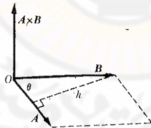
الشكل (3-20) ترتيب الأشعة في الجداء الشعاعي.
