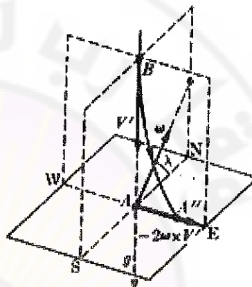
-a- نصف الكرة الجنوبي
