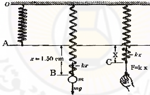
الشكل (9-8) العمل المبذول لدى شد النابض.
