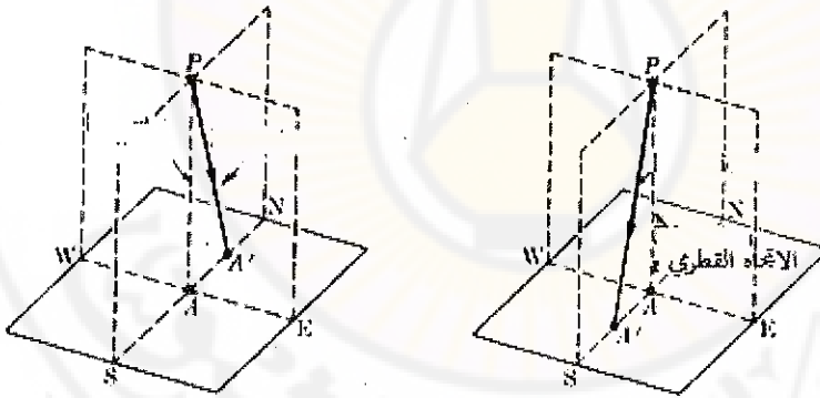
الشكل (6-9) انحراف مسار جسم ساقط سقوطاً حراً ناجم عن التسارع النابذ: نحو الجنوب (نحو الشمال) في نصف الكرة الشمالي (الجنوبي).
