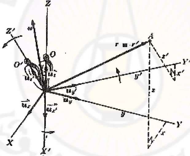
الشكل (6-5) جملتنا المقارنة في حركة نسبية دورانية منتظمة.
