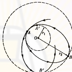
الشكل (8-24) الشكل العام للمسارات من أجل حركة تحت تأثير قوى مركزية. الشكل (8-25) اقصر مسافة اقتراب
