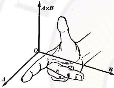
الشكل (3-21) قاعدة اليد اليمنى.
