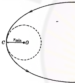
الشكل (8-24) الشكل العام للمسارات من أجل حركة تحت تأثير قوى مركزية. الشكل (8-25) اقصر مسافة اقتراب
