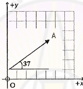
الشكل (3-5) الانتقال هو مقدار شعاعي.
