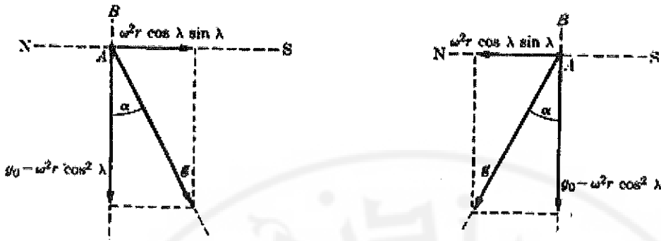
الشكل (6-8): تعريف المنحى الشاقولي والتسارع الفعلي للسقوط الحر.
