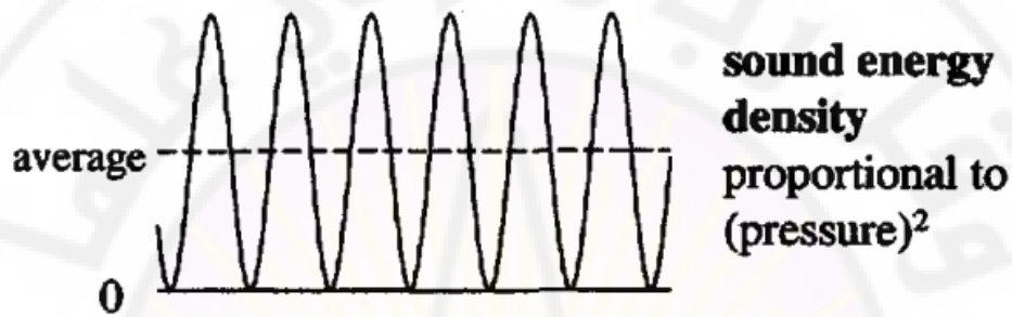
الشكل ٢,٣: معدل ضغط وطاقة الموجة الصوتية في واحدة الحجم
