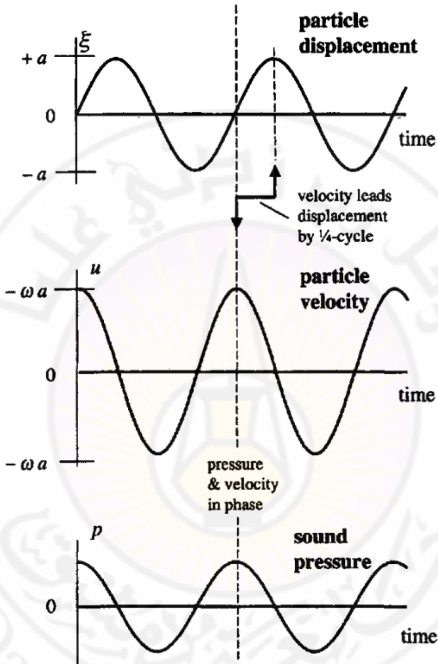
الشكل ٢,٢: شكل يوضح تمثيل إزاحة الجزيئات، سرعتها، وضغط الصوت في موجة جيبية بسيطة.
