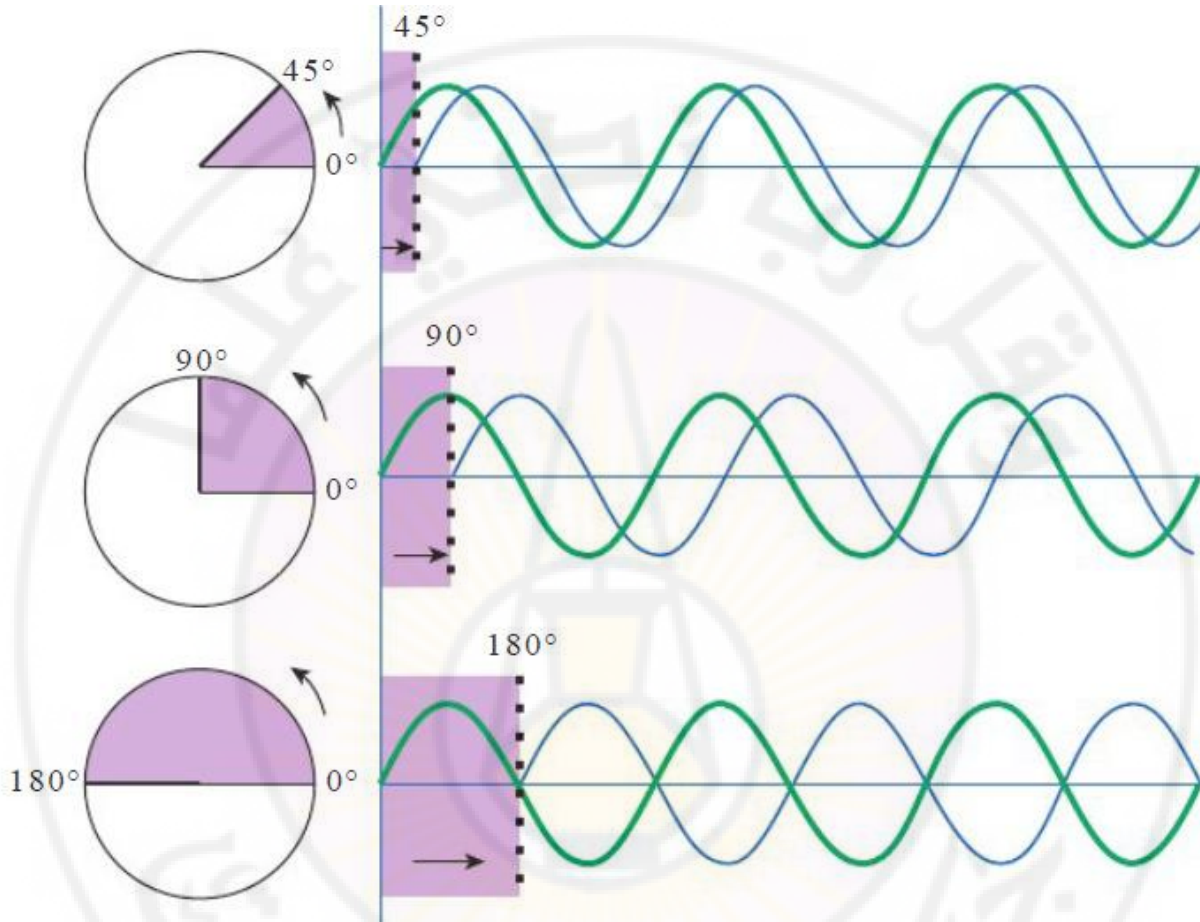
الشكل ٢،١: فرق الطور بين الأمواج الصوتية المتقدمة ومفهوم سرعة الطور.
