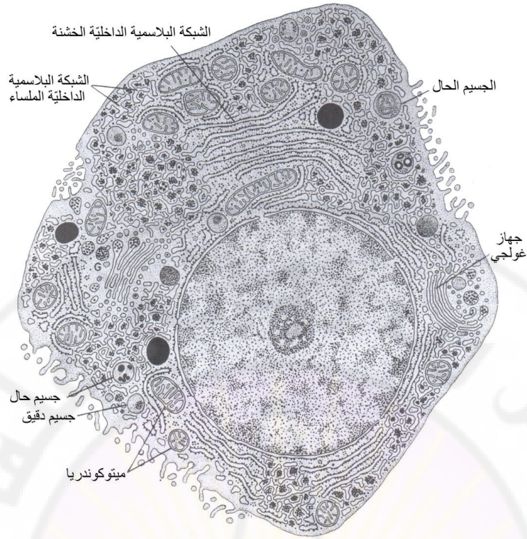
شكل تخطيطي لخلية كبدية نموذجية تبين كل من نوعي الشبكة الخشنة (RER) والشبكة البلازمية الملساء (SER).
