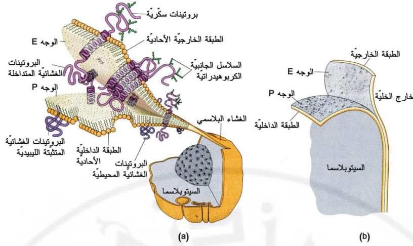
الشكل ٢: a النموذج الفسيفسائي السائل للغشاء البلاسمي، b شكل تخطيطي يمثل بنية الغشاء البلاسمي كما تظهر بالمجهر الإلكتروني الماسح.
