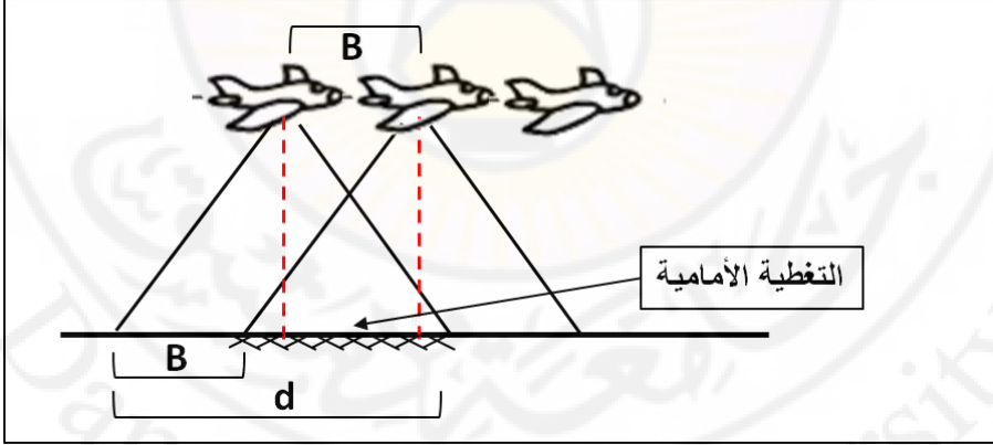
شكل (36): كيفية حساب التغطية الأمامية
