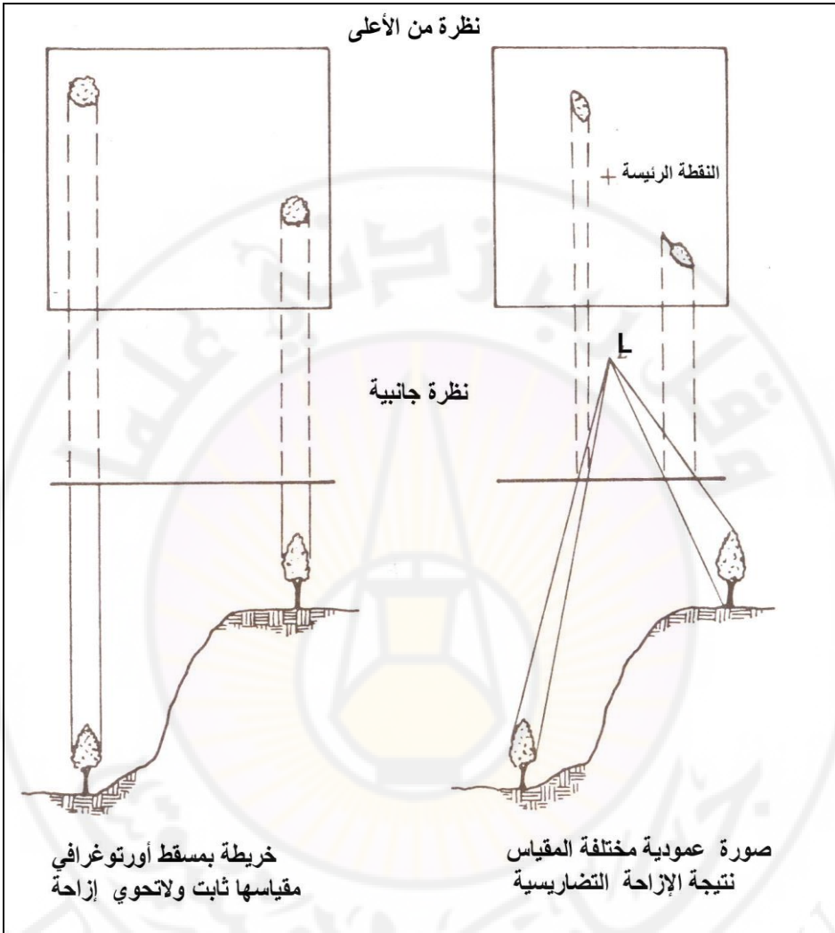
شكل (44): الإزاحة التضاريسية ومقارنة بين المظاهر الأرضية عند إسقاطها على الخريطة والصورة الجوية
