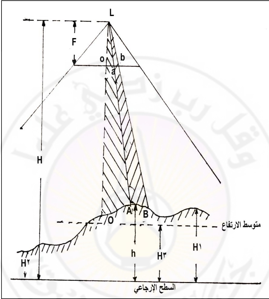
شكل (43): اختلاف المقياس على الصورة الجوية في مناطق مختلفة التضاريس (عن wolf 1974)
