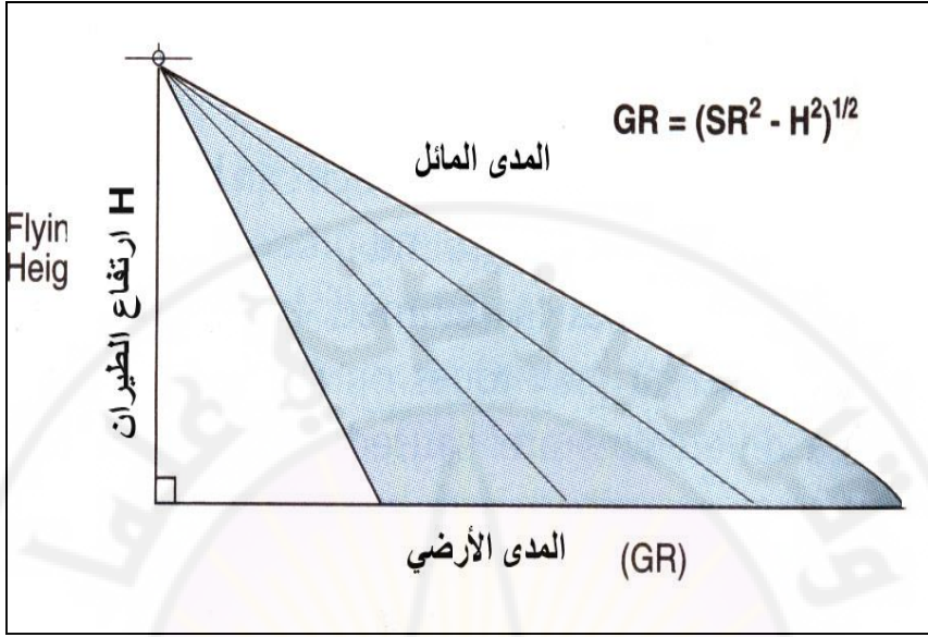
شكل (72): العلاقة بين مدى الانحراف والمدى الأرضي وارتفاع الطيران
