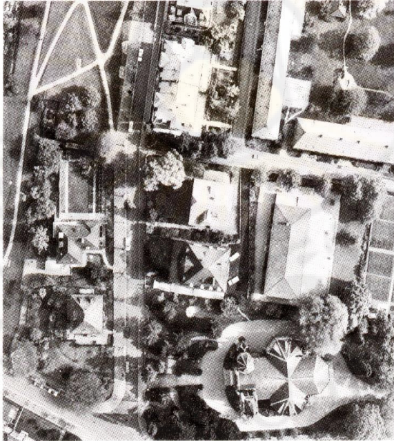
شكل (50): تأثير موقع الظاهرة من النقطة الرئيسة في الإزاحة التضاريسية في الصورة العمودية. الأبنية في A تنزاح باتجاه المركز وفي B باتجاه الأطراف
