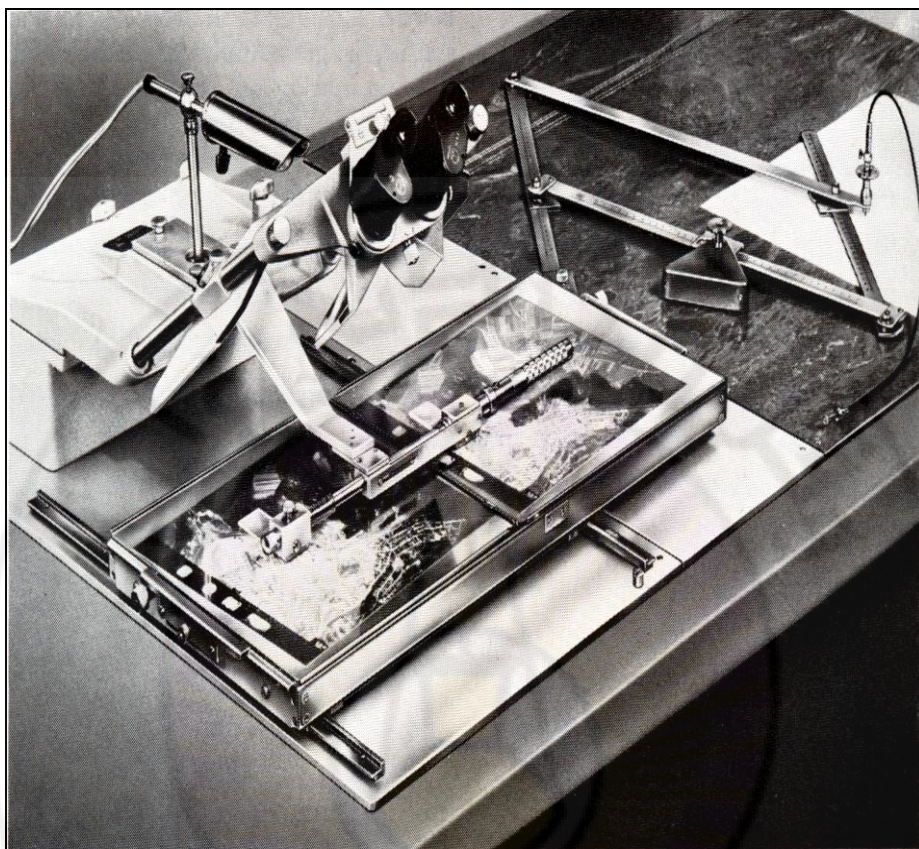
شكل (61): جهاز تفسير مجسم مزود بجهاز ستيريومتر ومانتوغراف وقلم راسم من كارل زايس Carl Zeiss Oberkochen
