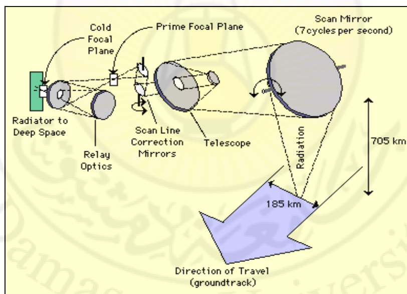
شكل (90): مكونات القمر لاندسات-7
