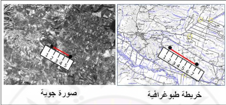
شكل (42): كيفية حساب مقياس صورة جوية بدلالة خريطة طبوغرافية
