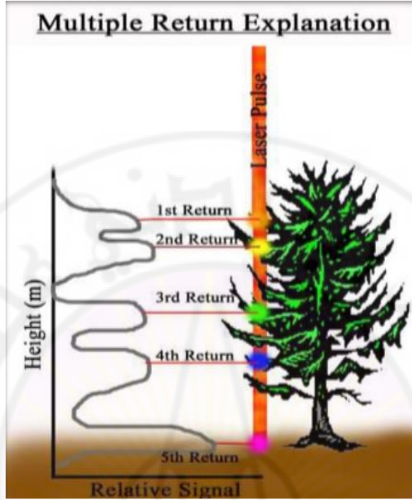
شكل (128): الارتدادات المتعددة لنبض ليزري واحد
