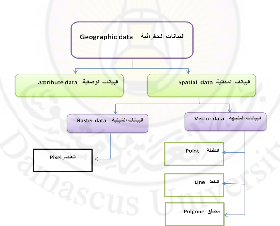
شكل (6) أنواع البيانات في نظم المعلومات الجغرافية
