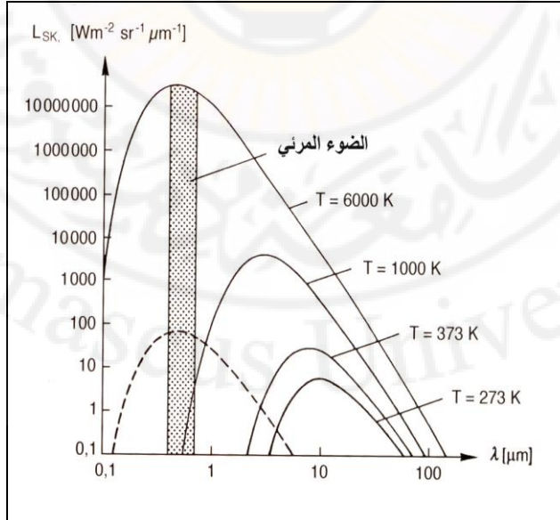
شكل (68): منحنى إشعاع الجسم الأسود
