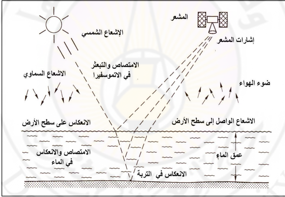
شكل (11): تفاعلات الطاقة مع الغلاف الجوي وبعض مظاهر الأرض (عن Albertz 2001)
