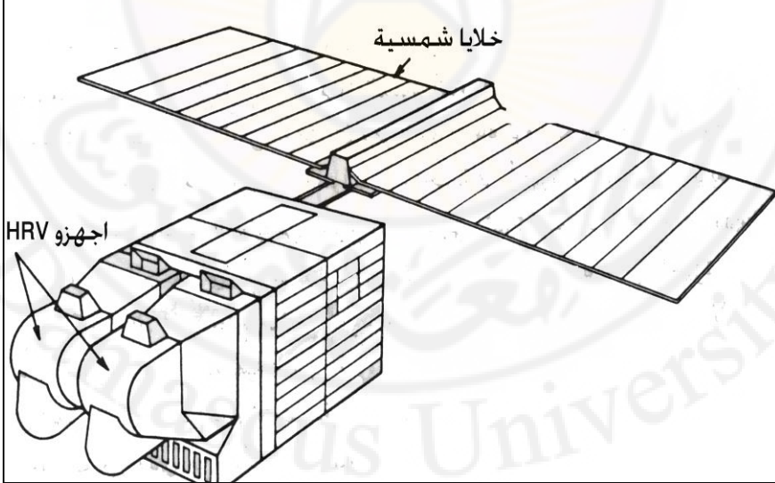
شكل (91): القمر الصناعي سبوت-1
