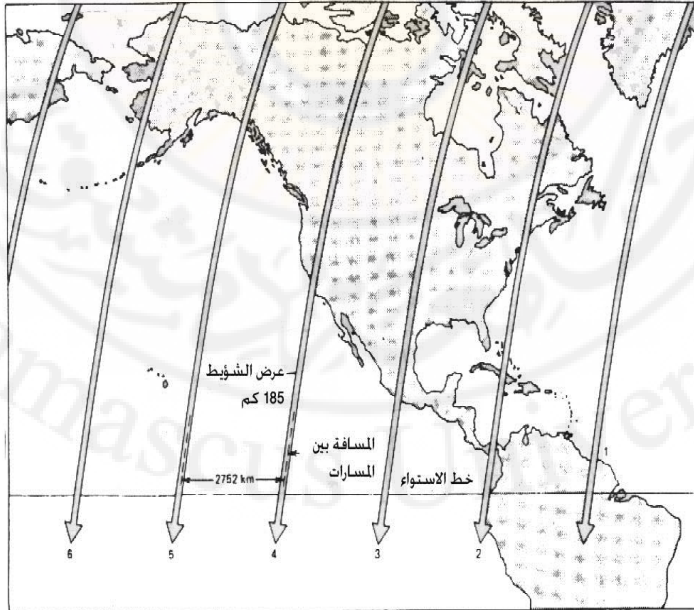
شكل (86): المسافة بين المسارات المتجاورة في لاندسات 4 و 5 تدور الكرة الأرضية مسافة 2752 باتجاه الشرق في منطقة خط الاستواء خلال الفترة الفاصلة بين مرورين (عن NASA)
