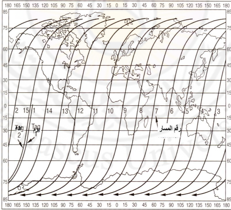
شكل (84): الحركة اليومية للاندسات 1، 2، 3
