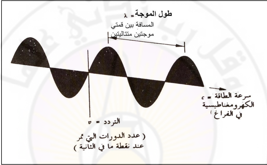
شكل (7): الموجة الكهرومغناطيسية
