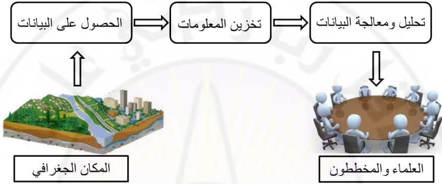
شكل (4): آلية عمل الاستشعار عن بعد
