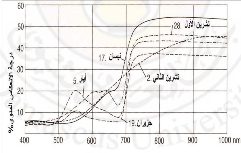
شكل (16): تغير درجة الانعكاس من أوراق البلوط خلال فترة النمو في المجال المرئي وتحت الأحمر القريب (عن Gatz 1970)
