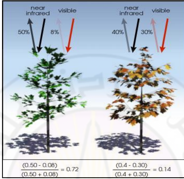
شكل (120): تطبيق مؤشر (NDVI) على النبات السليم والمصاب
