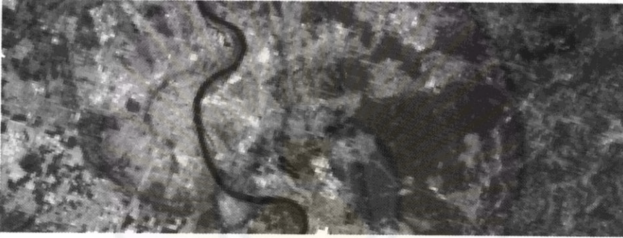
شكل (66): صورة ملتقطة بواسطة الماسح الغرضي المحمول على لاندسات عام 1992 لمدينة كولن ومحيطها في مجال الأشعة الحرارية ضمن المجال الطيفي 10-12 ميكرومتر بمقياس 1:250000
