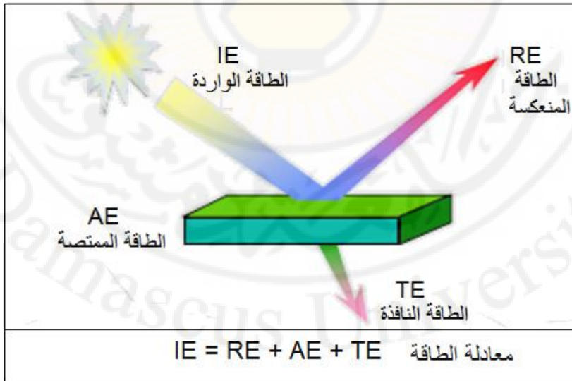
شكل (13): تفاعل الطاقة الكهرومغناطيسية مع سطح الأرض
