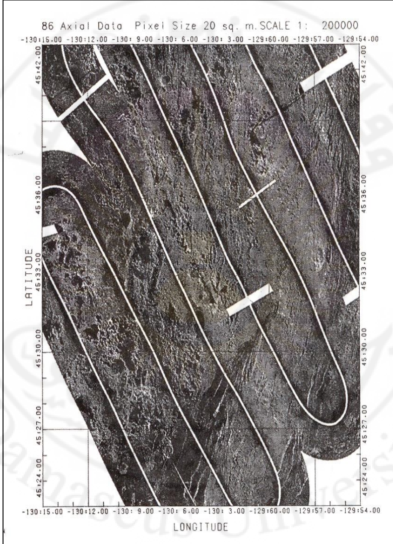
شكل (79): صورة سونوغراف لساحل Oregon تشبه صورة SLAR
