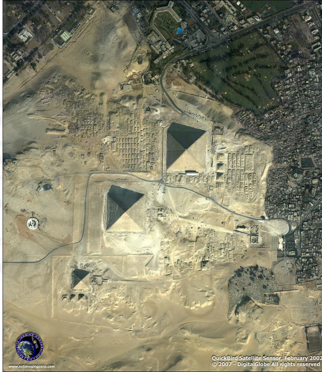
شكل (106): أهرامات الجيزة ملتقطة بواسطة القمر Quick Bird عام 2002 بقدرة تمييز 2,6 متراً
