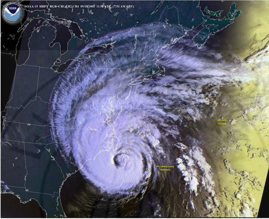
شكل (81): صورة بالأشعة تحت الحمراء لإعصار إيزابيل ملتقطة بواسطة NOAA-15 في 18 أيلول 2003
