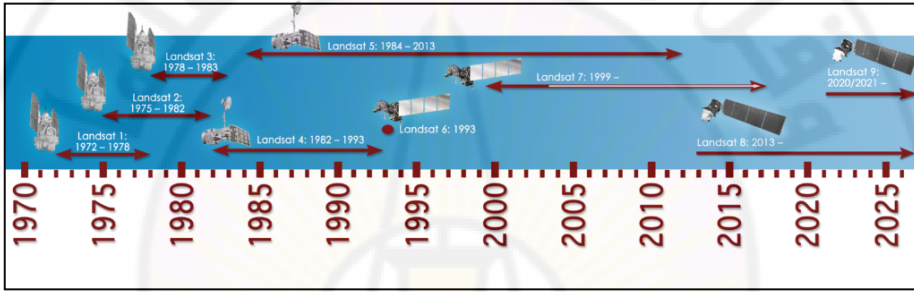
شكل (82): المخطط الزمني لإطلاق أقمار سلسلة لاندسات
