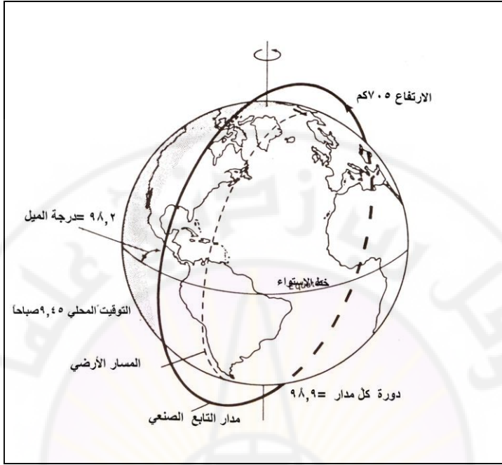
شكل (85): مدار قمري لاندسات 4 و 5 المتزامن مع الشمس
