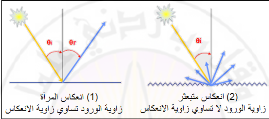
شكل (14): اختلاف الانعكاس على سطح الأرض حسب طبيعة السطح
