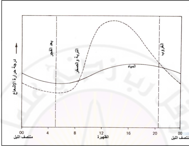
شكل (15): انعكاس كل من التربة والصخر والماء خلال 24 ساعة في المجال المرئي
