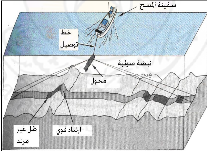
شكل (78): مكونات نظام التصوير الجانبي الصوتي
