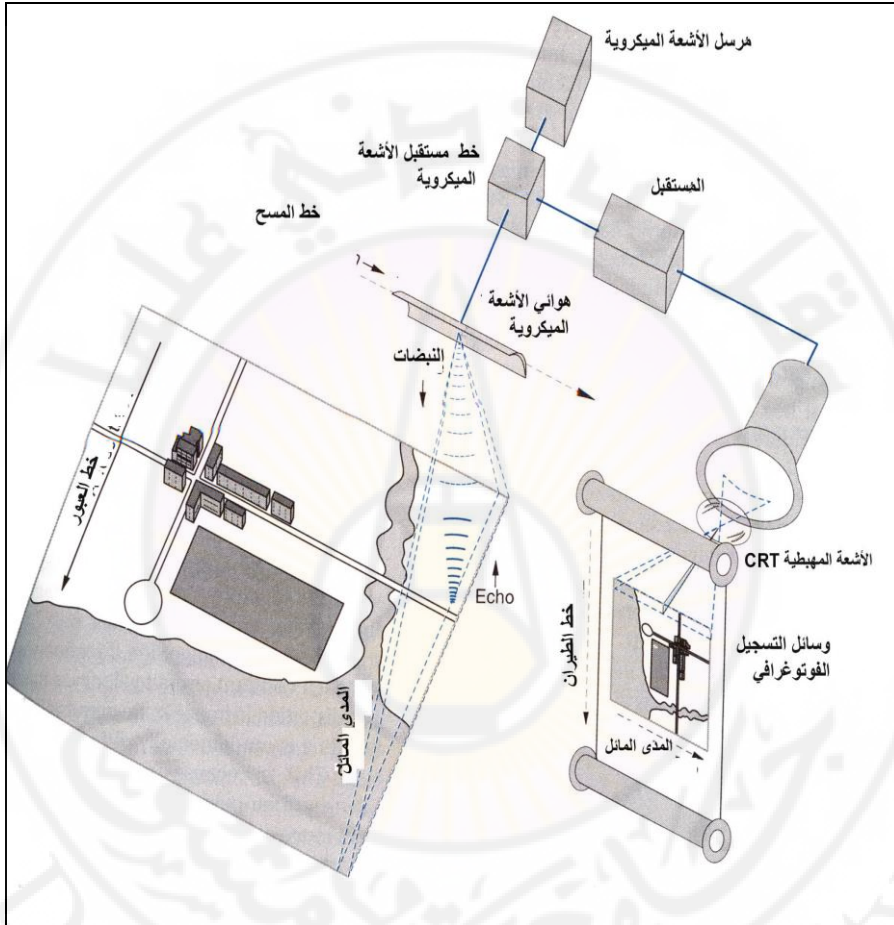
شكل (71): الرادار ذو الفتحة الجانبية SLAR
