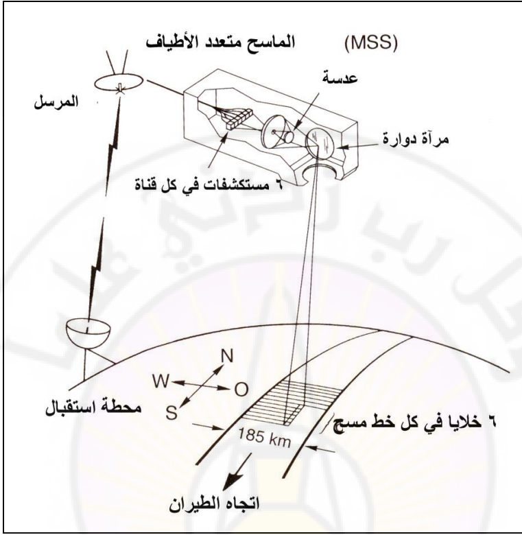
شكل (64): آلية المسح في الماسح متعدد الأطياف
