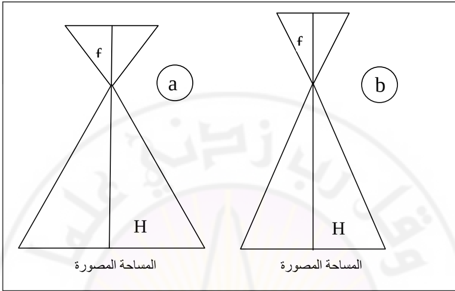
شكل (41): علاقة ارتفاع الطيران بمقياس الصورة إذا تغير البعد المحرق
