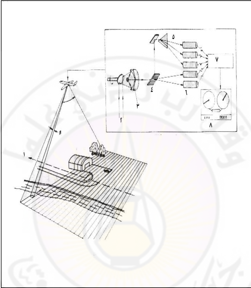
شكل (63): مكونات الماسح متعدد الأطياف
