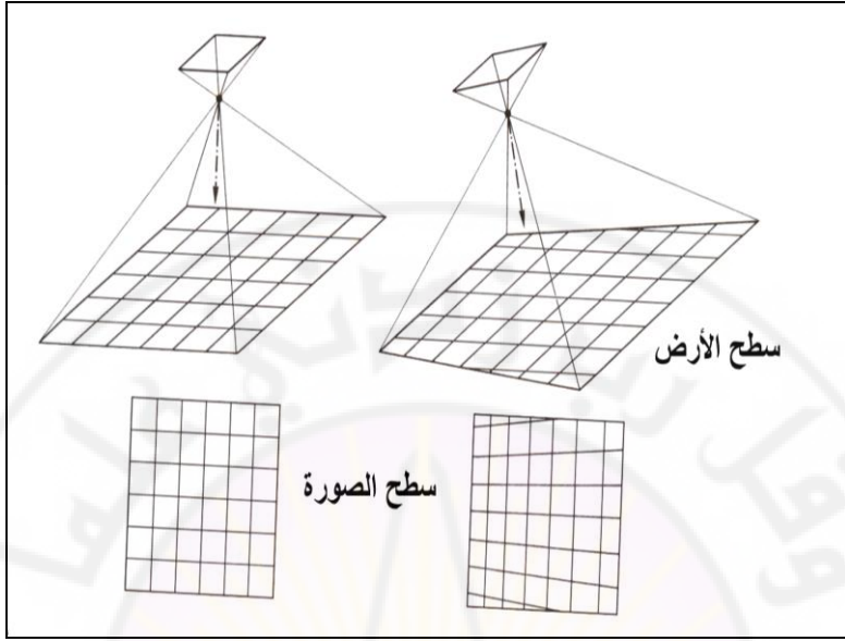
شكل (47): الإزاحة الميكانية وشكل شبكة الإحداثيات في حال التصوير العمودي والتصوير المائل
