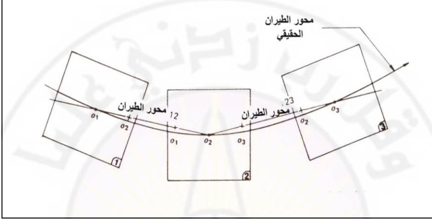
شكل (58): كيفية تحديد محور خط الطيران لأزواج مجسمة من الصور المتتالية على طول خط الطيران
