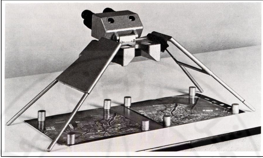
شكل (56): ستيريو سكوب ذو مرآيا يسمح بالتكبير 6 مرات
