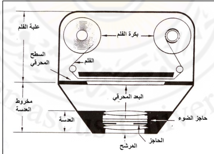
شكل (27): الأجزاء الرئيسة لآلة التصوير
