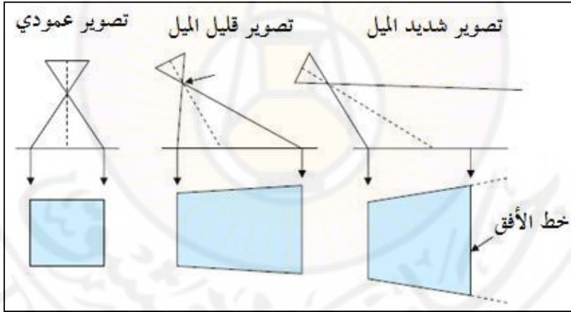
شكل (46): الإزاحة الميالية وشكل المساحة المصورة في التصوير العمودي والمائل
