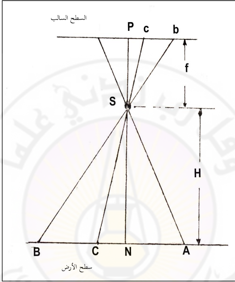
شكل (39): حساب مقياس صورة عمودية على أرض منبسطة
