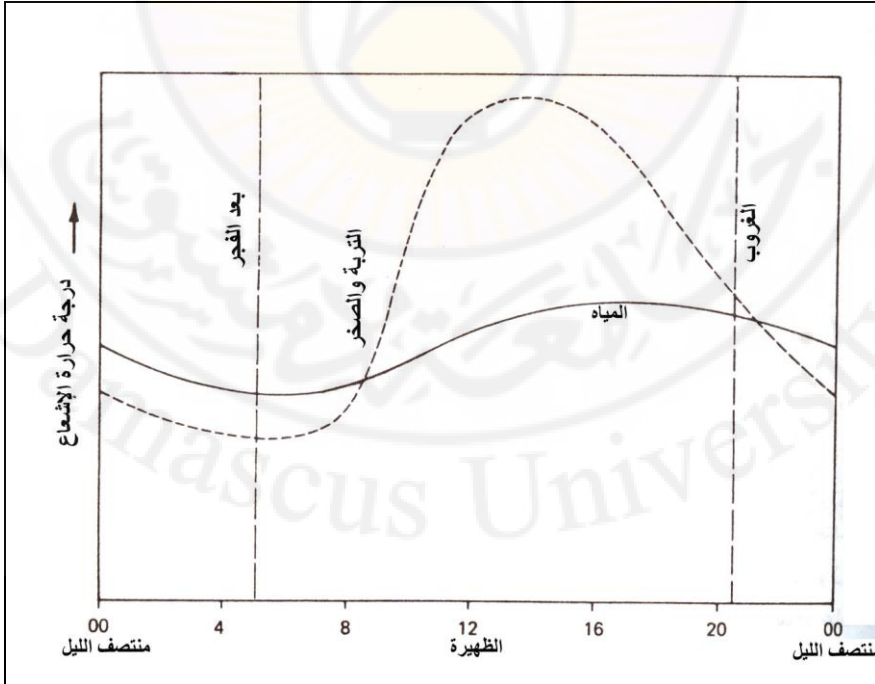
شكل (69) التغيرات اليومية لدرجات حرارة الإشعاع للتربة والصخور والمياه خلال 24 ساعة
