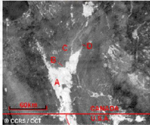
شكل (122): صورة لفيضان كندا عام 1997 في المجال تحت الأحمر الحراري
