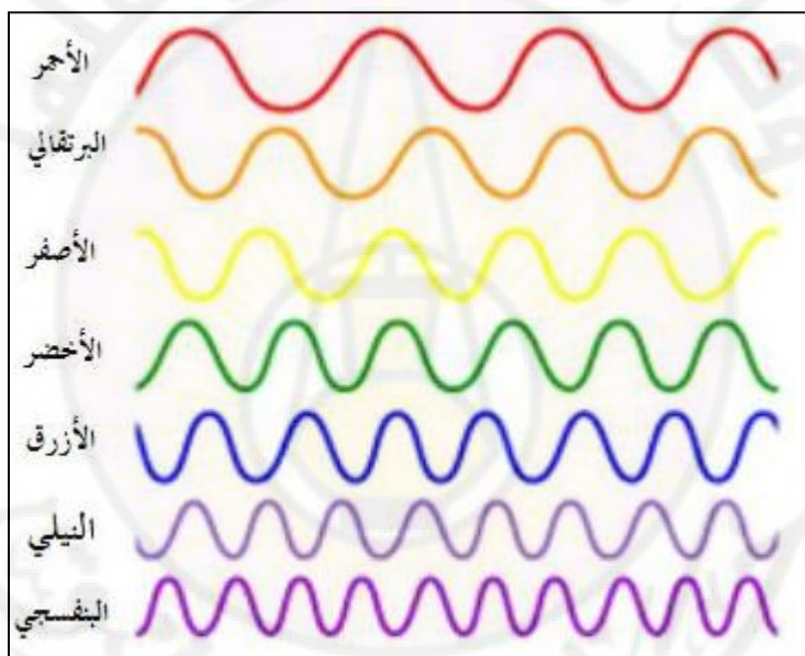
شكل (9): اختلاف أطوال موجات الألوان في المجال المرئي
