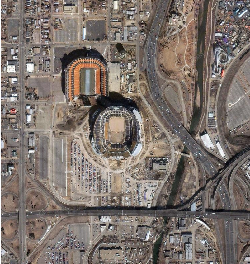
شكل (104): صورة ملتقطة من القمر IKONOS-2 للستاد الرياضي الجديد في مدينة دينفر في الولايات المتحدة الأمريكية بتاريخ 2001/8/19 بقدرة تمييز مكانية 1 متراً
