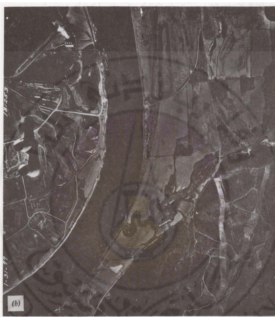
شكل (49): صورة ماثلة للموقع السابق نفسه ولكن الانزياح التضاريسي واضح في هذه الصورة بسبب ابتعاد البرجين عن النقطة الرئيسية
