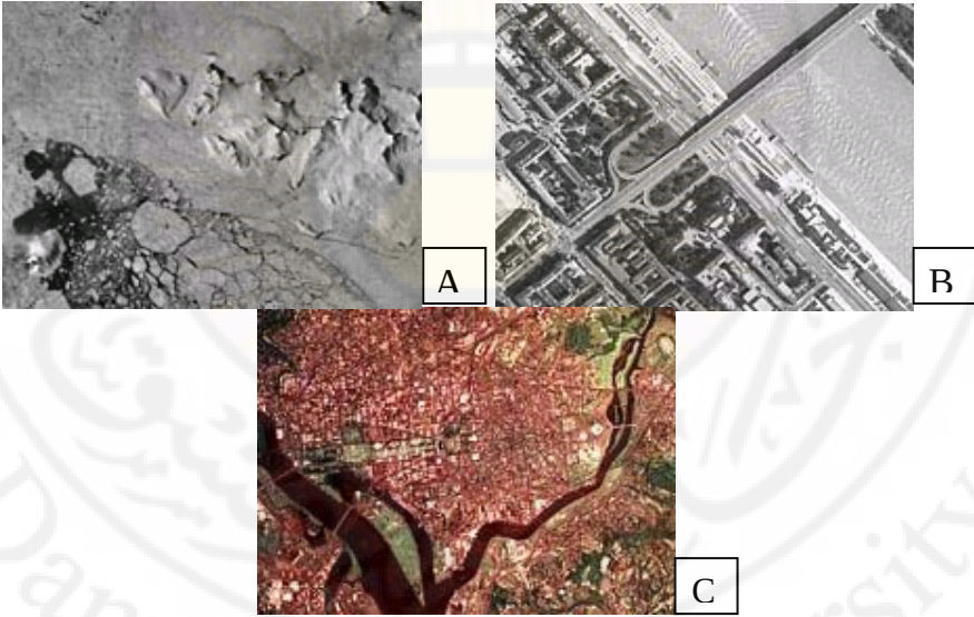
شكل (119): صور ملتقطة بآلات تصوير روسية مختلفة
