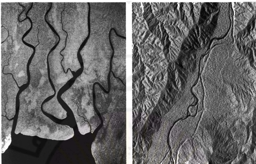
شكل (74): تأثير خشونة السطح وأشكال سطح الأرض في مرئيات الرادار
