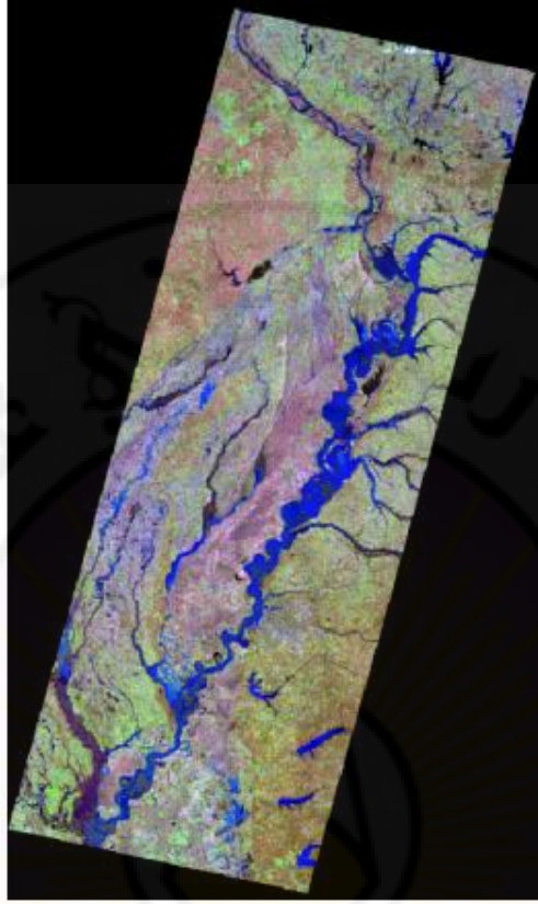
شكل (124): موزاييك لثلاث صور ملتقطة بالقمر الصناعي لاندسات لفيضان الميسيسيبي 1997م
