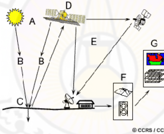
شكل (6): أسس عملية الاستشعار عن بعد: A مصدر الطاقة، B الممر الإشعاعي، C الظاهرة، D المشعرات، E المحطات الأرضية، F تفسير الصور، G التطبيقات
