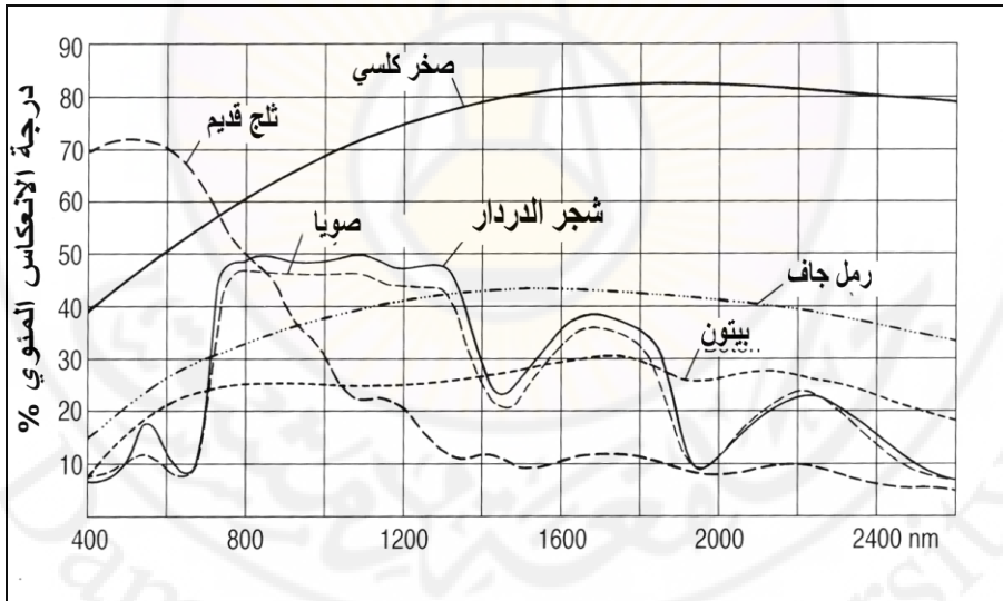
شكل (12): درجة الانعكاس لبعض الأرض: الأرضية
