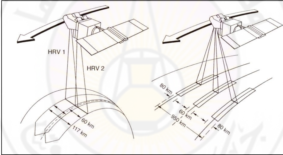
شكل (94): طريقة التقاط الصور بواسطة القمر سبوت.
