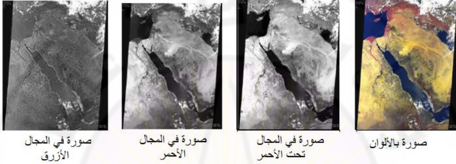
شكل (5): مثال عن صور مأخوذة بمجالات طيفية عدة للمنطقة نفسها من الوطن لعربي
