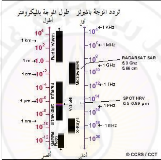
شكل (8): أنواع الموجات الكهرومغناطيسية وأطوالها
