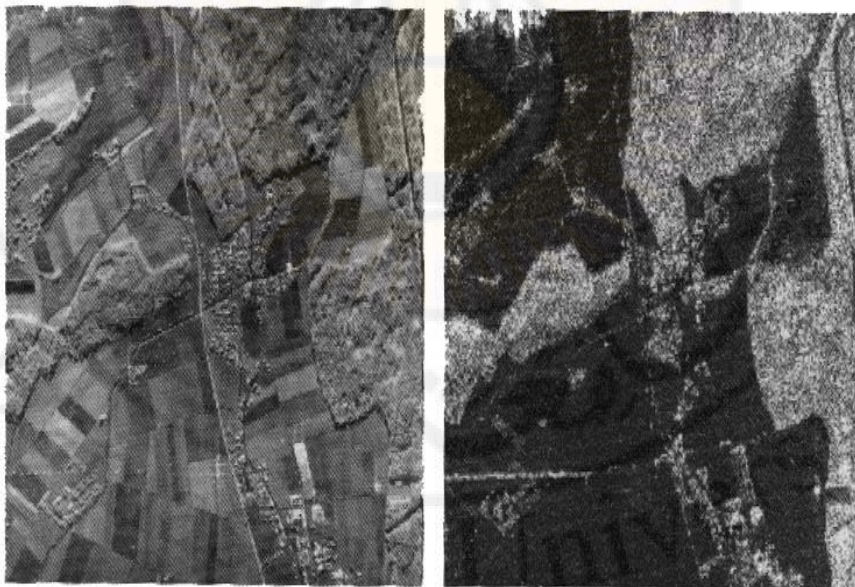
شكل (75): صورتان من SAR للمكان نفسه ملتقطتان في أطوال موجية مختلفة: الصورة اليسرى ملتقطة بموجة قصيرة في المجال X بطول 9.55 GHz، والصورة اليمنى بموجة طويلة في المجال B بطول 0.415 GHz بمقياس 35000/1.
