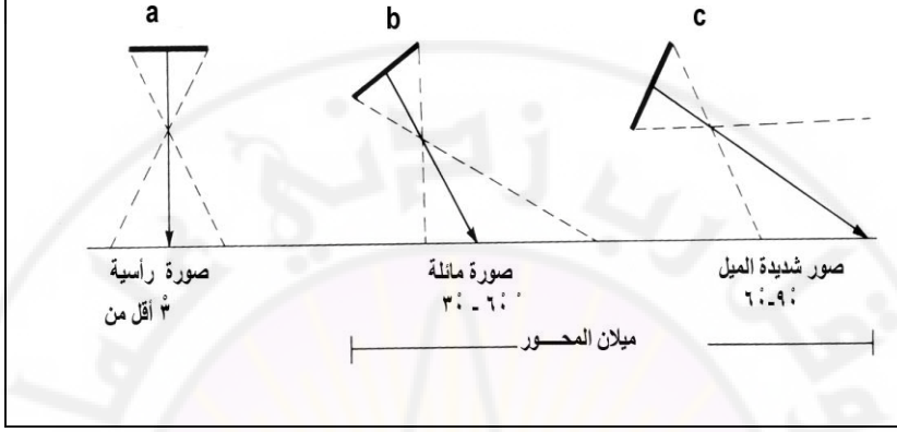
شكل (30): تصنيف الصور حسب ميلان محور العدسة
