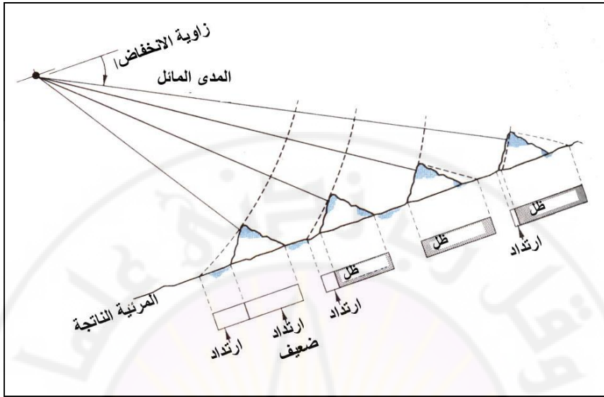
شكل (73) تأثير تضاريس سطح الأرض في الإزاحة في مرئيات SLAR
