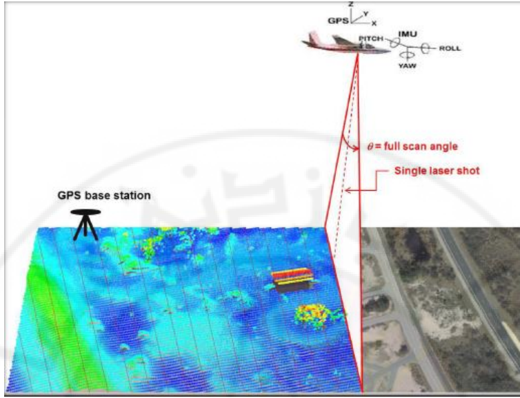
شكل (127) رسم تخطيطي لنتائج مسح الليدار المحمول جواً نتج عنه خطوط متوازية من النقاط المقاسة (توجد أنماط مسح ضوئي أخرى لكن هذا النوع من المسح هو الأكثر شيوعاً)
