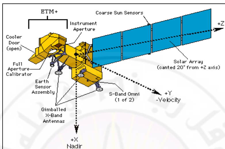
شكل (89): القمر الصناعي لاندسات-7 والمواسح التي يحملها
