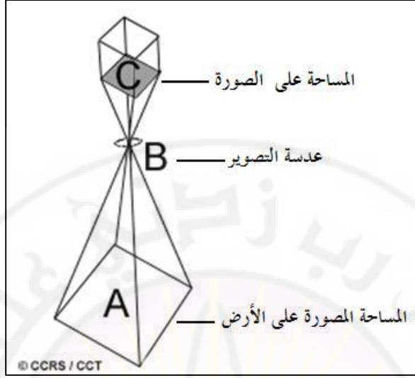
شكل (38): مقياس الصورة الجوية
