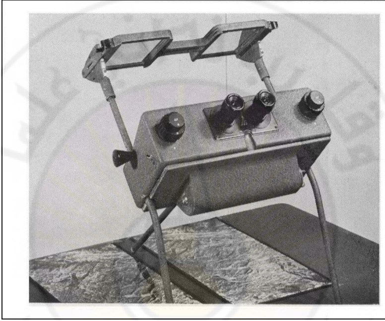
شكل (60): منظار مجسم ماسح ذو مرآيا من هولندا (عن Schneider, 1974)
