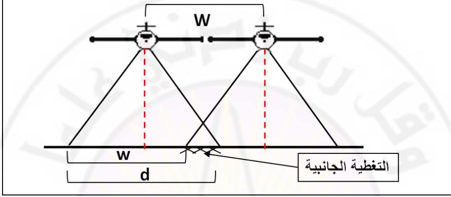
شكل (37): كيفية حساب التغطية الجانبية
