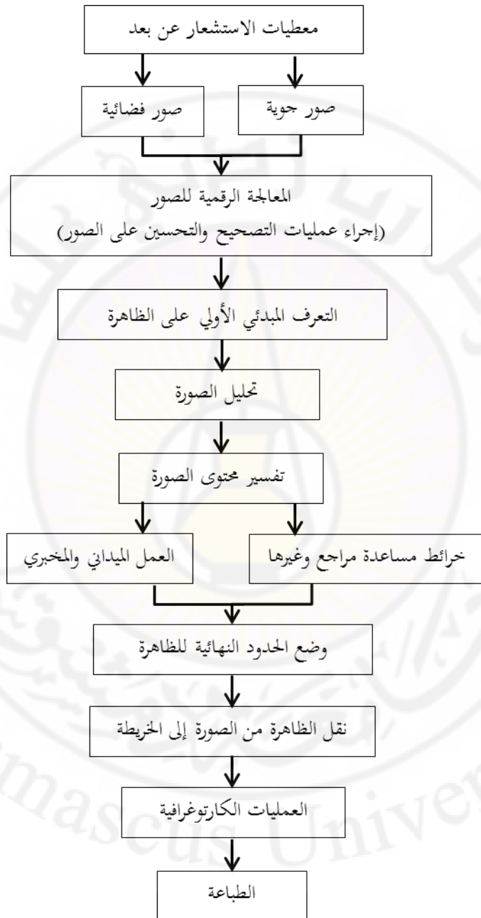
شكل (125): مخطط مراحل وضع الخرائط بواسطة معطيات الاستشعار عن بعد
