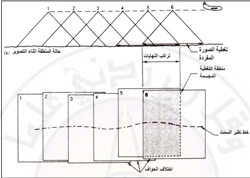
شكل (34): تراكب الصور على طول خط الطيران
