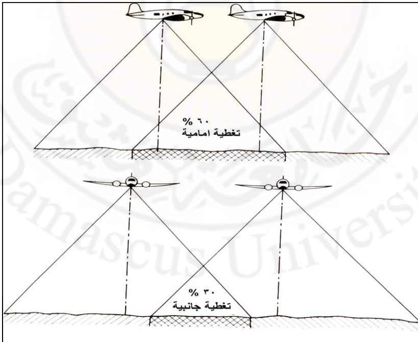
شكل (35): التغطية الأمامية والجانبية في الصور المتلاحقة (عن Schneider 1974)
