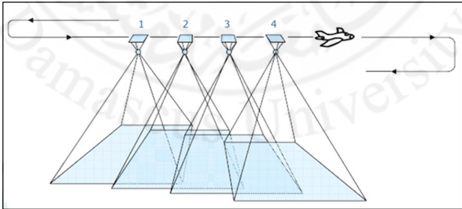
شكل (33): التقاط الصور بشكل متتابع على خط الطيران
