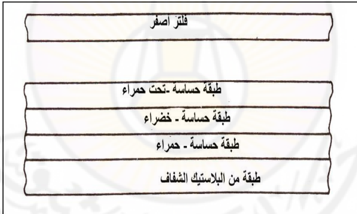
شكل (24): مقطع عرضي في فيلم ملون بألوان تحت حمراء
