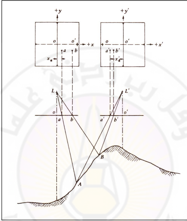
شكل (57): التجسيم الناتج عن اختلاف موقع النظر (عن Lillesand . Kiffer 1987)
