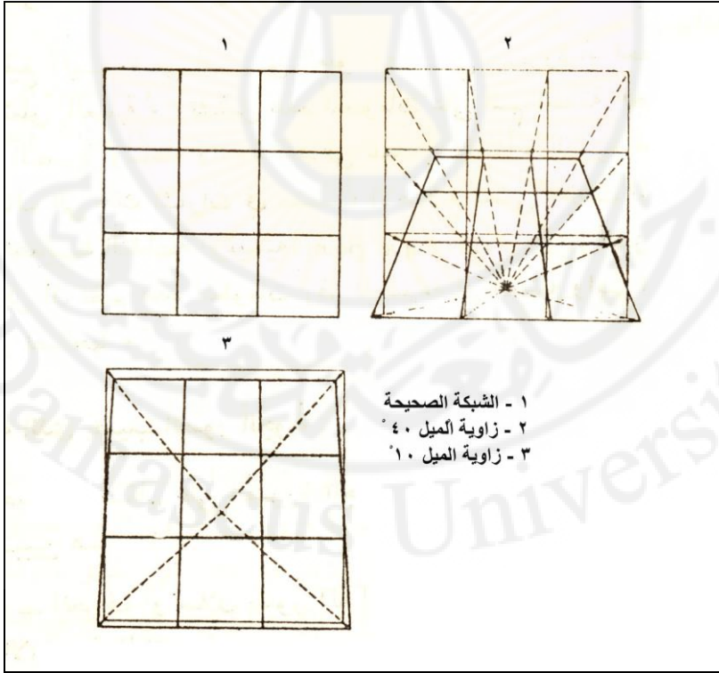
شكل (45): الإزاحة الميلاية في الصور الجوية حسب زاوية النظر
