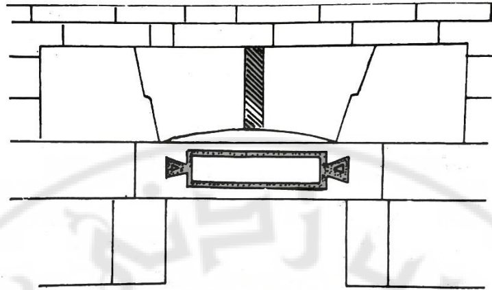
سكف مع قوس عاتق
