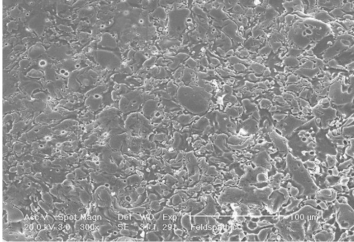
الشكل (1): صورة بالمجهر الإلكتروني الماسح للخزف الزجاجي الفلدسباري (McLaren and Cao 2009)
