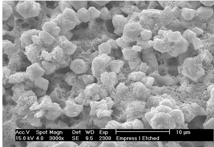
الشكل (2): صورة بالمجهر الالكتروني الماسح للخزف الزجاجي المقوى باللوسايت McLaren and Cao 2009
