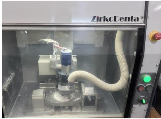
الشكل (16): جهاز النحت الخاص بنظام Zircodenta
