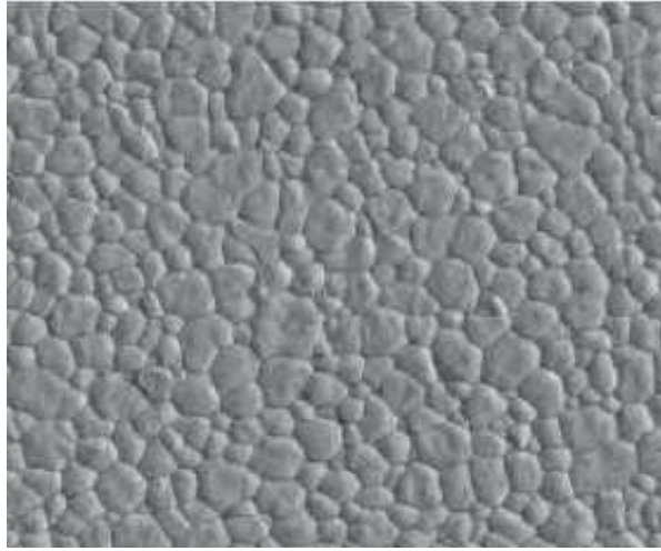
الشكل (4): صورة بالمجهر الإلكتروني الماسح للزركونيا المكثفة كلياً McLaren and Cao 2009
