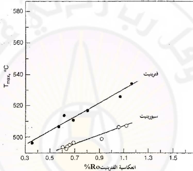
الشكل (10-10). التغيرات في قيم T_{max} مع ازدياد النضج كتابع لنوع المستخلص (Dembicki et al. 1983)
