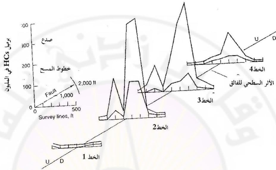
الشكل (3-5). بروفيل جيوكيميائي سطحي عبر فالق كبير في منطقة منتجة للنفط في شمال شرق تكساس. حيث يمثل المنحني العلوي الغاز الكلي، ويمثل المنحني السفلي مرافقات الميثان، وتمثل الخطوط المستقيمة مكان أخذ العينة
