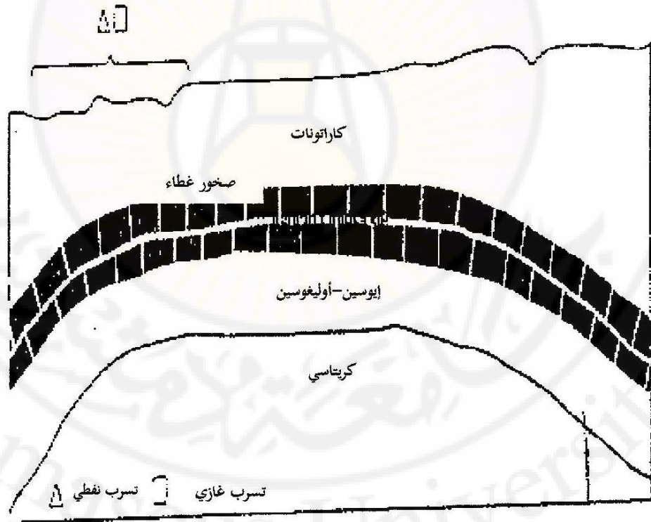
الشكل (5-1). تسرب النفط والغاز عبر الصخور الكلسية المشققة في تشكيلة أسمري في حقل مسجد سليمان في إيران.
