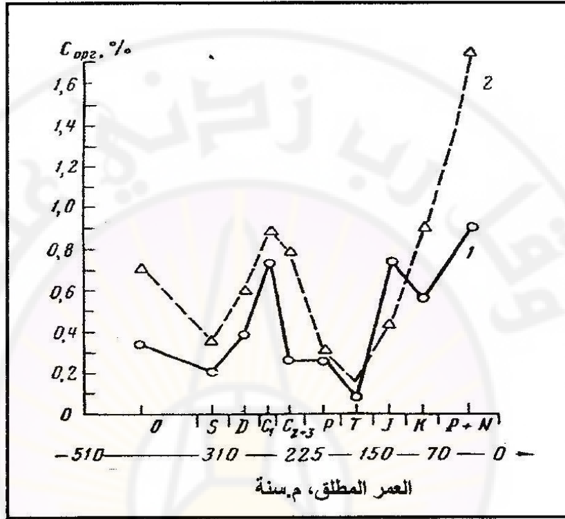
الشكل ( 1 - 2 ) محتوى الكربون العضوي في الصخور الرسوبية، ذات الأعمار المختلفة. 1- البلاتفورا الروسية . 2 - أمريكا الشمالية. (عن كارتسوف) .
