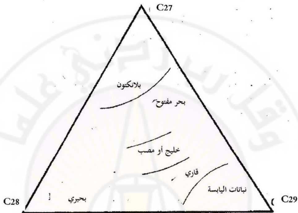
الشكل (8-9). مخطط ثلاثي لتفسير التوزع المنشئي للسيرانات
