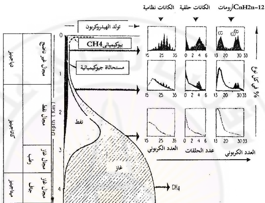
الشكل (3-4) مخطط عام لتولد المواد الهيدروكربونية الناتج عن ازدياد عمق طمر الصخور.
