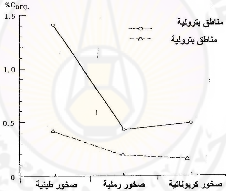
الشكل ( 3-20 ) المعدل الوسطي للكربون العضوي في كل من الصخور الطينية، والرملية، والكربوناطية.
