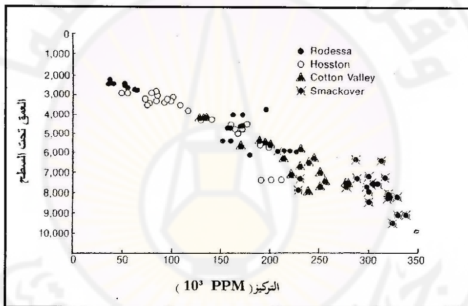
الشكل (3-7). ازدياد ملوحة المياه مع ازدياد عمق الطمر.
