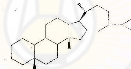
الشكل (32-3). بنية الديستيران (Disterane).
