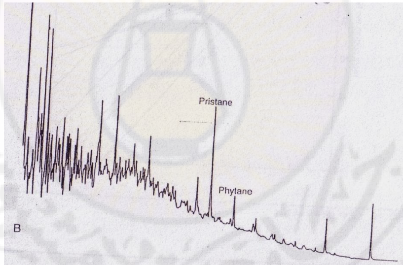
الشكل (2-9). كروماتوغرام غازي من C12-C27، نلاحظ من خلاله خسارة جزئية للبارفينات النظامية في أ، وخسارة كاملة تقريباً لهذه البارفينات في ب.
