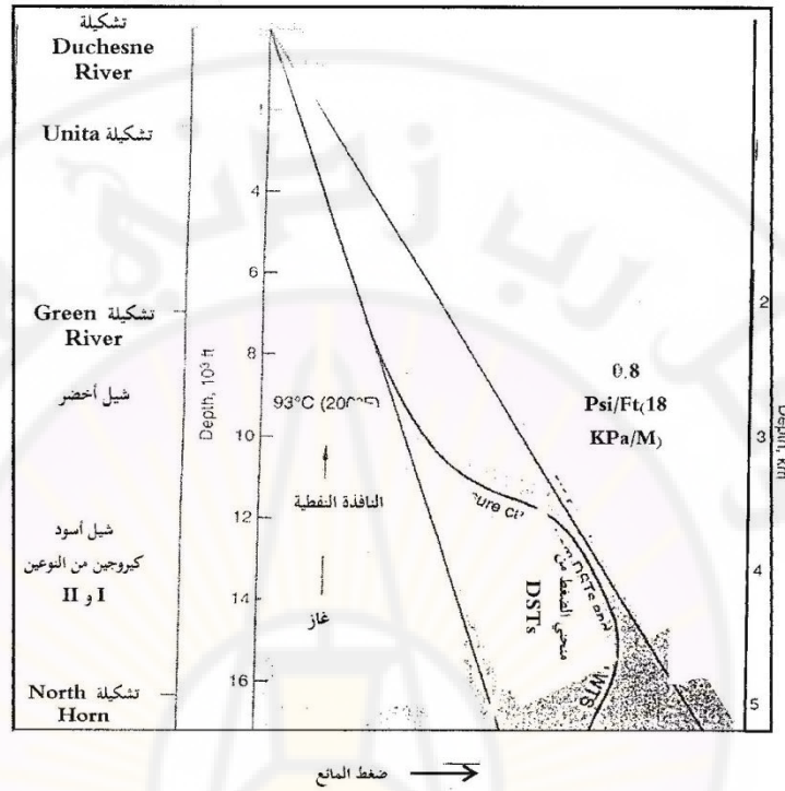
الشكل (8-6). العلاقة بين تولد المواد الهيدروكربونية وضغط الموائع في البئر 1-11B4 Brevorson في حقل Greater Altamont في حوض Uinta في Utah
