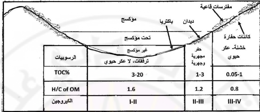
الشكل (3-3) تأثير البيئات المائية القاعية البحرية، والبحيرية، ومحتوى الأكسجين على محتوى الكربون
