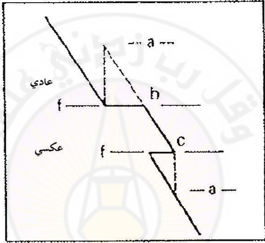
الشكل (4-15). وجود مجال عمقي فيه قيم SCI أعلى من القيم المقترضة.
