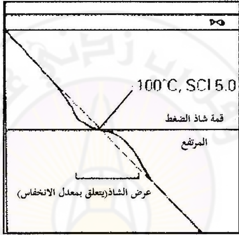
الشكل (4-16). حالة تناقص في تدرج قيم SCI قبل مستوى معين، ثم تزايد بعده، ليشكل الخط منحنين متعاكسي الاتجاه قبل أن يأخذ استقامة من جديد.
