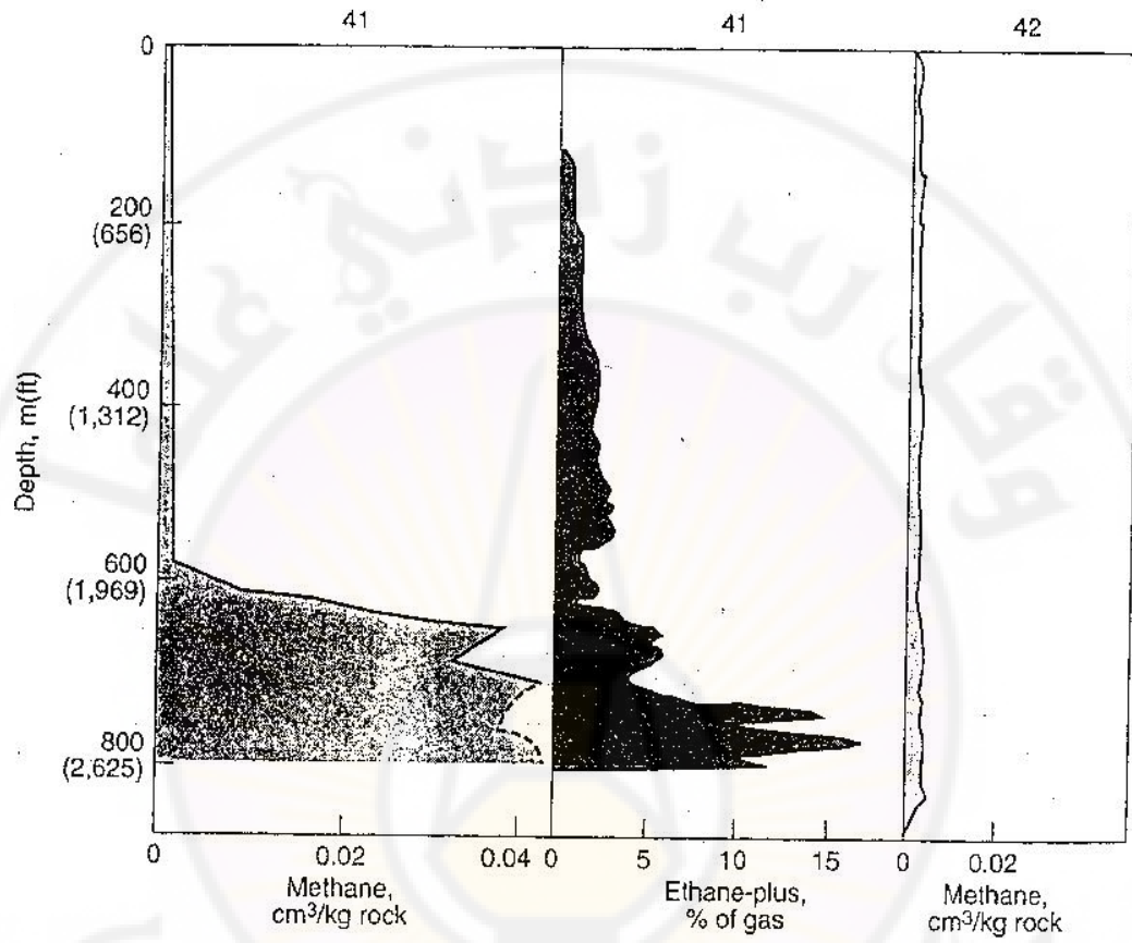
الشكل (10-1). سجلات الغاز في طين الحفر في البترين 41 و 42 في منطقة Kum-Dag في روسيا) (Yasenev, 1962)
