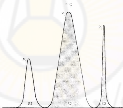
الشكل (4-6). البيكات الثلاثة الناتجة عن التكسير الحراري للصخر.
