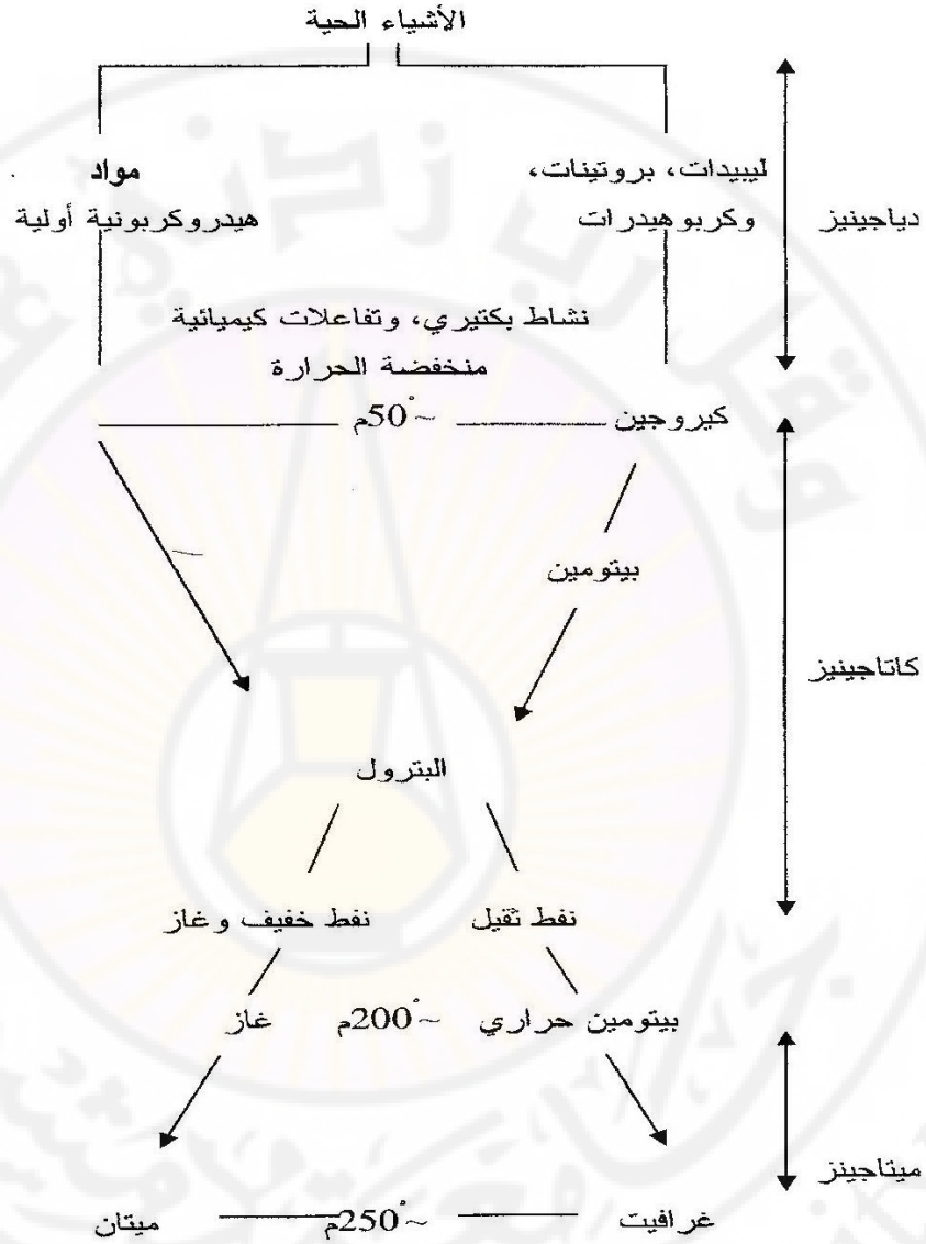
الشكل (4-1). نشأة البترول ونضجه اعتباراً من الكائنات الحية.
