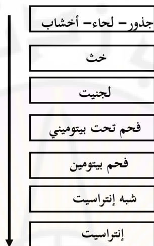
الشكل ( 3-23 ) مخطط سلسلة الفحوم الهيومية حتى الانتراسيت .
