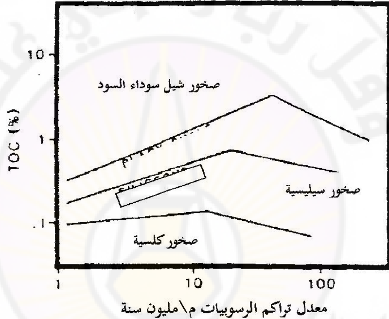
الشكل (3-14) العلاقة بين قيم الكربون العضوي الكلي، ومعدل تراكم الرسوبيات، وتأثره عند معدلات الترسيب العالية جداً بعامل التخفيف.
