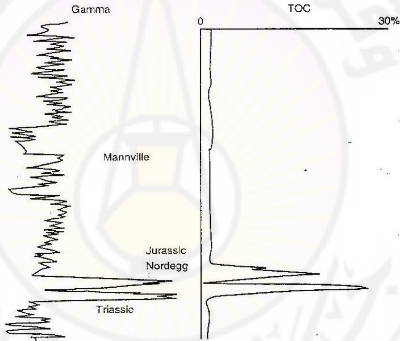
الشكل (3-10). مقارنة بين نسب الكربون العضوي وقياسات أشعة غاما في صخور الشيل في تشكيلة نورديج الجوراسية والتشكيلات المجاورة (Creaney and Allan, 1990)
