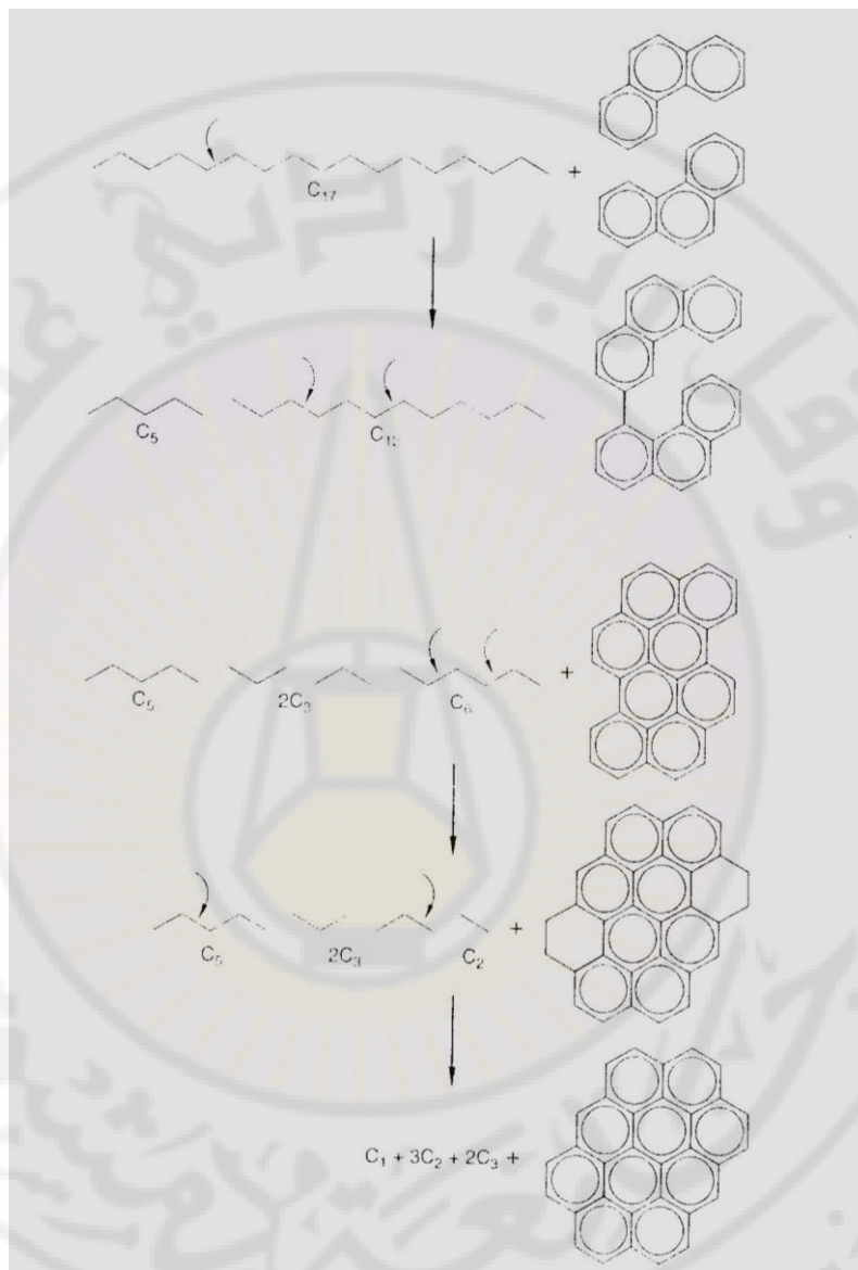
الشكل (3-9). تشكل المواد الهيدروكربونية الغازية، و البيروبيتومين، أو الغرافيت المتبقي أثناء التفكك الحراري للبترو في الخزان.
