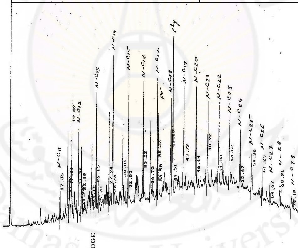
الشكل (2-3) زمخطط ناتج عن التحليل في الكروماتوغراف الغازي (كروماتوغرام)
