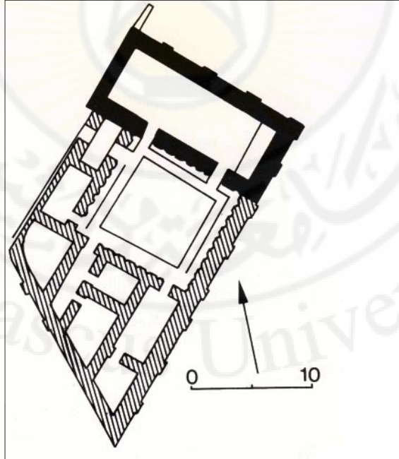
الشكل ٤٣: معبد نينر في ماري، عن: (Margueron, J.-C. 2003, fig. 205a).
