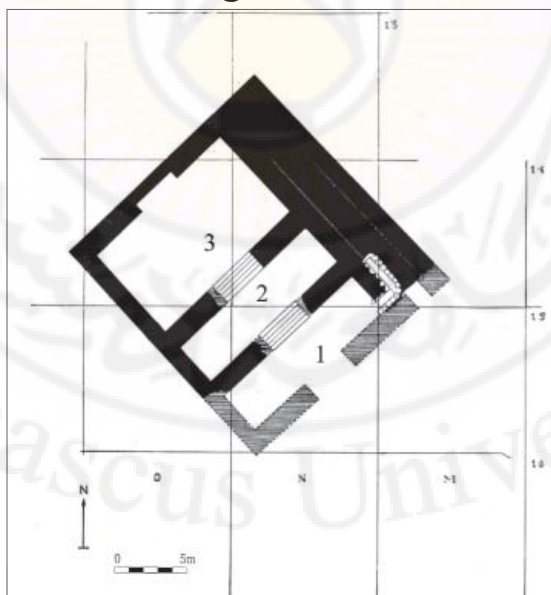
الشكل ٧١: معبد آلالاخ السوية ٤، عن: (Woolley, L. 1955, fig. 30).
