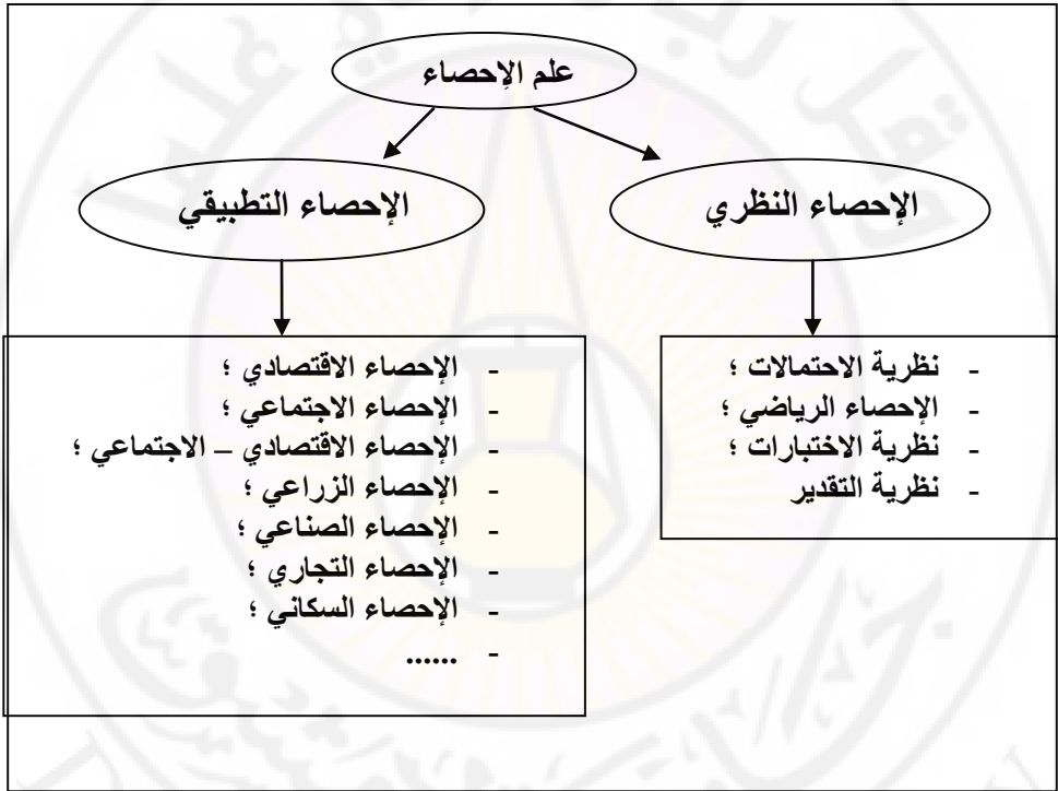
الشكل رقم (1-1) : الفروع العلمية لعلم الإحصاء وما يتفرع عنها
