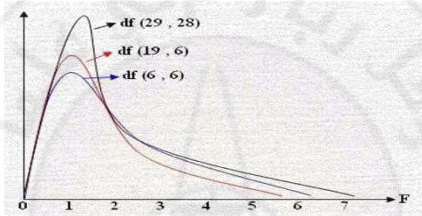
شكل (3-1): الشكل البياني لتوزيع (F).
