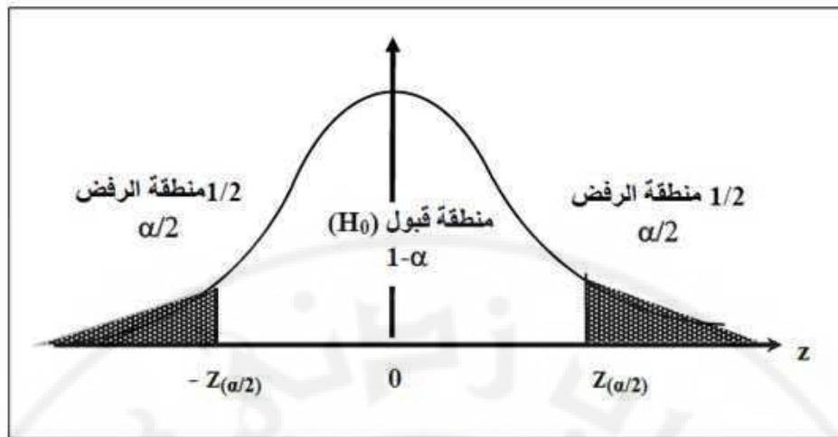
شكل (2-10): التمثيل البياني لاختبار الفروض للفرق بين متوسطي مجتمعين تباينهما معلوم.
