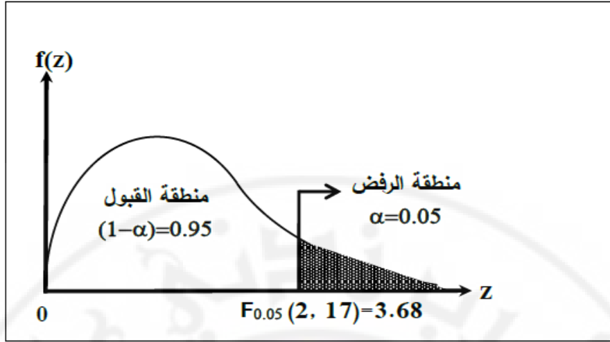
شكل (3-3): التمثيل البياني لمنطقتي القبول والرفض للمثال (3-3).
