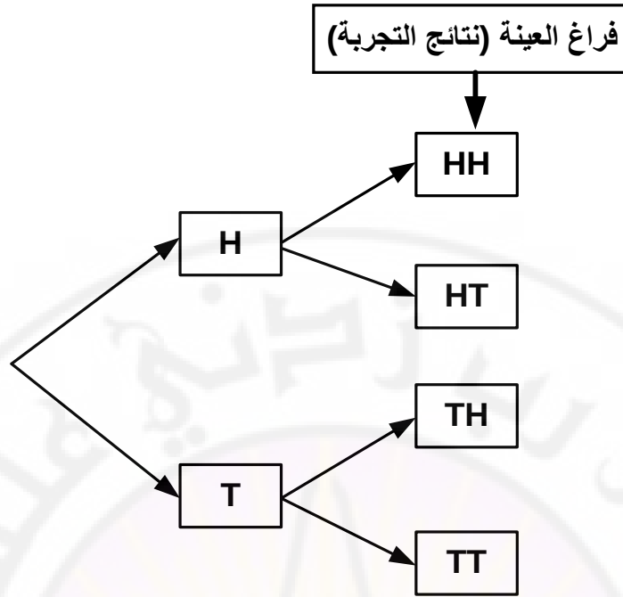
شكل (1-1): الرسم الشجري لتجربة إلقاء قطعة النّود مرتين.
