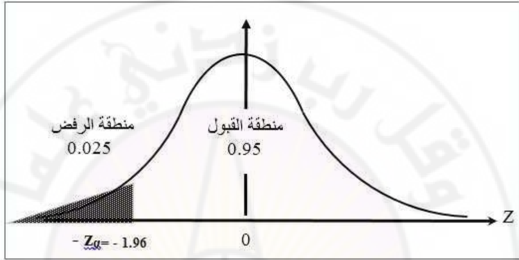
شكل (2-12): التمثيل البياني لمنطقتي القبول والرفض للمثال (7-2).
