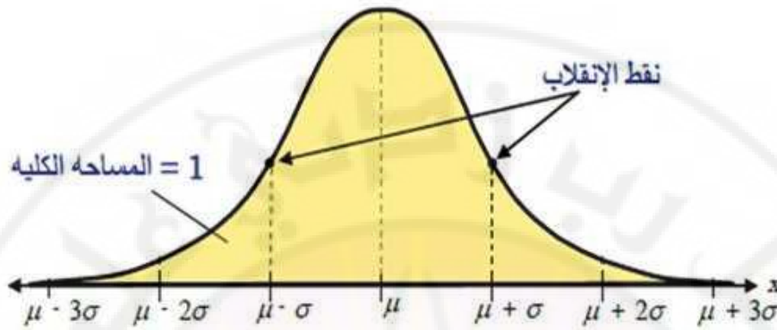
شكل (12-1): التمثيل البياني للتوزيع الطبيعي.
