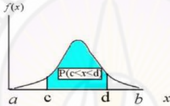
شكل (10-1): التمثيل البياني لحساب احتمال المتغير يقع c \leq X \leq d .
