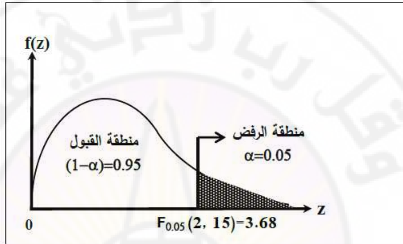
شكل (6-3): التمثيل البياني لمنطقتي القبول والرفض للمثال (5-3).
