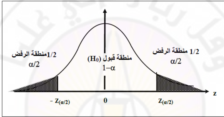
شكل (19-2): التمثيل البياني لاختبار الفروض للفرق بين نسبتي مجتمعين.
