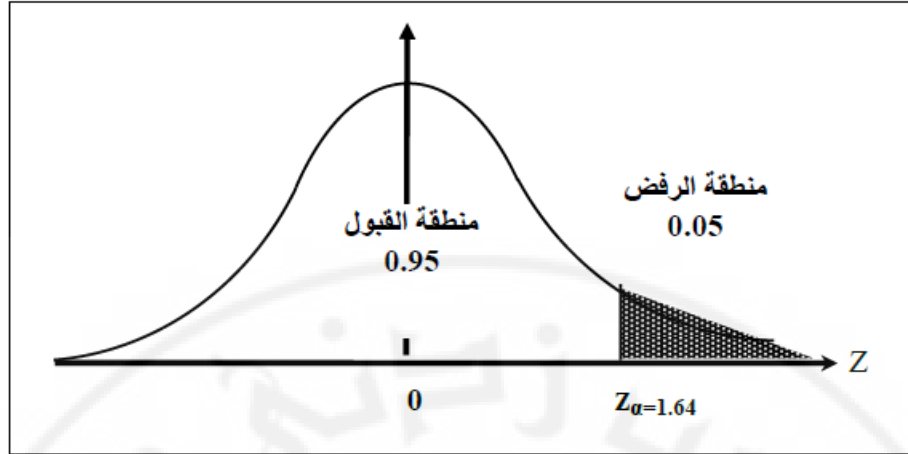
شكل (8-2): التمثيل البياني لمنطقتي القبول والرفض للمثال (4-2).
