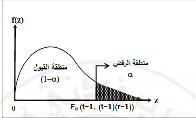
شكل (4-7): التمثيل البياني لمنطقتي القبول والرفض لاختبار F بتصميم (CRBD).
