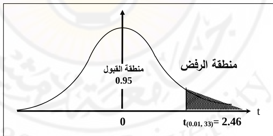
شكل (2-15): التمثيل البياني لمنطقتي القبول والرفض للمثال (2-9).
