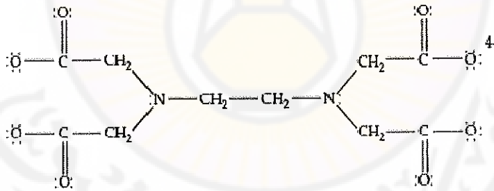
\text{EDTA}^{4-} , ethylenediaminetetraacetate ion
