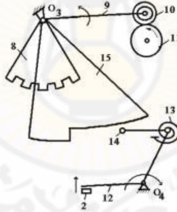
الشكل (17-1): آلية لمنع توقف الملف عند القطر المحدد للملف Imatex BA "
