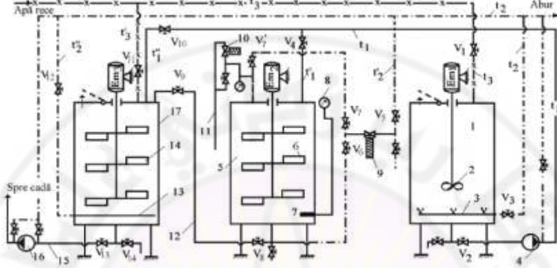
الشكل (9-3): محطة تحضير (مطحخ) البوش (Iacob, I., 2010)
