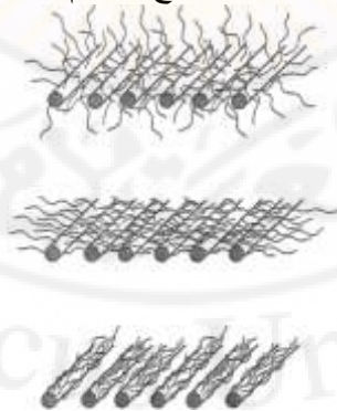
الشكل (3-13): التحكم بتشعر الخيوط بالتنبويز: الصورة في الأعلى: غير مُبوش، الصورة في الوسط: مبوش بشكل غير مناسب، الصورة في الأسفل: مبوش بشكل مناسب (Adanur, S., 2001).
