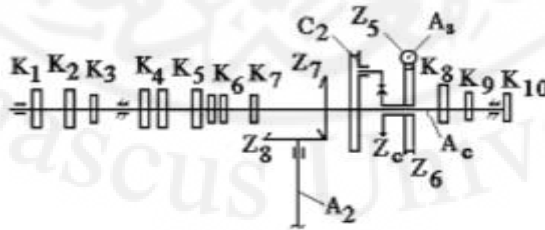
الشكل ( d-2-1 ): تحريك محور الكامات A_c ، A_2
