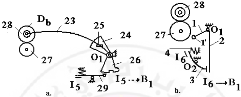
الشكل (4-1): آليات توقف الملف Imatex BA "
