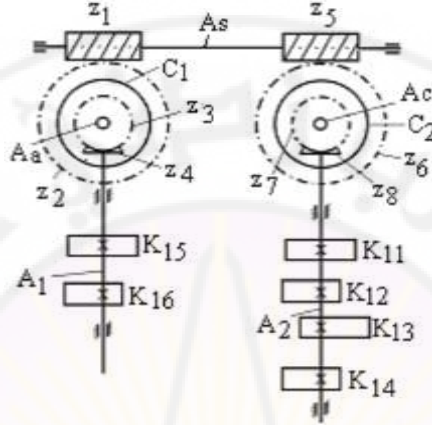
الشكل ( b-2-1 ): تشغيل أعمدة الكامات لآلة اللف Imatex BA
