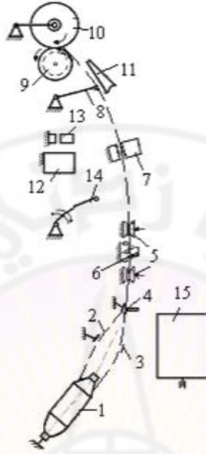
الشكل ( 1-1 ) : مخطط آلة اللف الأوتوماتيكية "IMATEX BA".
