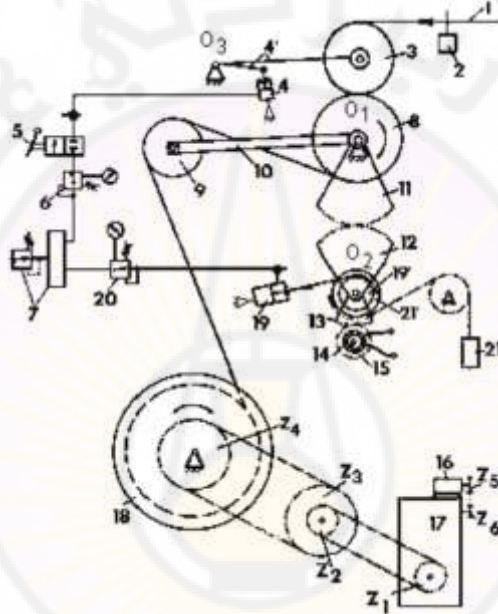
الشكل (3-8): آلية لف السداة بآلة التبويض
