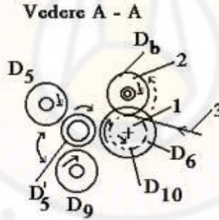
الشكل ( c-2-1 ): تفاصيل تحريك الكونة (لفائف)
