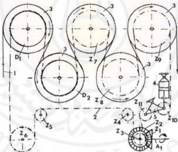
الشكل (6-3): آلية تشغيل اسطوانات التجفيف
