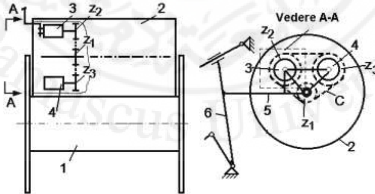
الشكل (7-2): عداد الطول لآلة التسدية "Elitex".
