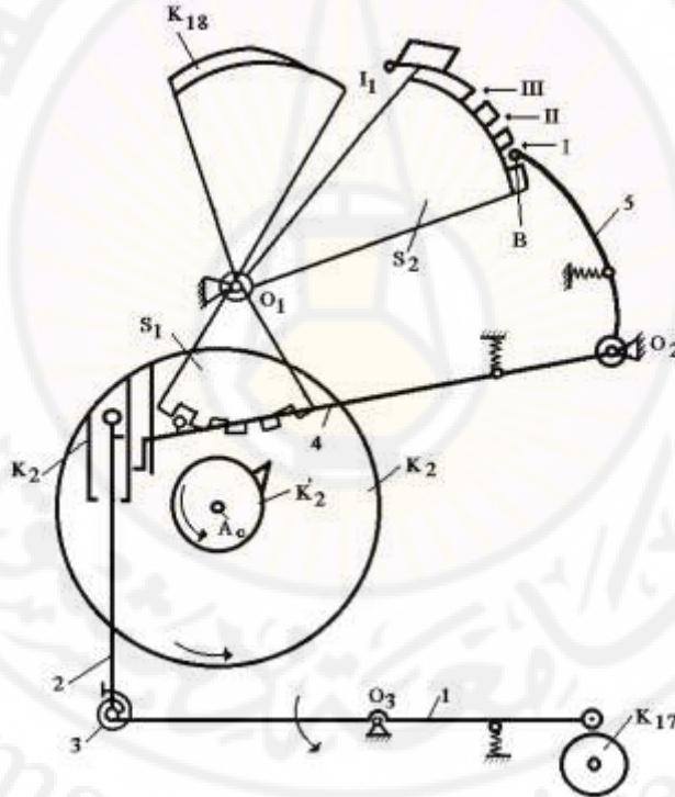
الشكل (7-1): آلية إيقاف التشغيل الأتوماتيكي بعد (2...4) دورات اقتران غير ناجحة Imatex BA
