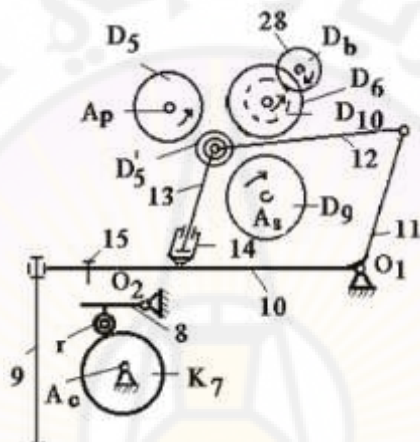
4-5-1- آلية دوران المخزن مع المواسير الاحتياطية
