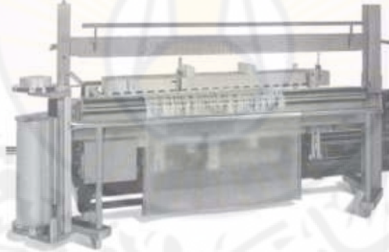
الشكل (4-4): آلة لحام خيوط السداء (Staubli) (Adanur, S.,2001). (Warp welding machine)
