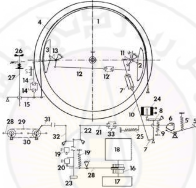
الشكل (2-17): آلية التشغيل والتوقف لآلة التسدية بالشرائط (الشقات) TEXTIMA
