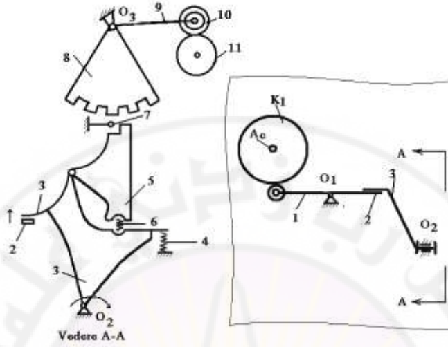
الشكل (16-1): آلية رفع وخفض الكونة (الملف) أثناء تشغيل الآلة Imatex BA "
