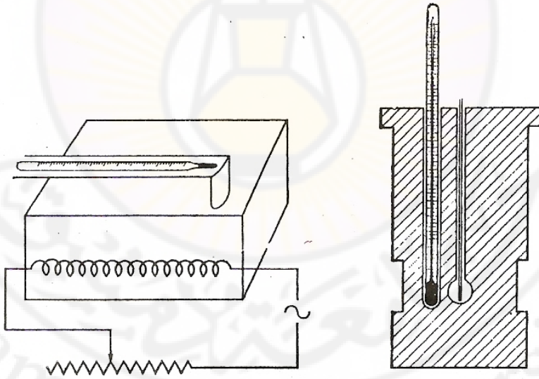
الشكل (3-10): الكتلة النحاسية المستعملة لتحديد درجة الانصهار
