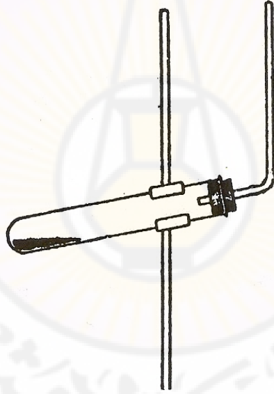
الشكل (2-3): جهاز الكشف عن الآزوت النشادري
