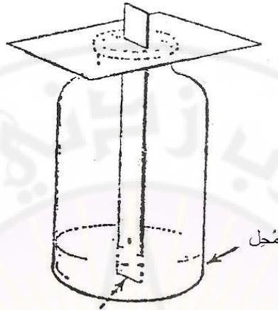
كروماتوغرام ورقي
