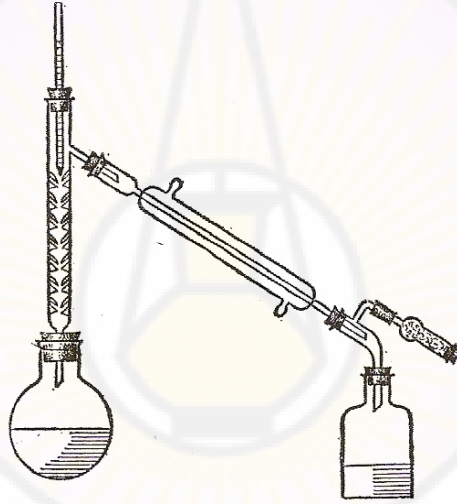
الشكل (1-11): جهاز لتقطير المحالّات المَجْفَفة
