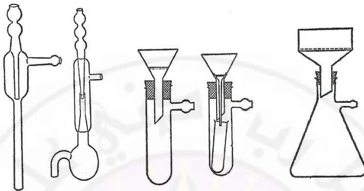
مُخلية مائية جهاز ترشيح تحت الخلاء جهاز ترشيح تحت الخلاء (ميكروني)
