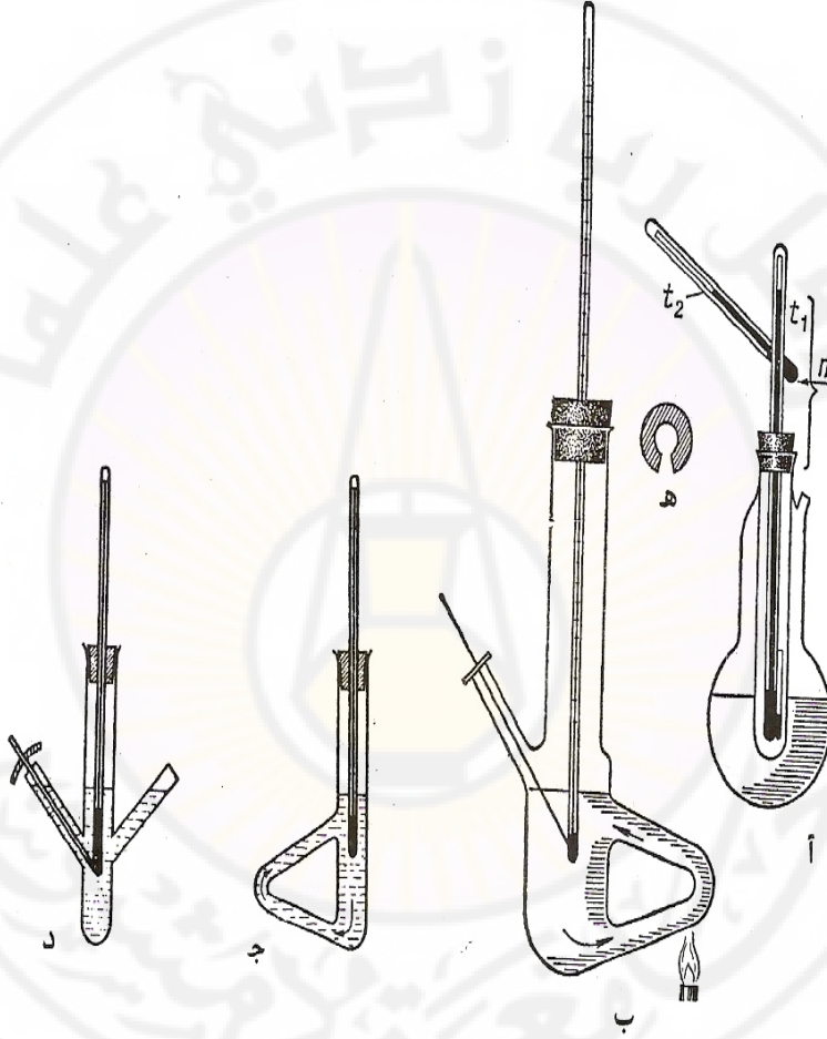
الشكل (2-10): الأجهزة المستخدمة لتحديد درجة الانصهار
