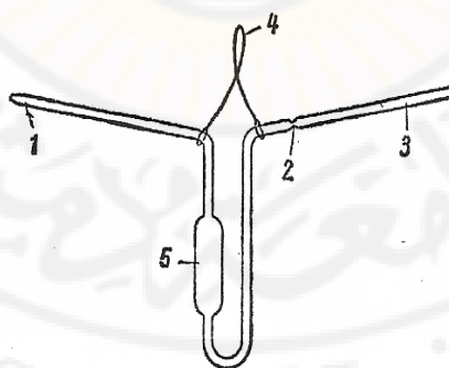
الشكل (5-10) نموذج البيكنومتر
