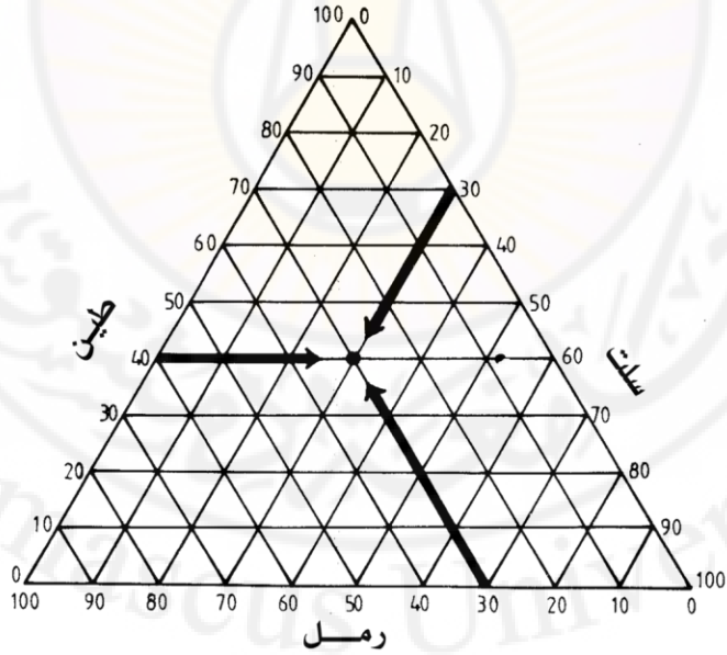
الشكل (٦ - ٧): مثلث القوام لتعيين قوام التربة.
