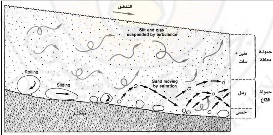
الشكل (٦ - ١٧): مقطع توضيحي يوضح تباين حجم المنقولات حسب العمق في مجرى نهر.
