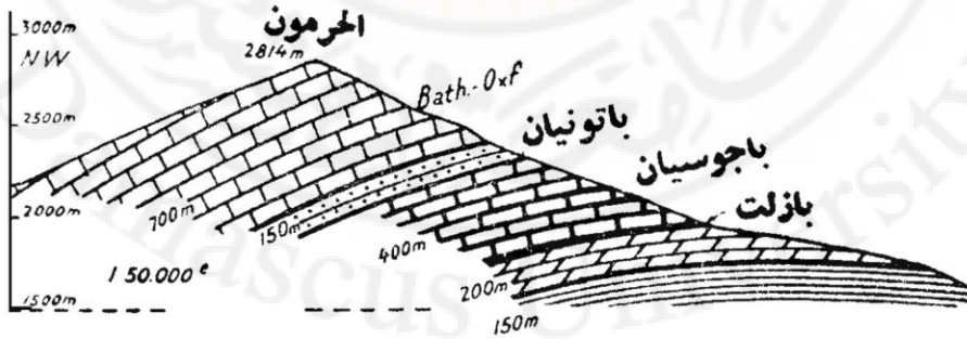
الشكل (٦ - ١٤): مقطع جيولوجي نموذجي للجوراسي في الحرمون.
