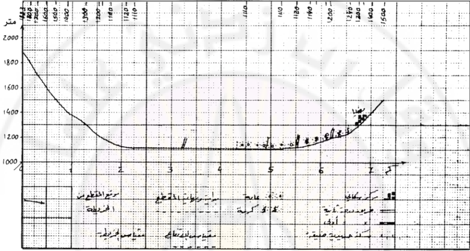
الشكل (٦-١٣): طريقة رسم المقطع الطبوغرافي
