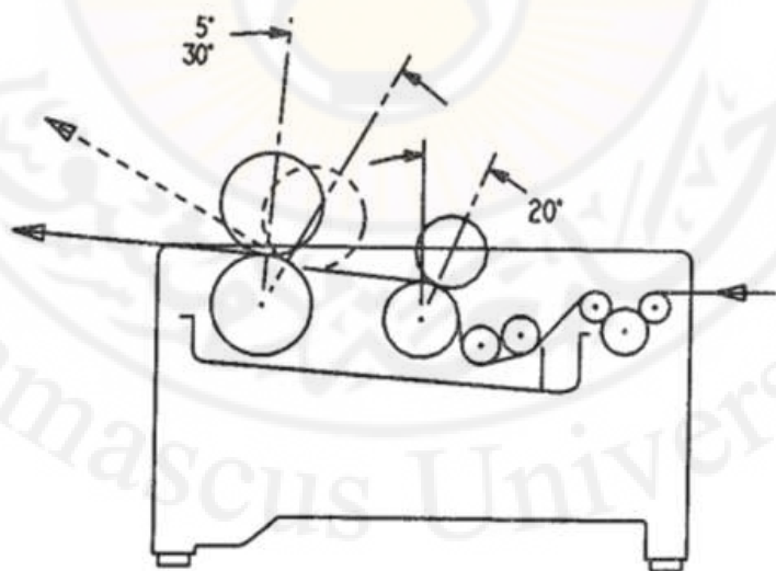
الشكل (4-4): الخروج الأمثل للسداء من اسطوانة العصر (Adanur, S., 2001)
