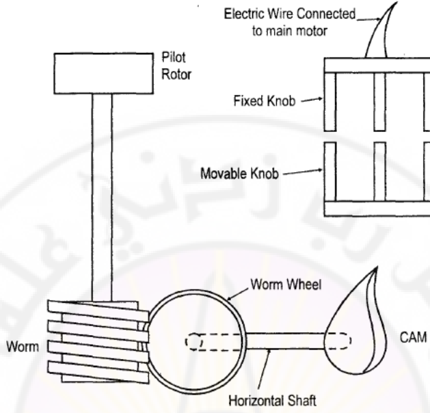
الشكل (2-24): طريقة تغيير سرعة سلندر اللف Method of changing winding of drum speed
