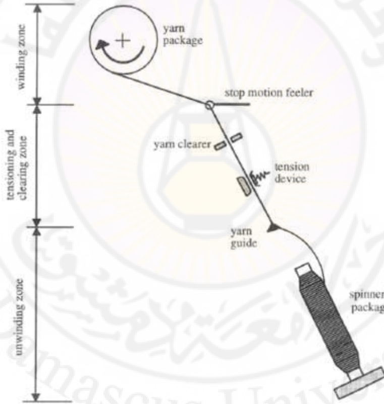
(الشكل 2-26): المخطط التكنولوجي لآلات التدوير (Adenor, S.,2001)
