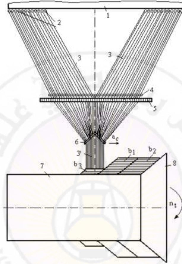
الشكل (3-9): التسدية غير المباشرة.
