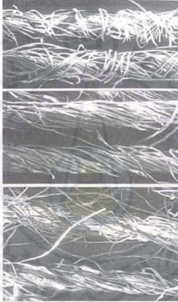
الشكل (4-39) : مقارنات بين غزول الطرف المفتوح open-end (العلوية) والغزول الحلقية ring spun (الوسطية) والغزول spun yarns بالنفث الهوائي.
