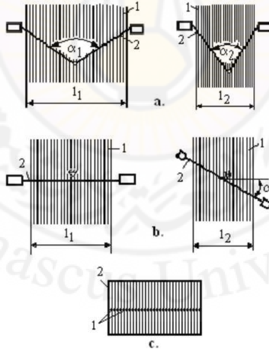
الشكل (3-11): مشط العرض Spata de lățime [47].
