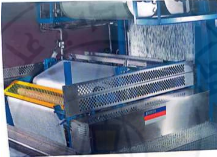
الشكل (4-56-أ) : آلية الترطيب في منطقة الغمر
