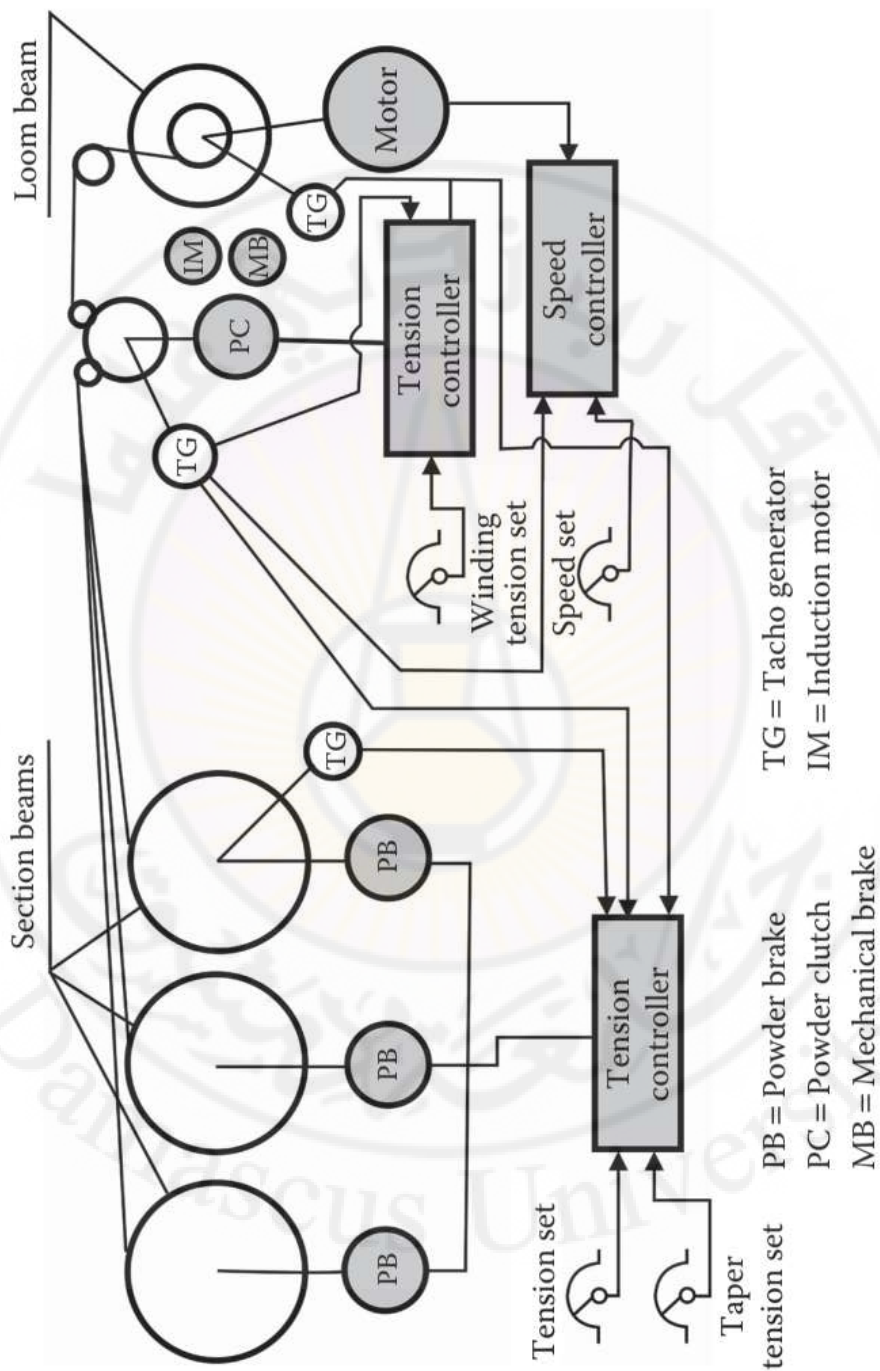
الشكل (4-65): التحكم التلقائي في الشد عند تنشيط الخيوط الفردية.
