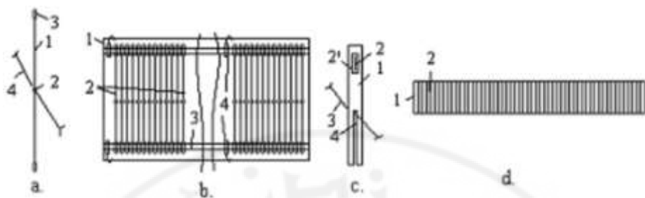
الشكل (3-5): العناصر البنائية للنير، الدرا وشفرات حساس السداء والمشط (Iacob, I., 2010)
