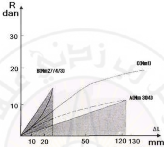
الشكل (7-1): العمل الميكانيكي للقطع
