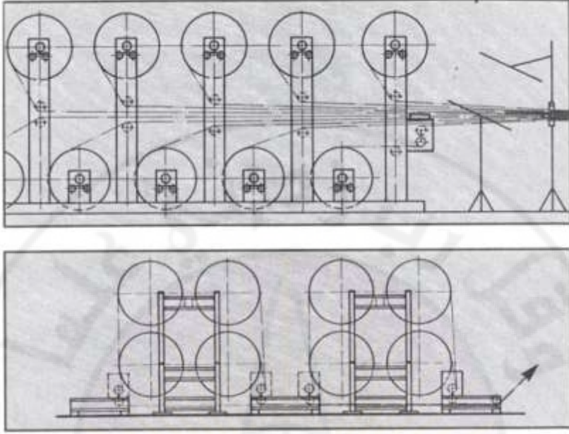
الشكل (4-5): ترتيبات المطاوي في النصبية. أعلى: نصبية متداخلة للخيوط المستمرة، أسفل: نصبية الغزل مع
