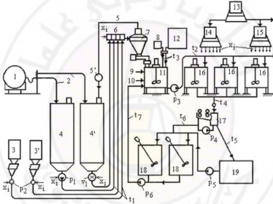
الشكل (4-43) : المنشأة التلقائية لتحضير البوش.
