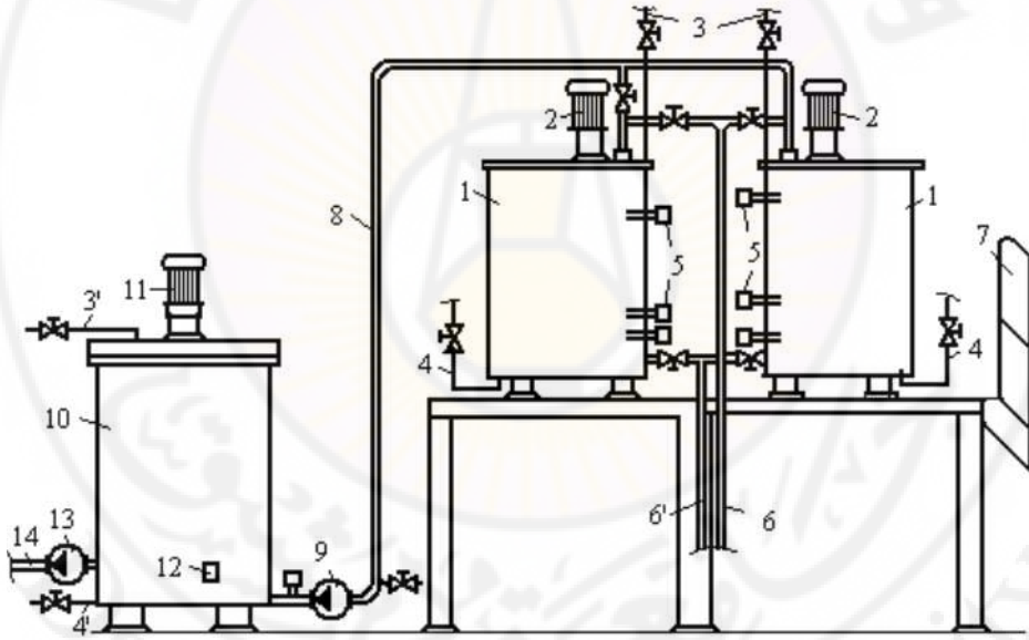
الشكل ( 4-41 ): تجهيزات التنشئة مع خزانات للخلط والتحضير والتخزين للبوش من نوع "Ben-Sizemix".
