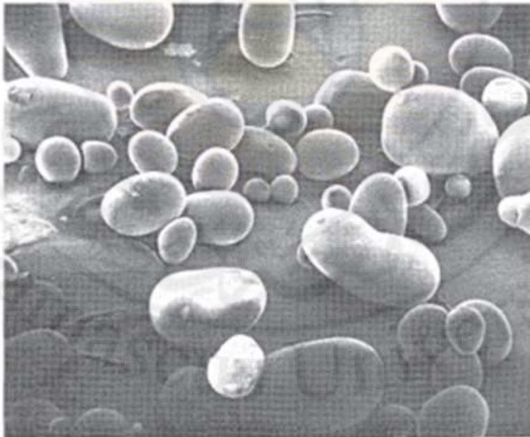
الشكل (4-32ب) : حبيبات نشاء الذرة (أعلى) وحبيبات نشا البطاطا Cornstarch granules (top) and potato starch granules
