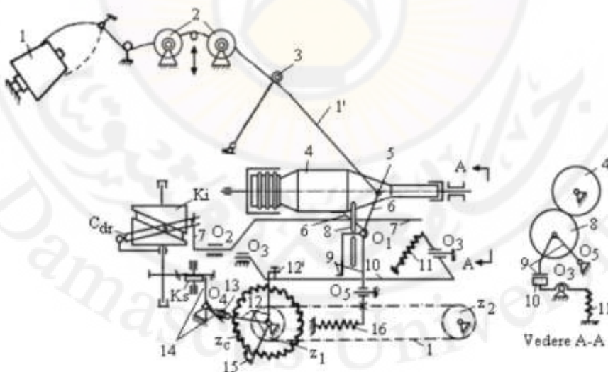
الشكل (2-8): مبدأ لف المواسير مع حامل. [47]
