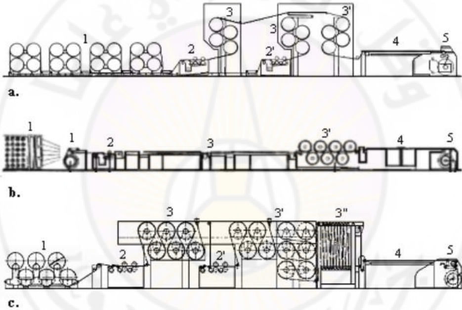
الشكل (4-10) : المبادئ التكنولوجية لآلات التبيوش (التنشئة) الحديثة
