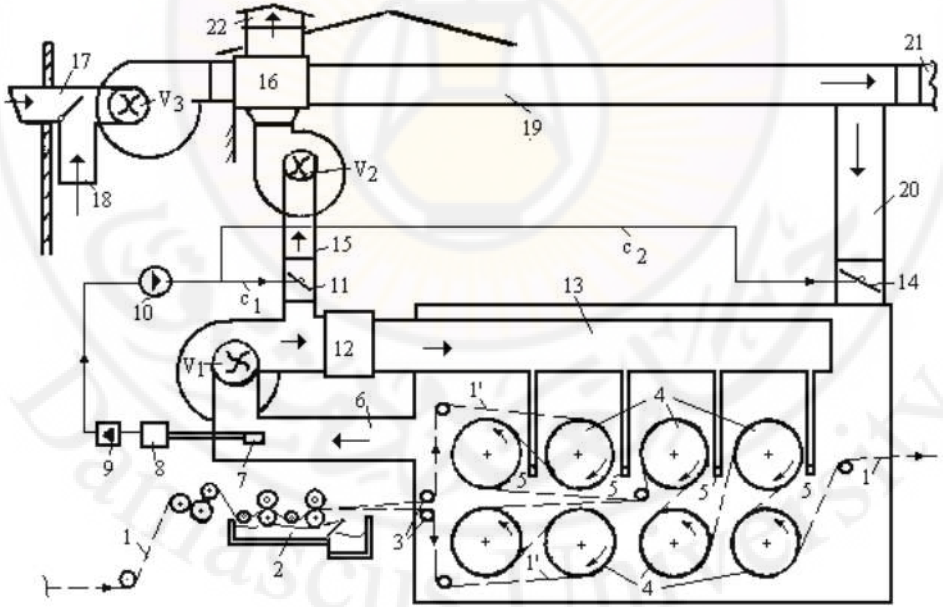
الشكل (4-26) : مجفف بنظام استعادة الحرارة
