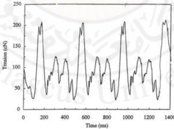
الشكل (1-4): دورات شد السداء لنسيج الدنيم ذي التصميم النسجي مبرد 1/3
