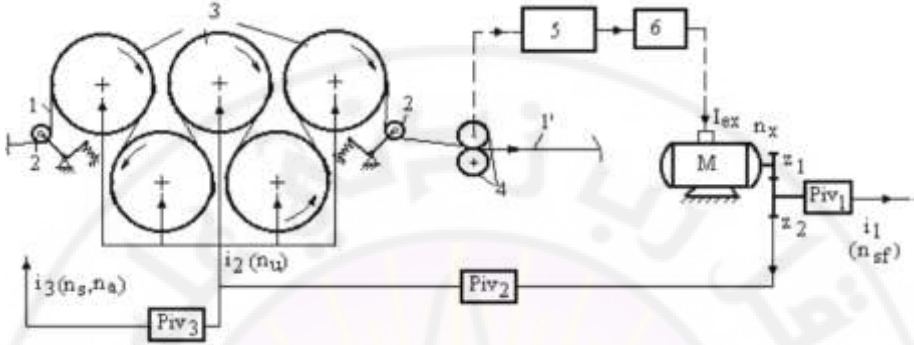
الشكل ( 4-27 ) : مبدأ قياس رطوبة السداء المنشأ
