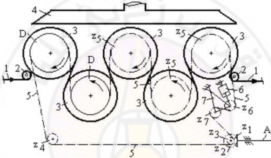
الشكل (4-21): تشغيل سلندرات التجفيف
