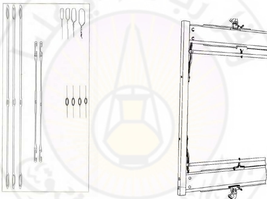
الشكل (4-5): الدراة ، ونماذج من النير (Onder, E., Berkalp, O., 2008) ,
