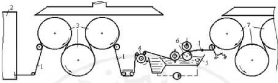
الشكل (4-24) : التجفيف المسبق للسداء بعد الصباغة (قبل التنشئة)
