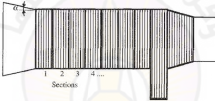
الشكل (3-5): رسم تخطيطي لشقات خيوط السداء على الطنبور بنهاية مخروطية
