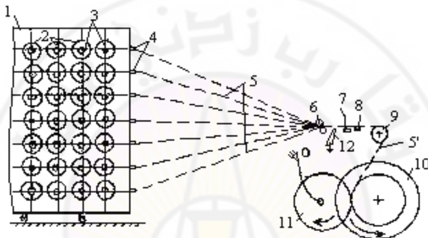
الشكل (3-3): مبدأ عمل آلة التسدية المباشرة (التسدية العرضية)
