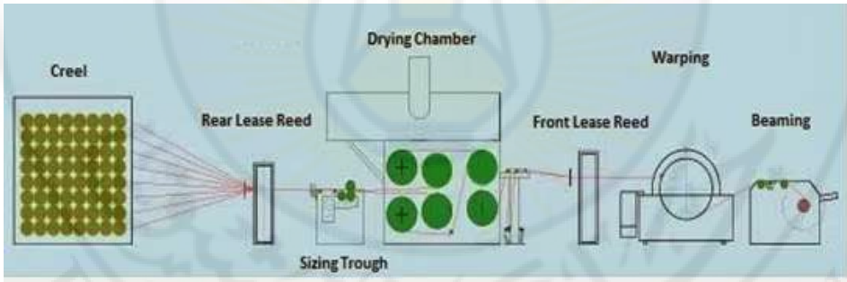
الشكل (4- 98): مخطط لآلة التبويش الجاف غير التقليدي Non-Conventional Dry Sizing
