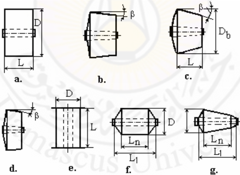
الشكل 2-6 : أنواع الكونات (Iacob, I., 2009)
