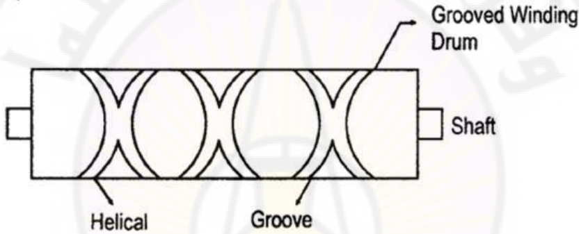
الشكل (2-21): سلندر ذو أخاديد متقاطعة Drumer with intersecting grooves
