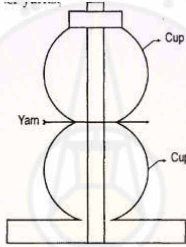
الشكل (2-19): أجهزة شد من النوع القرصي أو الدوار، (N.Gokarneshan, 2017)
