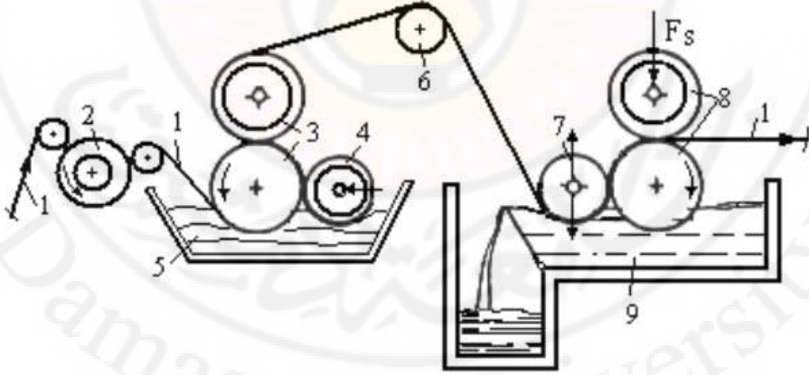
الشكل (4-18) : ترطيب السداء مسبقاً قبل التنشئة
