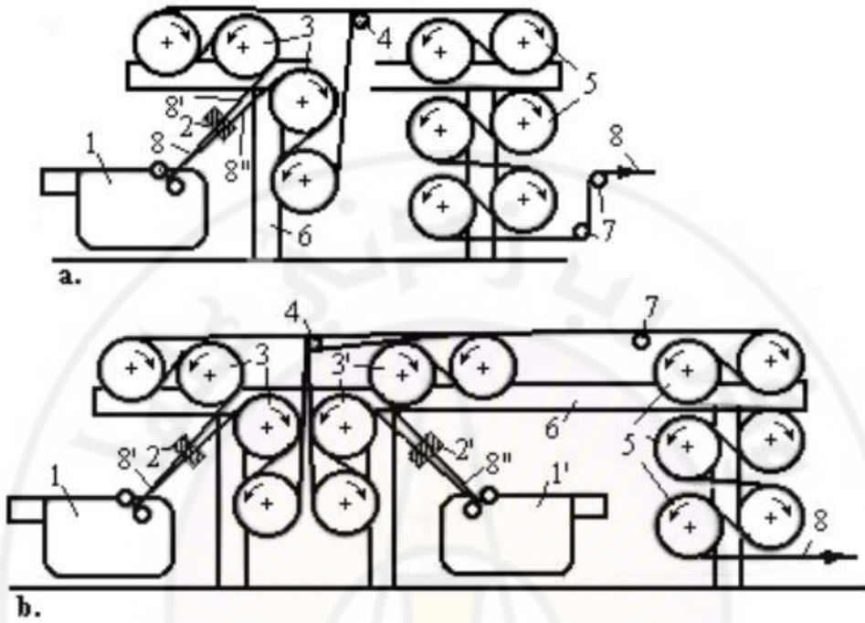
الشكل (4-23): مجففات مع فصل السداء في منطقة سلندرات التجفيف
