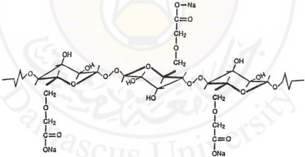
الشكل ( 35-4 ) : بنية كربوكسي ميثيل السليلوز (CMC) Carboxymethyl cellulose
