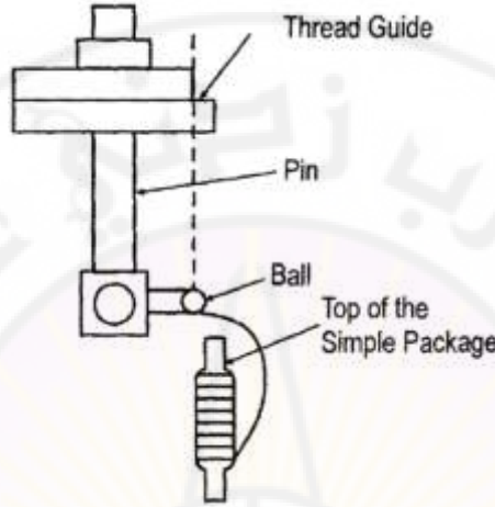
الشكل (2-17): كاسر البالون (N.Gokarneshan,2017) Balloon breaker
