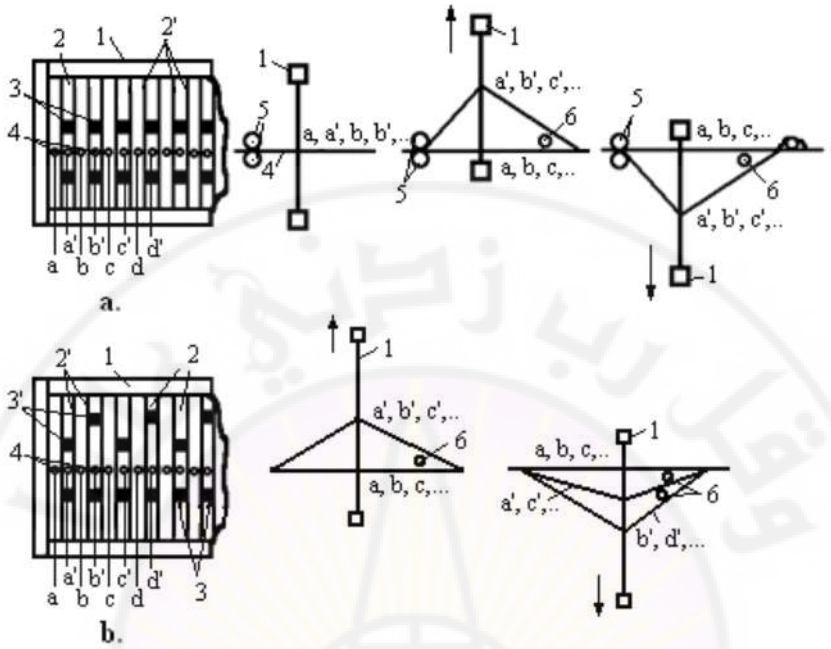
الشكل (10-3): العناصر البنائية لمشط المفصل [47].
