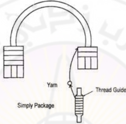
الشكل (2-18): شداد نوع الغسالة Washer type tensioner (N.Gokarneshan, 2017)
