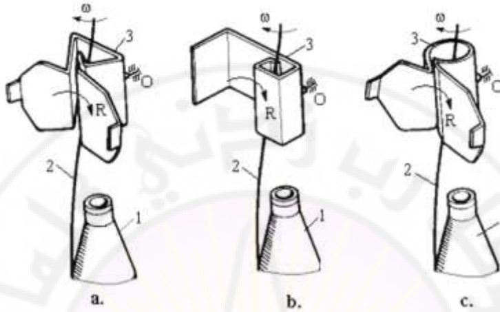
الشكل (2-3): كاسر البالون (Iacob, I., 2009)
