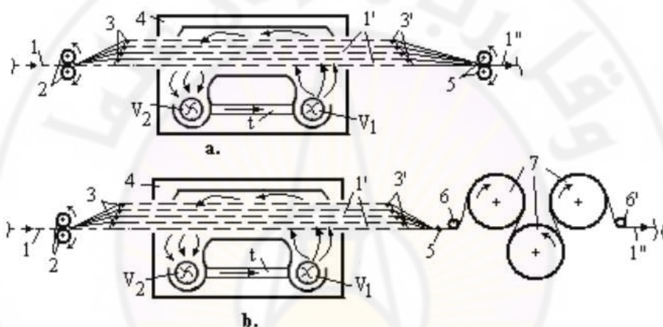
الشكل (25-4): مجففات بغرفة التجفيف
