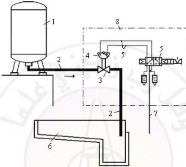
الشكل ( 4-42 ) : مبدأ تغذية حوض التنشية بالبوش
