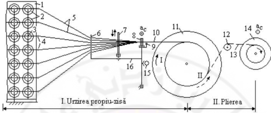
الشكل ( 8-3 ) : مبدأ اتسدية بالشقات [47].
