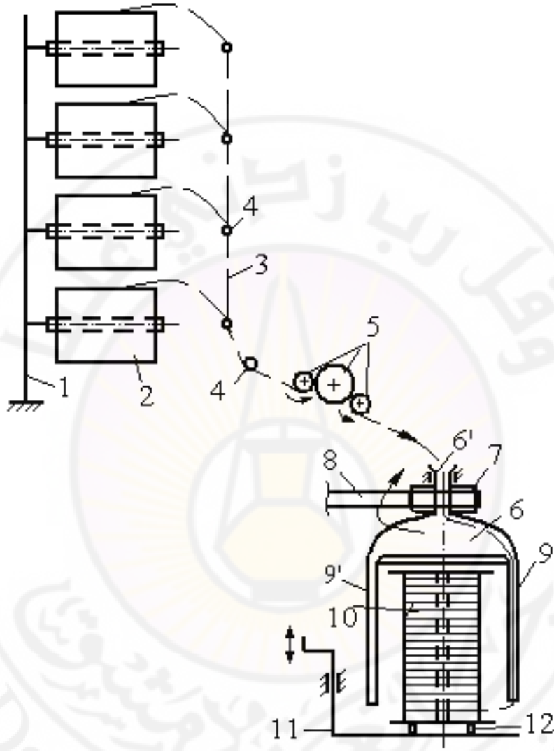
الشكل (2-41): المبدأ التكنولوجي لآلة الزوي بالشوكة
