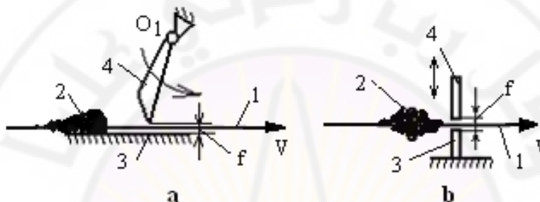
الشكل(5-2): المنظفات الميكانيكية (Iacob, I., 2009)
