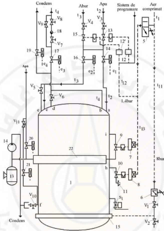
الشكل (2-14): تجهيزات الأوتوكلاف لتثبيت الخيوط
