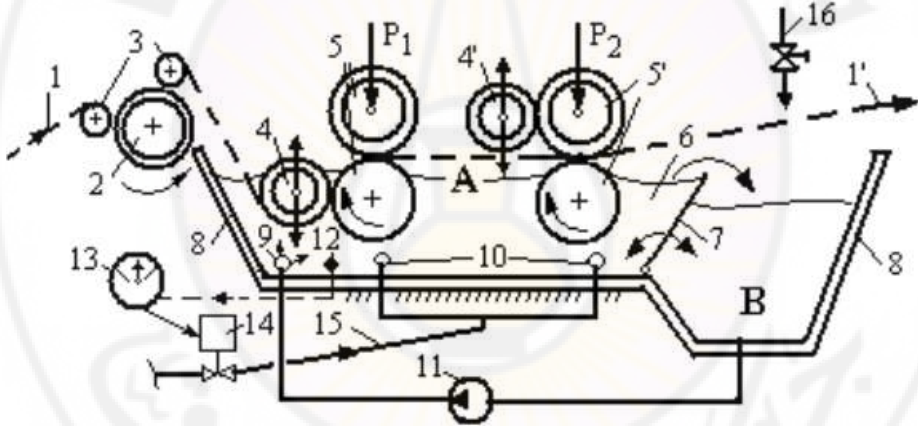
الشكل (14-4): مخطط تنشئة السداء. حوض التنشئة
