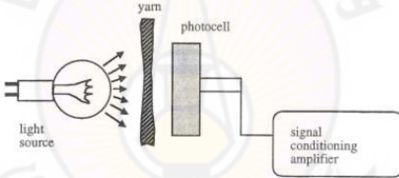
الشكل (2-32): المبادئ التخطيطية لمنظفات الخيوط الإلكترونية
