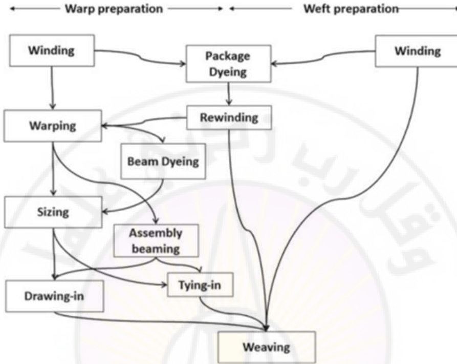
الشكل (0-1): عمليات التحضير الرئيسية لخياط السداء واللحمة [Springer Nature]
