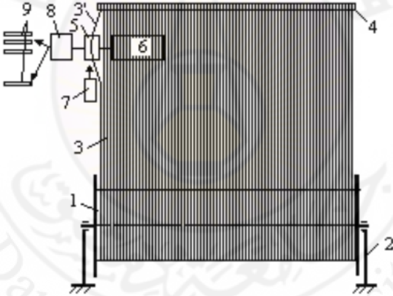
الشكل (5-6): مبدأ اللقي التلقائي لخيوط السداء في نير الدراً (Iacob, I., 2010)
