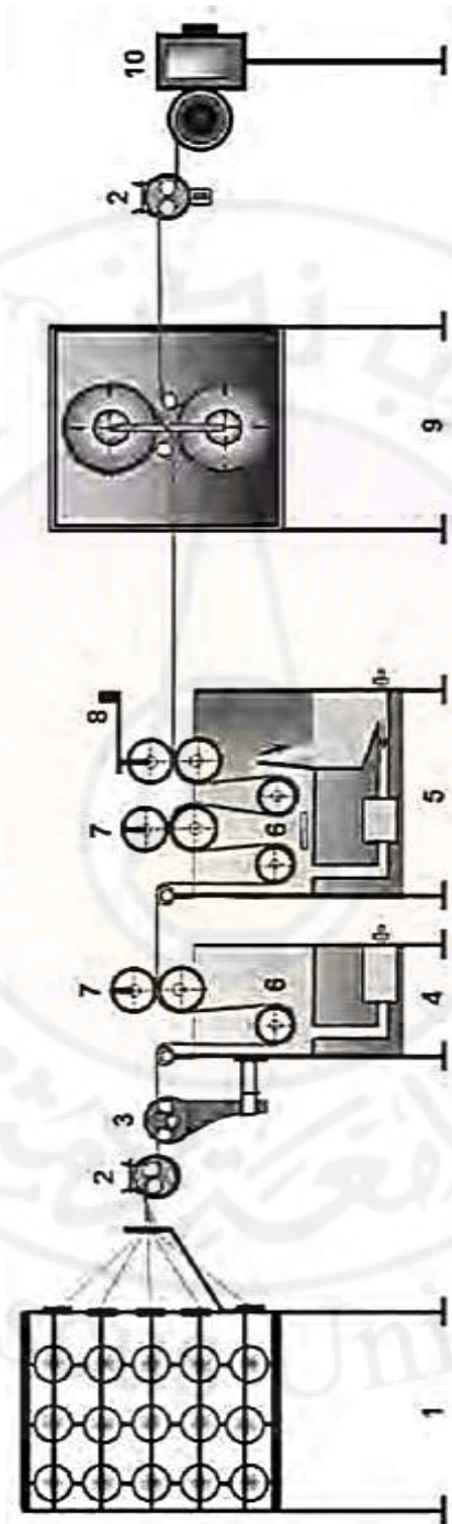
الشكل (4-55) : المخطط التكنولوجي لآلة التنشيط مع عملية الترطيب
