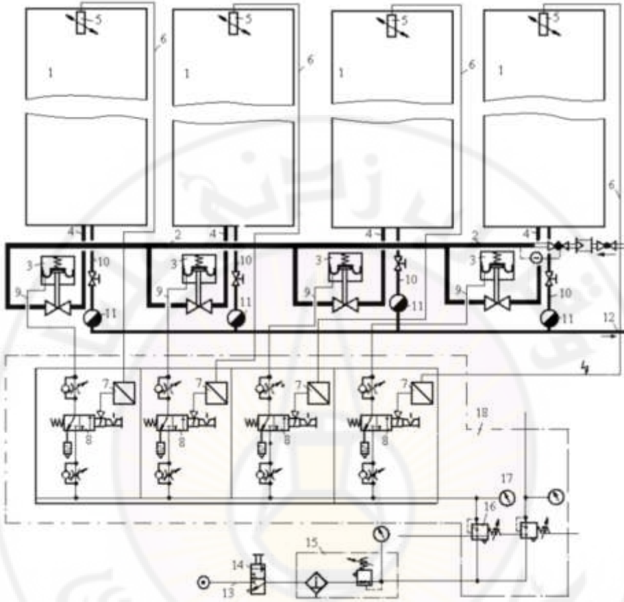
الشكل (4-22): مبدأ تسخين سلندرات المجفّف
