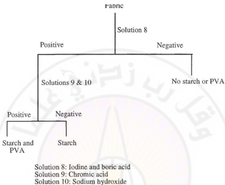
الشكل (4-59): مخطط تدفقي لتمييز خلطات النشا/PVA
