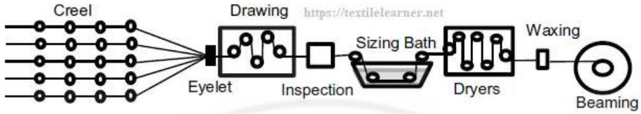
الشكل (4- 97): مخطط لآلة قياس تنشئية وسحب a draw sizing machine
