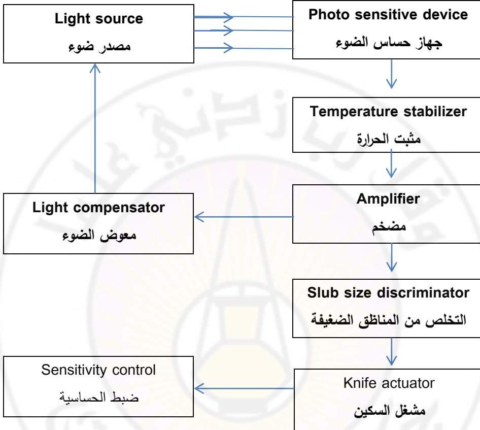
الشكل (2-43): منظف الخيط ذي الخلية الضوئية.. Photocell type electronic yarn clearer.
