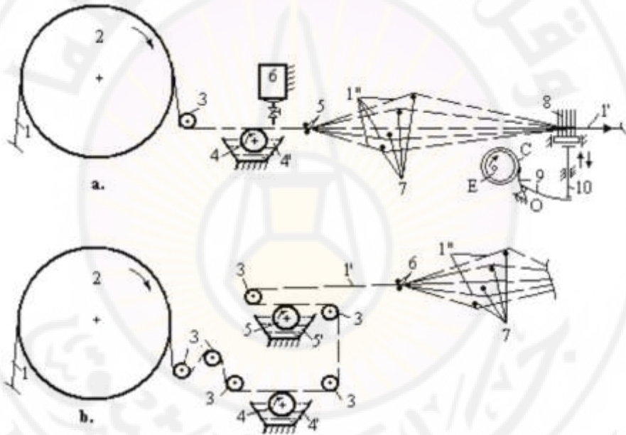
الشكل ( 4-28 ) : تشميع السداء، فصل الخيوط المنشأة
