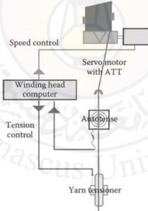
الشكل (2-44): جهاز الشد التلقائي. Autotense.
