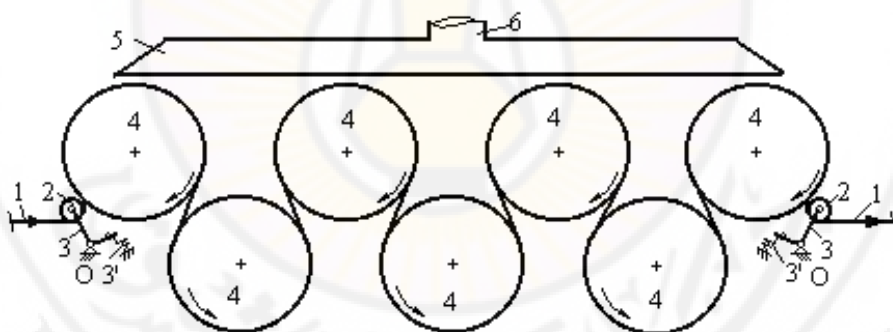
الشكل (4-20) : المجفف بسلندرات تجفيف
