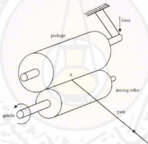
الشكل (2-35): التحريك الاحتكاكي للعبوة Friction drive of a package
