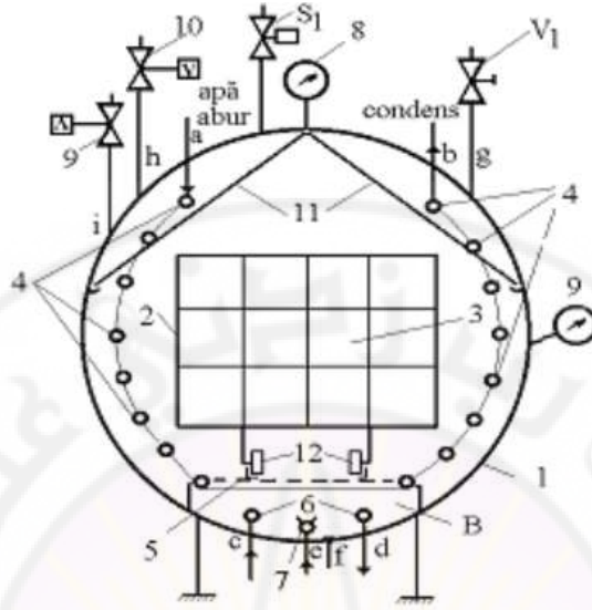
الشكل (2-13): أوتوكلاف تبخير الخيوط (Iacob, I., 2009)
