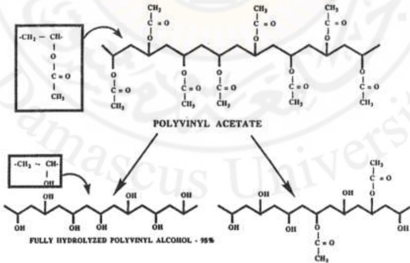
الشكل (4-34) : كيمياء كحول البولي فينيل chemistry of polyvinyl alcohol
