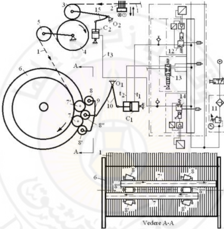
الشكل (4-29) : ضغط السداء في أثناء اللف على المطواة النهائية
