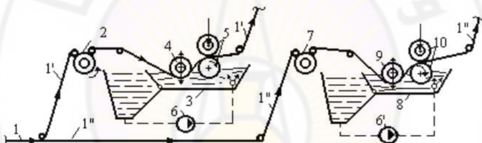
الشكل (4-17): أحواض متعددة للتنشئة
