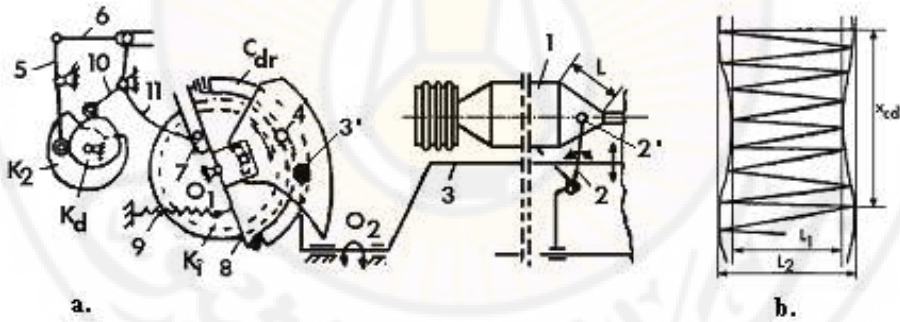
الشكل (2-10) : آلية اللف التفاضلي للخيط على الماسورة
