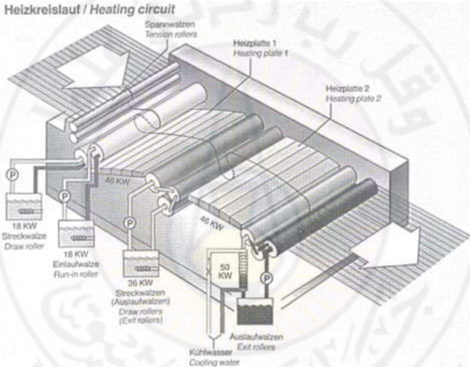
الشكل (3-14): رسم تخطيطي لعملية التسدية السحابية (Adanor, S., 2001)
