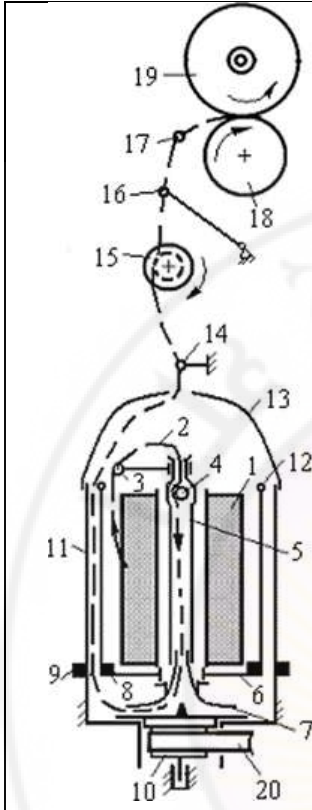
الشكل (2-38): المخطط التكنولوجي لآلة الزوي ذات البرم المزدوج
