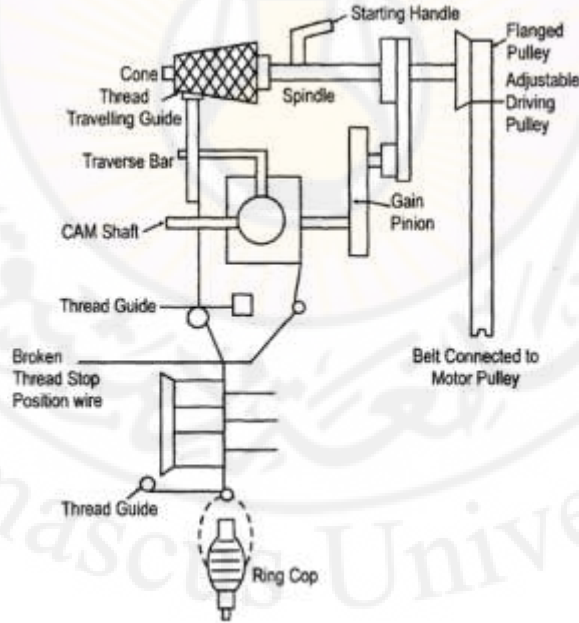
الشكل (2-25): مرور الخيط من خلال آلة التدوير (اللفاف) الدقيقة
