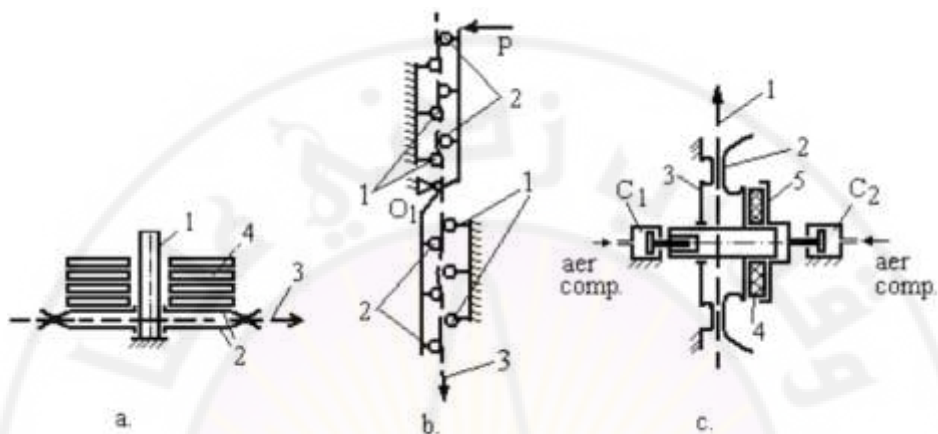
الشكل (2-4): مبادئ شد الخيوط في أثناء اللف (Iacob, I., 2009)
