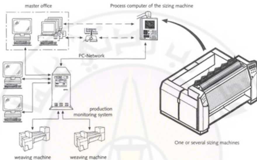
الشكل (4-8): آلات التبويش كجزء من أنظمة التحكم والمراقبة (Sucker Muller Hacoba)
