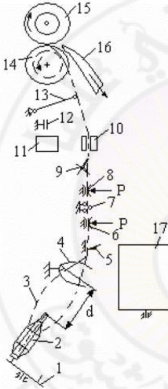
الشكل ( 2-2): المبدأ التكنولوجي لآلة اللف (Iacob, I., 2009)
