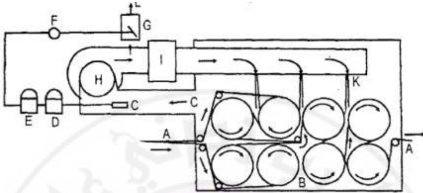
الشكل (4-67): نظام توفير الطاقة النموذجي في التجفيف
