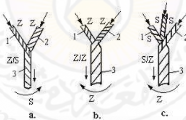
الشكل (2-37): اتجاه برم الخيوط عند الزوي
