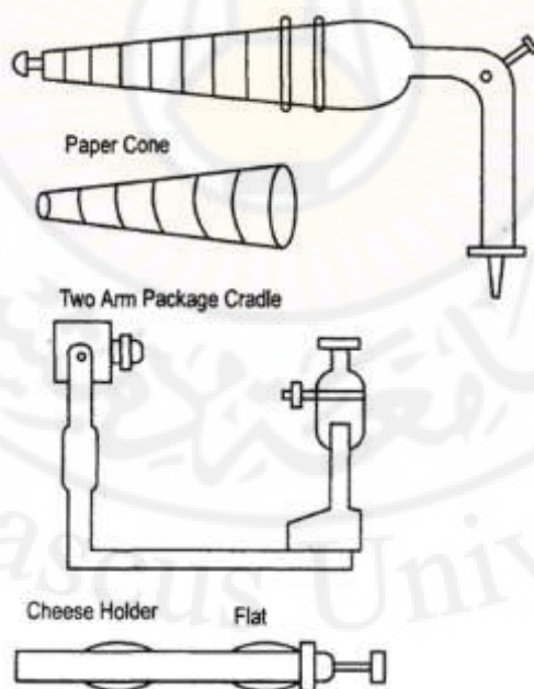
الشكل (2-23): أنواع حاملات المخروط Types of cone holders
