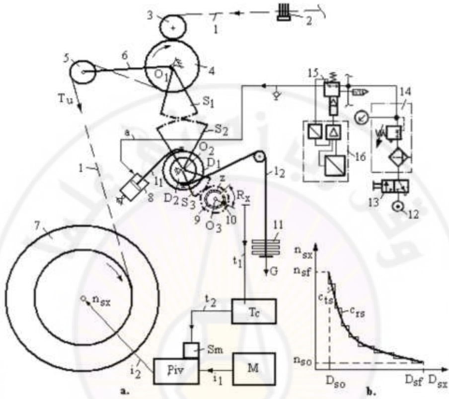
الشكل (4-30) : جهاز اللف على آلة التنشية
