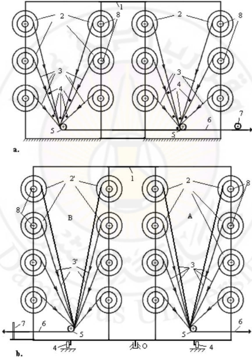
الشكل (4-11): نصابات تغذية مطاوي السداة للتنشئة
