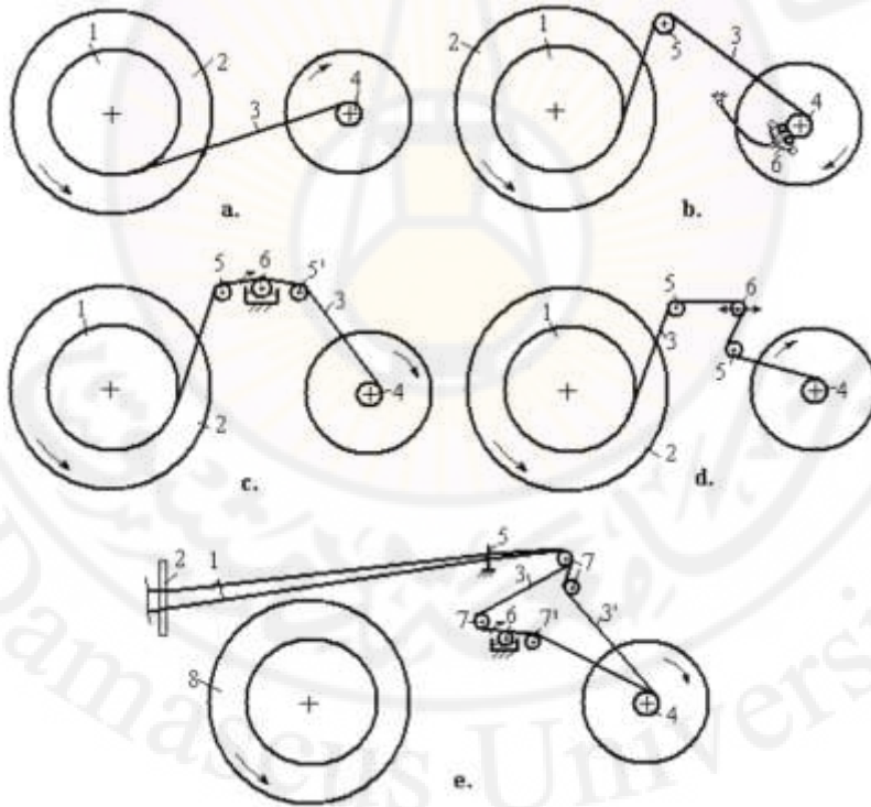
الشكل (3-9): مبدأ تشكيل لف السداء النهائي على آلة التسدية بالشفق
