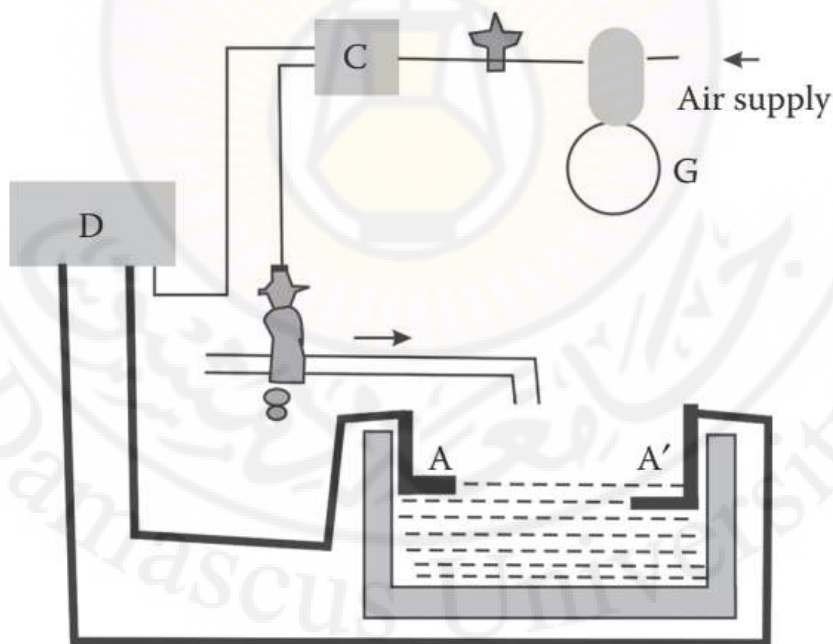
الشكل (4-64) : التحكم في مستوى النشاء.
