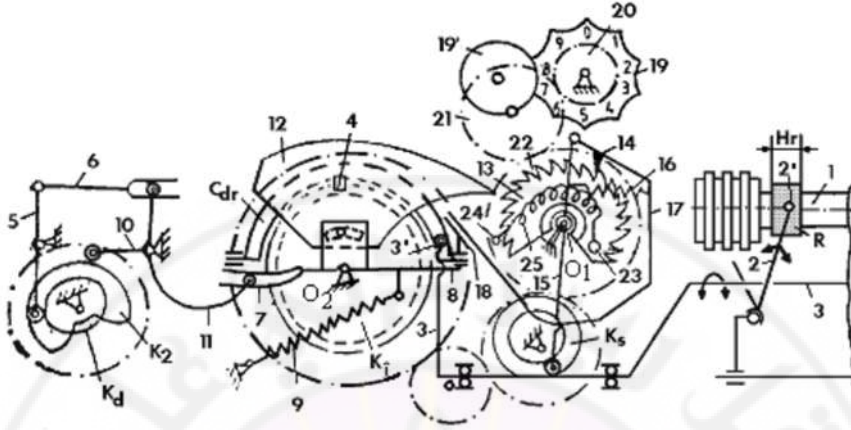
الشكل (2-11): آلية لف الطول الاحتياطي
