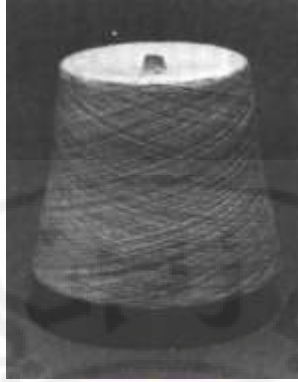
الشكل (2-49): مخروط على شكل جرس Bell shaped Cone (Gokarneshan, N., 2009,P92)
