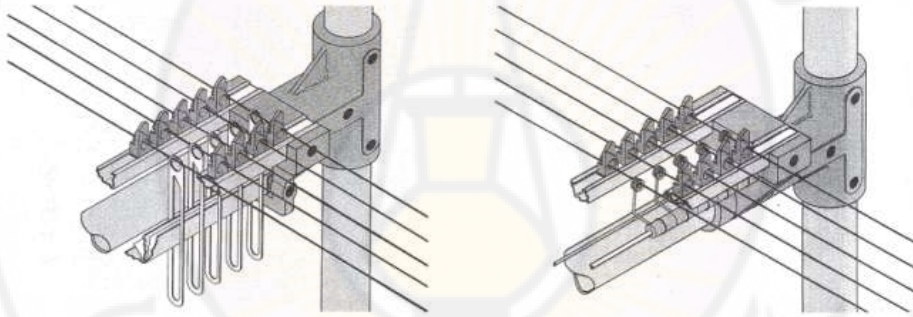
الشكل (3-19): شفرات حساس خيط السداء (يساراً)، وسلك حساس (يميناً).
