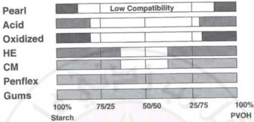
الشكل (4-33) : مدى توافق النشاء مع PVA
