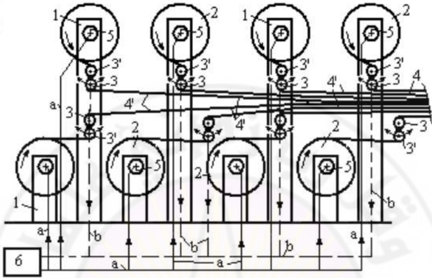
الشكل (4-13-ب): نسبة التغذية مع محركات موازنة servomotrs لقيادة مطاوي التغذية
