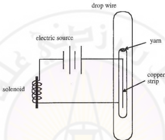
الشكل (5-2): رسم تخطيطي كهربائي لإيقاف حركة السداء warp stop motion
