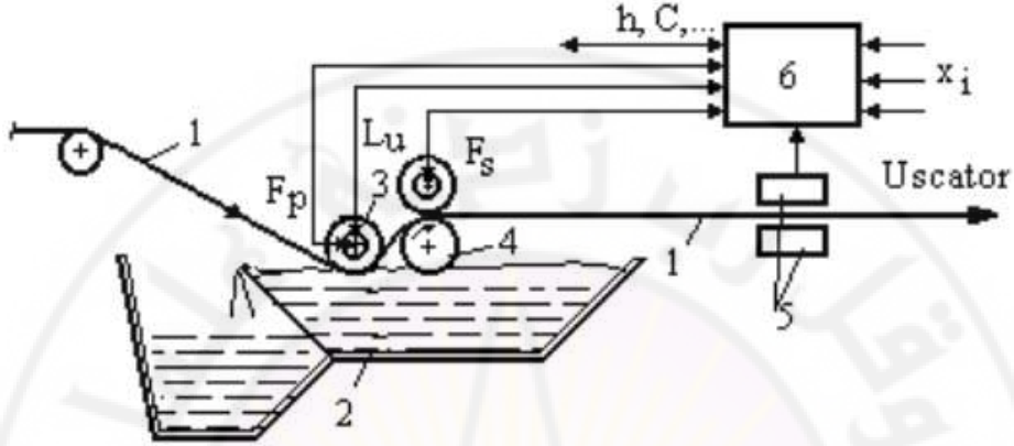
الشكل (4-19): مبدأ قياس تحميل السداء بالنشاء في المنطقة الرطبة
