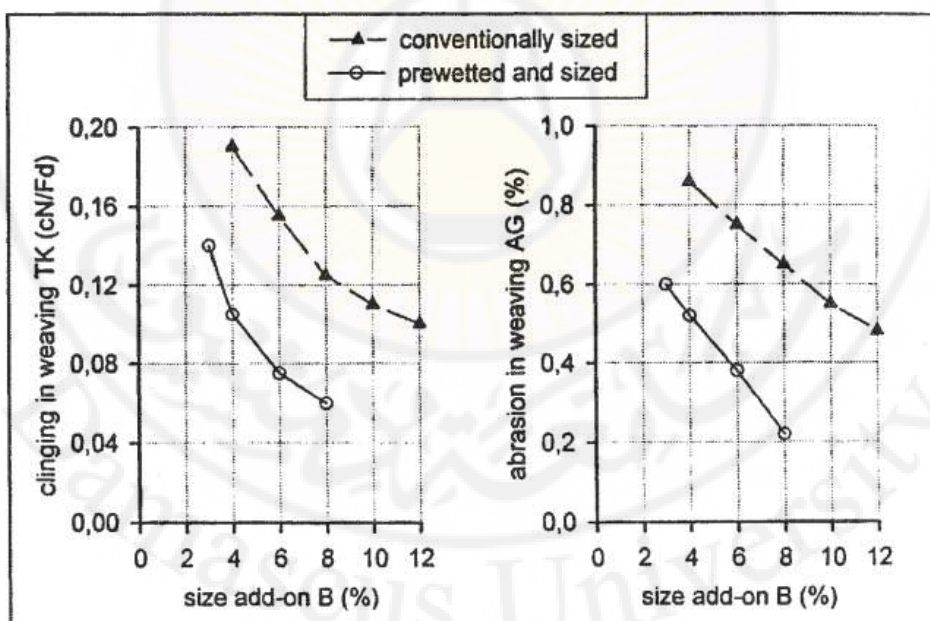
الشكل (4-47): مقارنة سلوك النسج للخيوط ذات التبيوش التقليدي والخيوط ذات التبيوش بالترطيب
