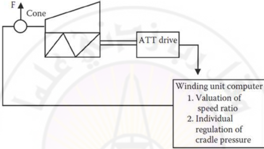
الشكل (2-46): نظام بروباك Propack
