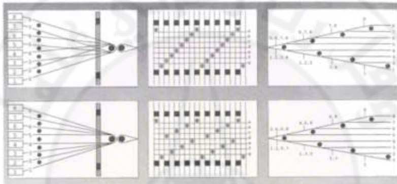
الشكل (3-81): سحويات "مباشرة" و"تخطي فردي
