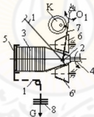
الشكل (2-12) : مبدأ الحصول على المواسير دون حامل
