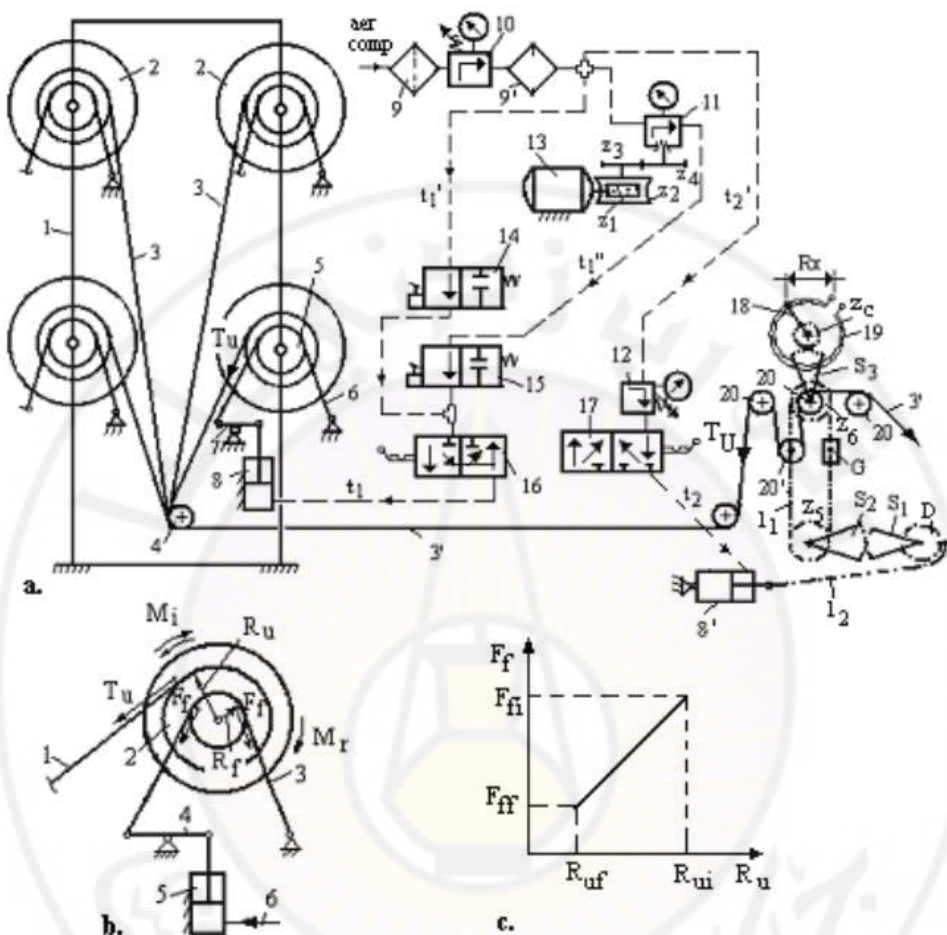
الشكل (4-12): مبدأ المعايير التلقائية لقوة كبح مطاوي السداء في نسبة التغذية.
