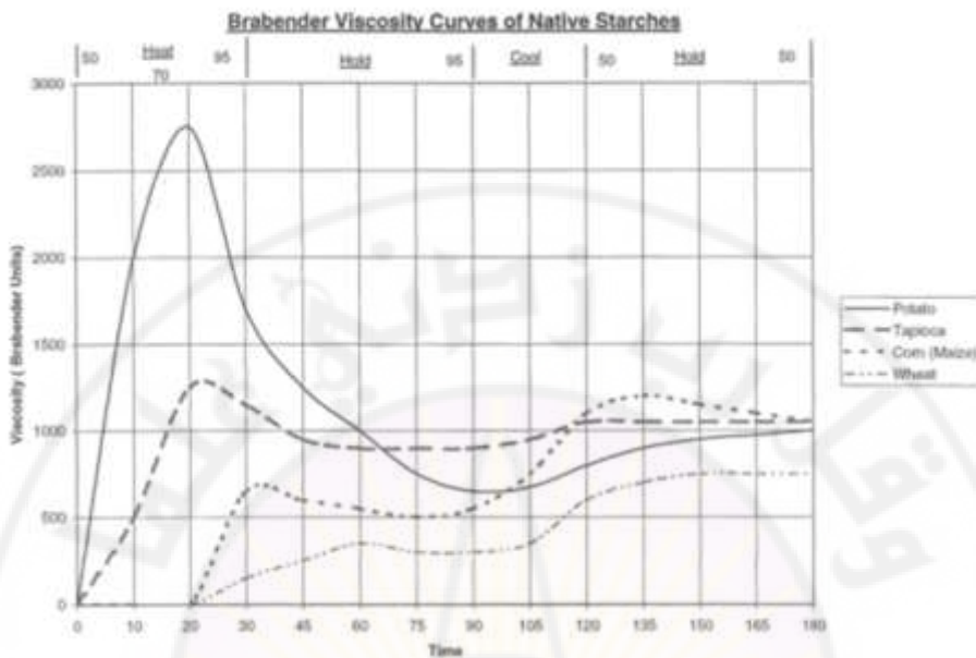
الشكل (4-33) : منحنيات لزوجة النشا Starch viscosity curves .
