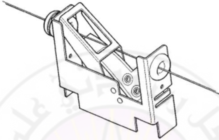
الشكل (3-20): رسم تخطيطي لحركة إيقاف الخيط الحساسة للاهتزاز
