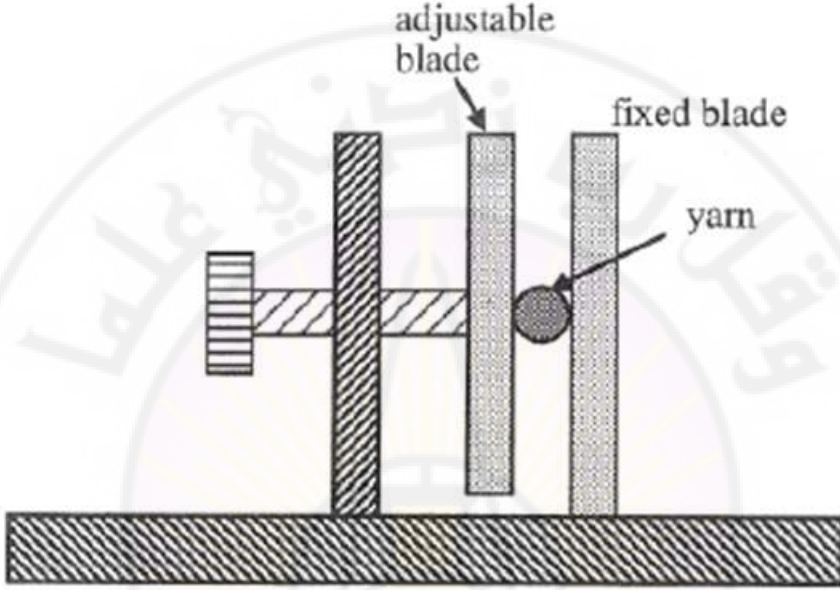
الشكل (2-31): المبدأ التخطيطي لمنظف لغزل الميكانيكي (Adenor, S., 2001)
