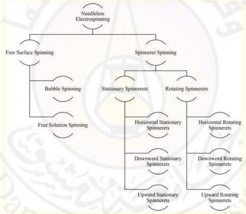
الشكل 7-8: طرق تصنيف الغزل الكهربائي
