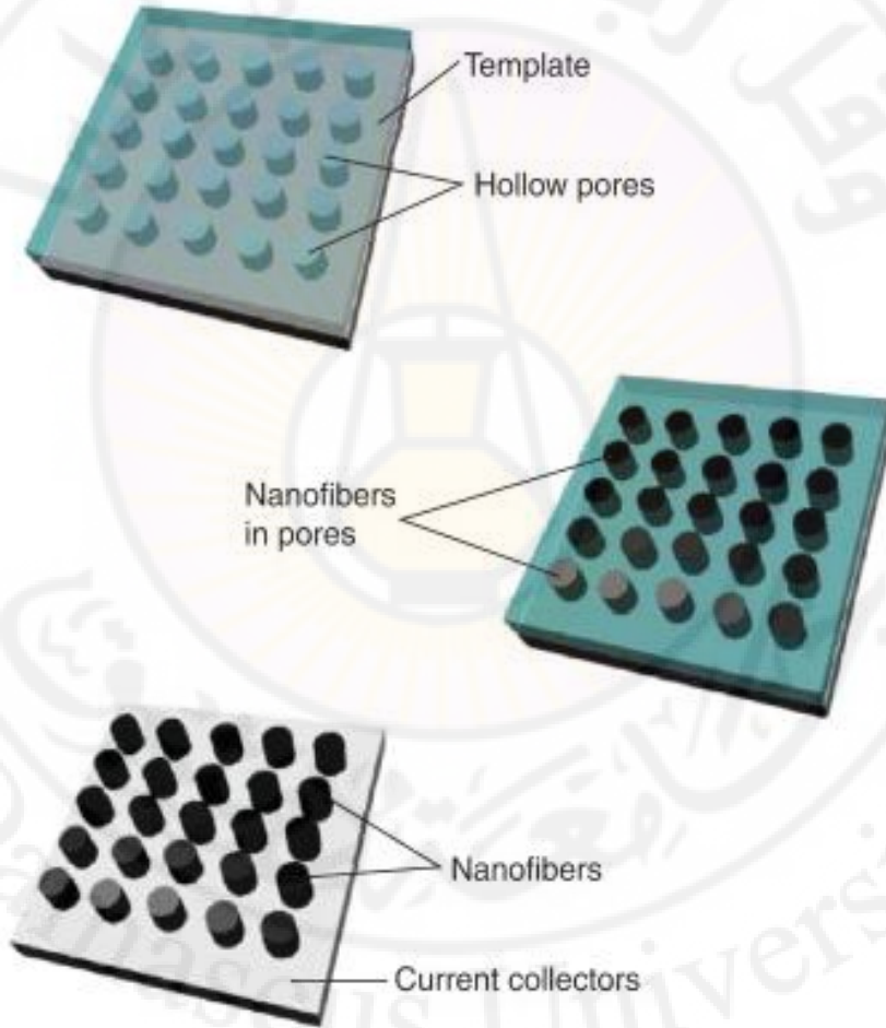
الشكل 8-13: قالب التوليف Template synthesis هو وسيلة لإعداد الألياف النانوية (B. Meyer, F. Croce, 2009)
