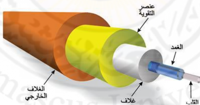
الشكل 5-8: مقطع عرضي للليف زجاجي بصري
