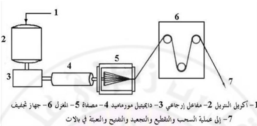
الشكل 4-18: يوضح طريقة إنتاج الأورلون
