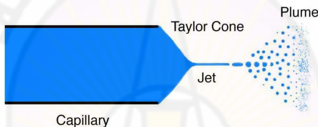
الشكل 8-5: مخروط تايلور الذي يتم دفع محلول Taylor cone from which jet of polymer solution is ejected
