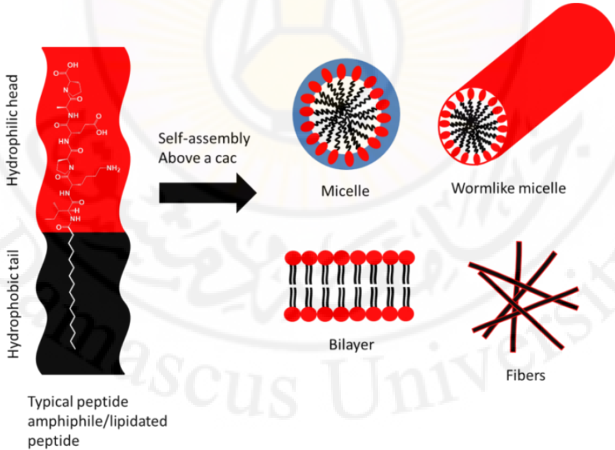
الشكل 8-15: مخطط لإظهار الهياكل المحتملة المجمعة ذاتياً من أمفيڤيلات الببتيد النموذجية peptide amphiphiles
