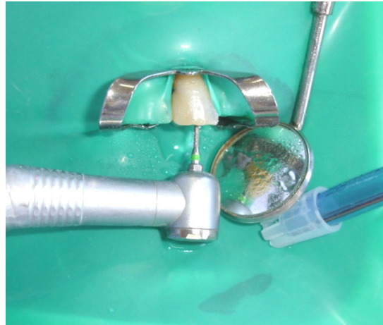
الشكل رقم (50-2) يوضح النفوذ ضمن العاج باستخدام سنبلّة ماسية بعمق 1-2 ملم.
