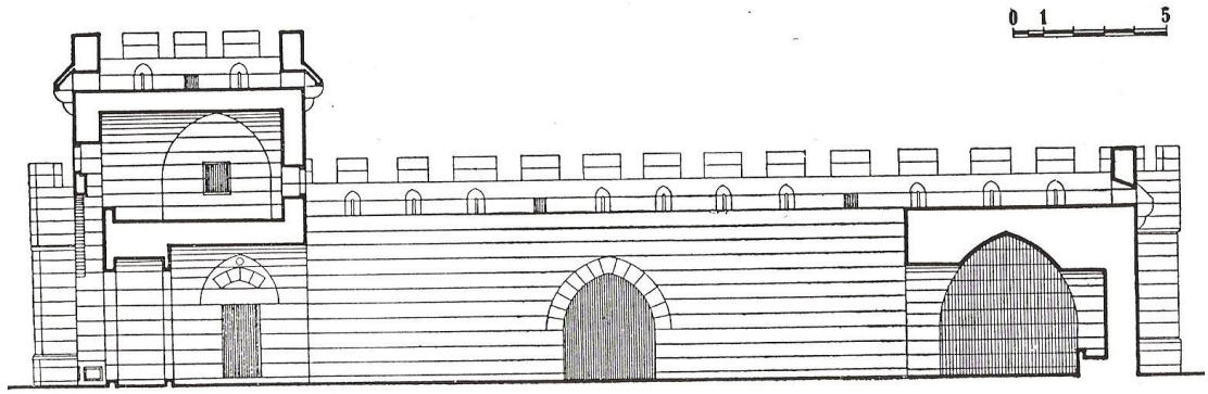
FIG. 17. — Le caravansérail d'Inqirâtâ : coupe suivant l'axe.
