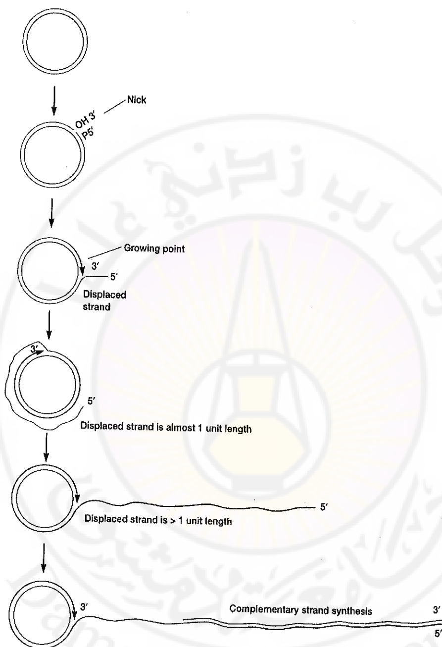
الشكل 4-39 نموذج تضاعف الحلقة المتحركة
