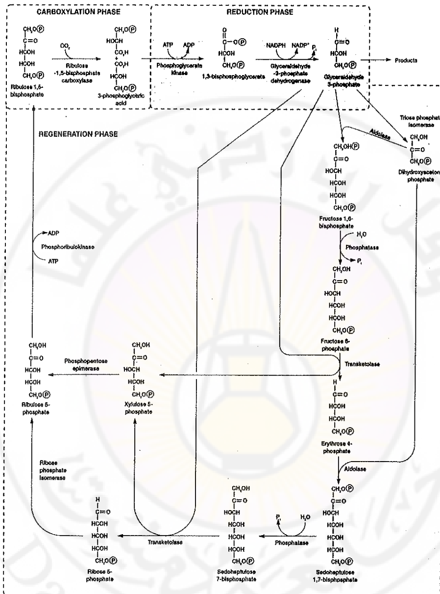
الشكل 3-4 حلقة كالفن Calvin Cycle بأطوارها الثلاثة
