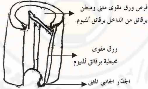
الشكل (2-6): عبوات من الكارتون برميلية الشكل
