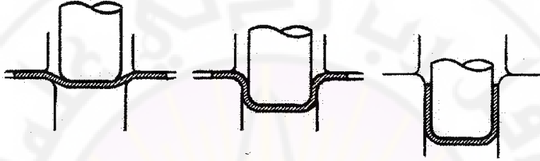
الشكل (1-6) خطوات تصنيع علب الألومنيوم بطريق الضغط في القوالب
