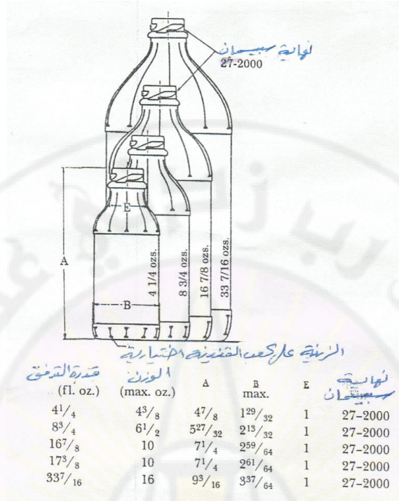
د - زجاجة مستديرة ذات رقبة قصيرة الشكل (1-4) أشكال مختلفة من الأوعية الزجاجية
