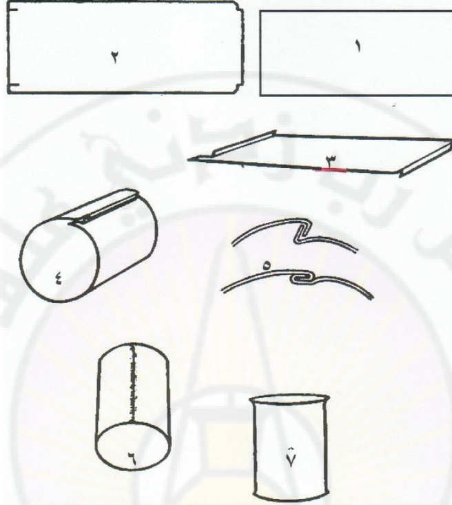
الشكل (3-4) خطوات صناعة علب الصفيح
