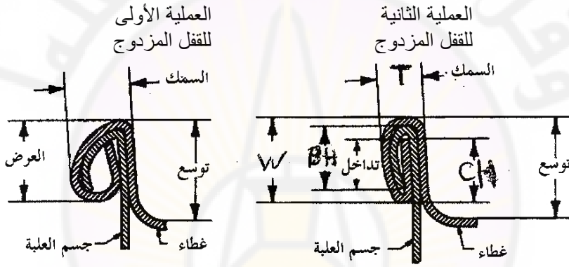
الشكل (3-15) تسمية أبعاد القفل المزدوج
