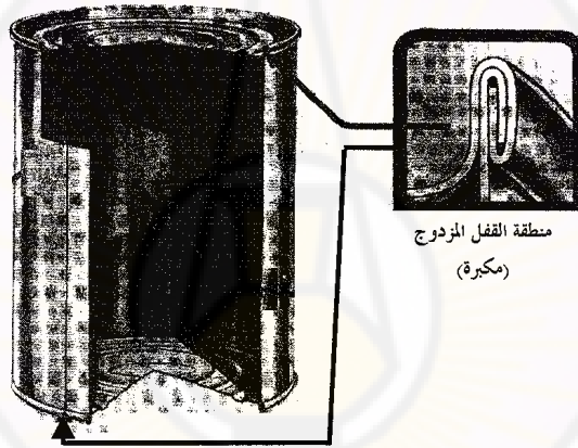
الشكل (3-5) يبين منطقة القفل المزدوج
