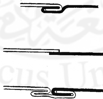
شكل (3-6): أشكال اللحام الجانبي لعلب الصفائح
