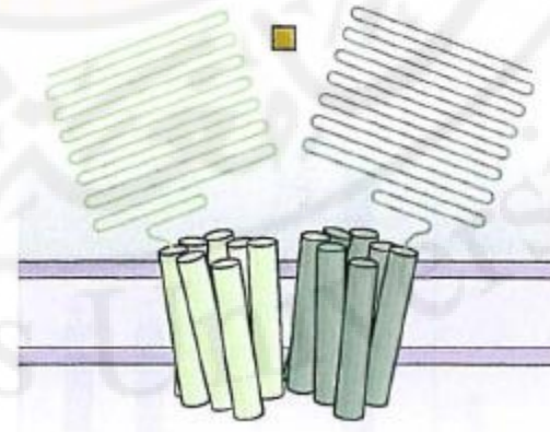
Umami (T1R1 + T1R3)
