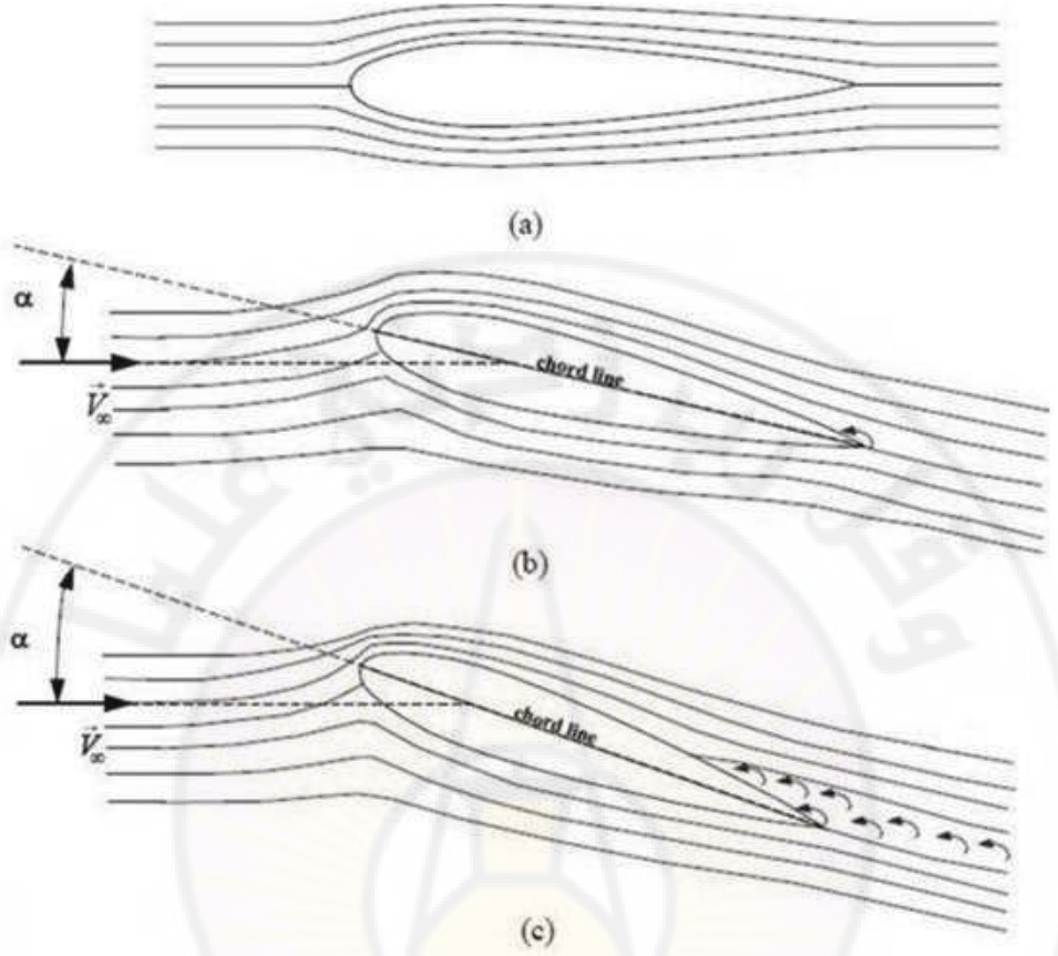
الشكل (4-5): الجريان حول بروفييل جناح متناظر بقيم مختلفة لزوايا الهجوم \alpha
