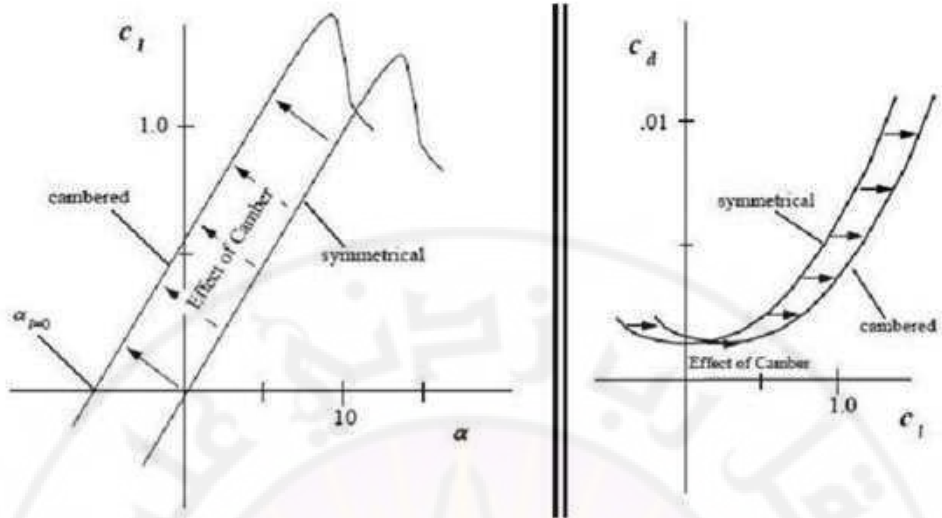
الشكل (4-7): متحنيا كل من عامل الرفع ( c_l ) وعامل الجر ( c_d ) لبروفيلي جناح متناظر ومقعر
