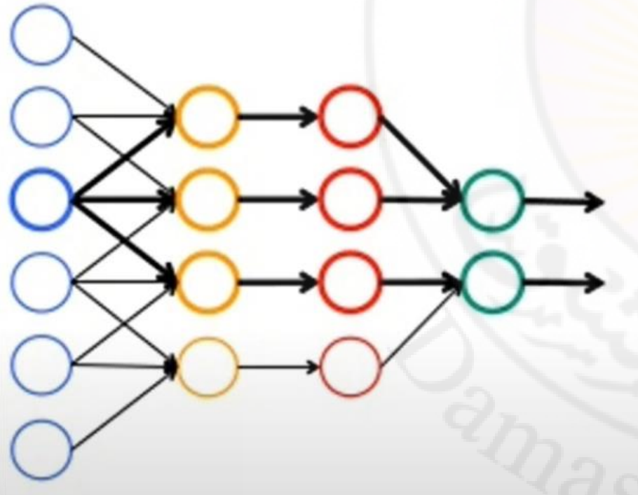
مسار البيانات الأمامي
