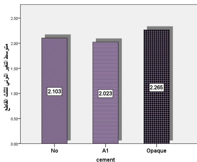
مخطط رقم (24): يمثل المتوسط الحسابي لقيم التغير اللوني للثلث القاطع \Delta E(I) وفقاً لتطبيق الإسمنت اللاصق (أثر رئيسي)
