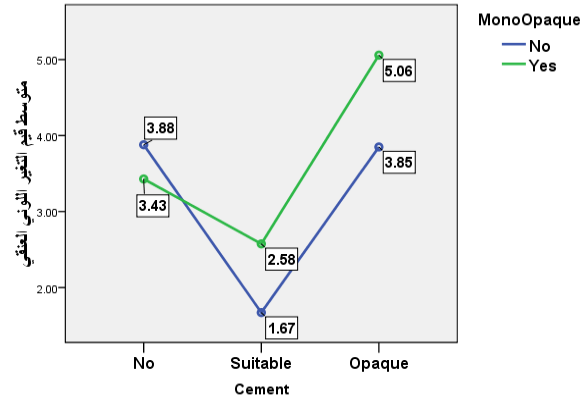
مخطط رقم (41): يبين التفاعل بين تطبيق المعدل اللوني ومراحل الإسمنت اللاصق الثلاث (لا يوجد)، (موافق)، (ظليل)
