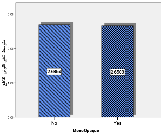
مخطط رقم (90): يبين الأثر الرئيسي لتطبيق المعدل اللوني على التغير اللوني القاطع في مجموعة الإسمنت الظليل مع الشاهدة
