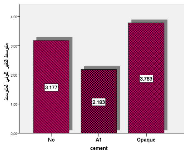
مخطط رقم (48): يبين الأثر الرئيسي لنوع الإسمنت اللاصق على التغير اللوني المتوسط
