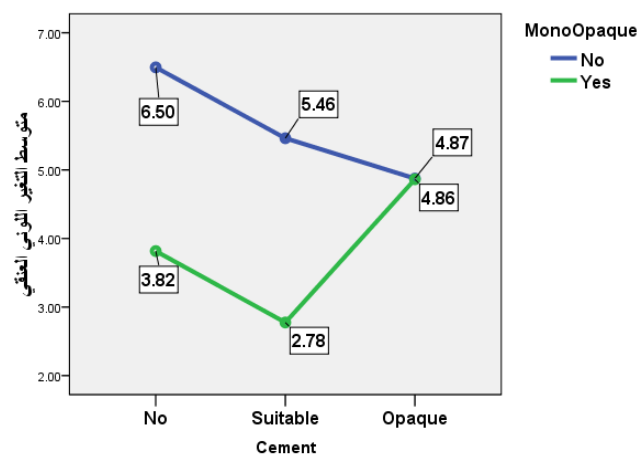
مخطط رقم (68): يبين التفاعل بين تطبيق المعدل اللوني ومراحل الإسمنت اللاصق الثلاث (لا يوجد)، (موافق)، (ظليل)
