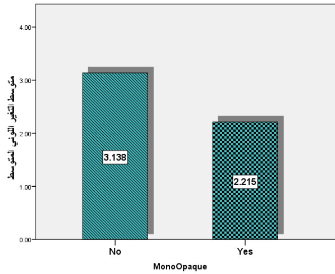
مخطط رقم (80): يبين الأثر الرئيسي لتطبيق المعدل اللوني على التغير اللوني المتوسط في مجموعة الإسمنت الموافق مع الشاهدة
