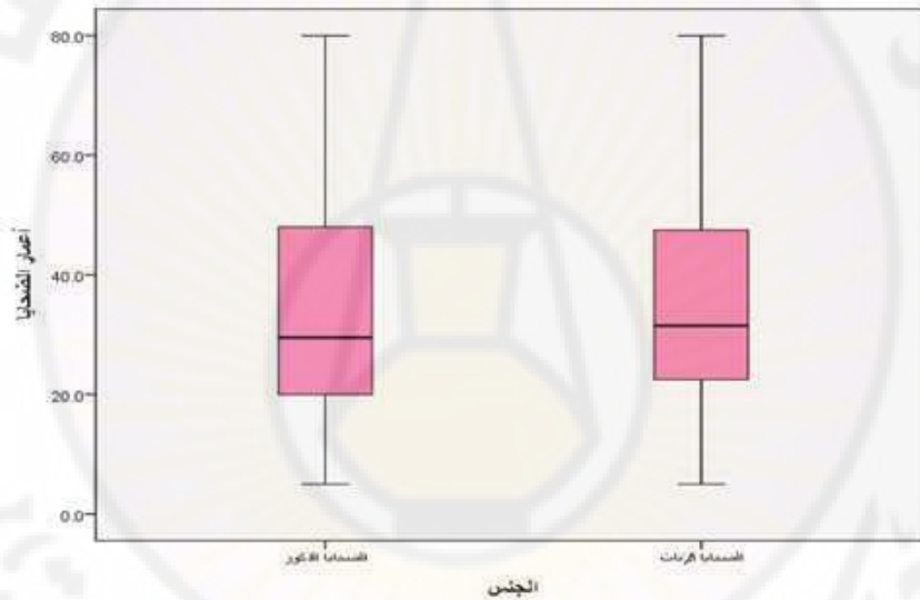
الشكل (4-7) مخطط صندوقي لتوزيع وتشتت أعمار ضحايا حوادث المرور
