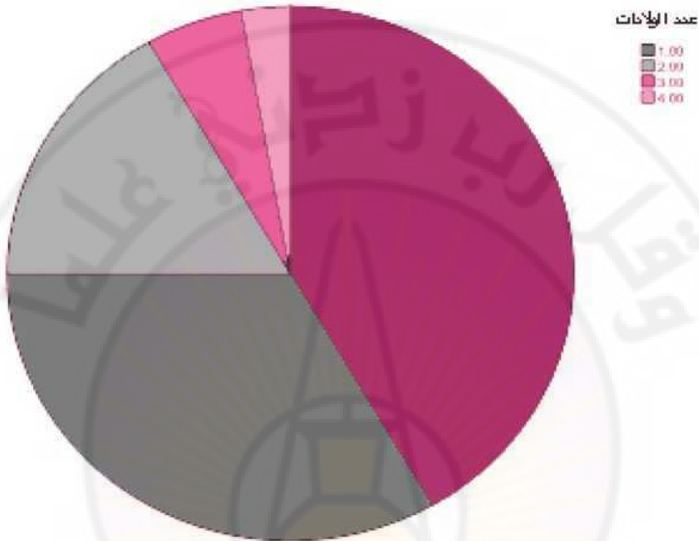
الشكل (8-4) مخطط الدائرة لعدد الولادات
