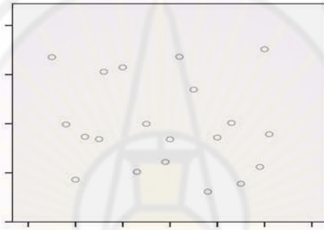
الشكل (2-9) شكل مخطط الانتشار لمتغيرين لا علاقة بينهما
