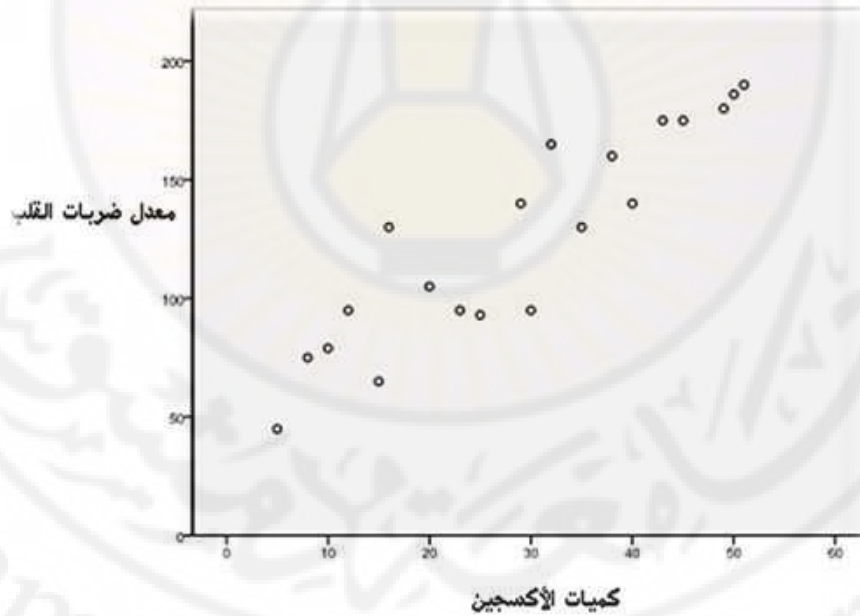
الشكل (9-1) مخطط الانتشار لكمية الأوكسجين ومعدل ضربات القلب.
