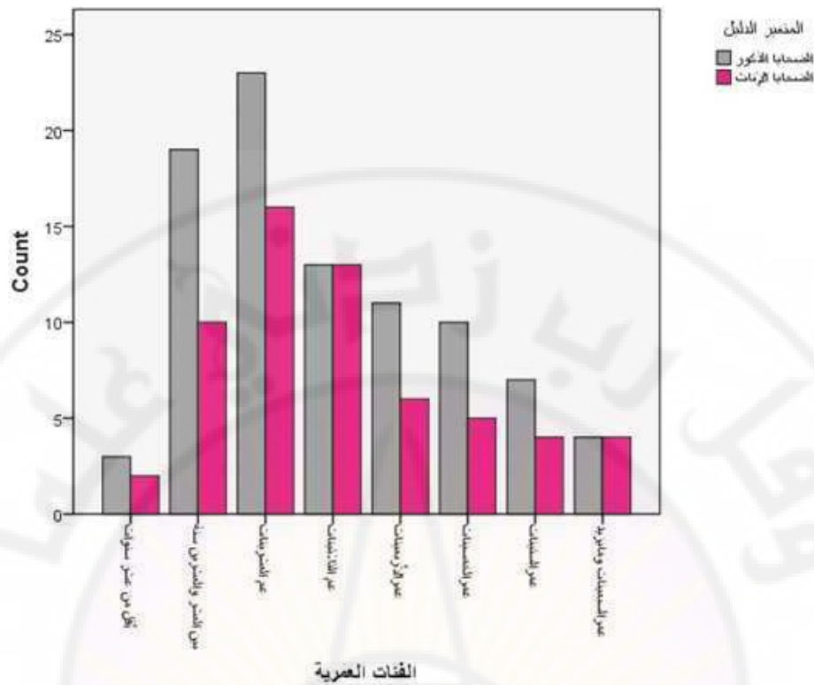
الشكل (4-4) مخطط الأعمدة المركب لمقارنة أعداد العينتين في كل فئة عمرية
