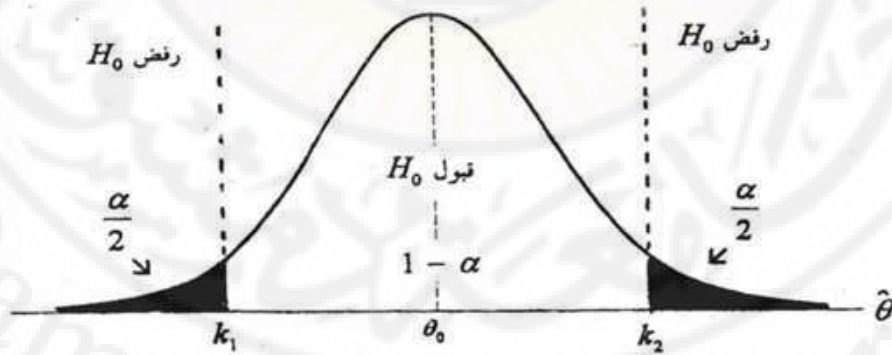
الشكل 3.7 (3.7) المنطقة المظللة لـ H_1 : \theta \neq \theta_0
