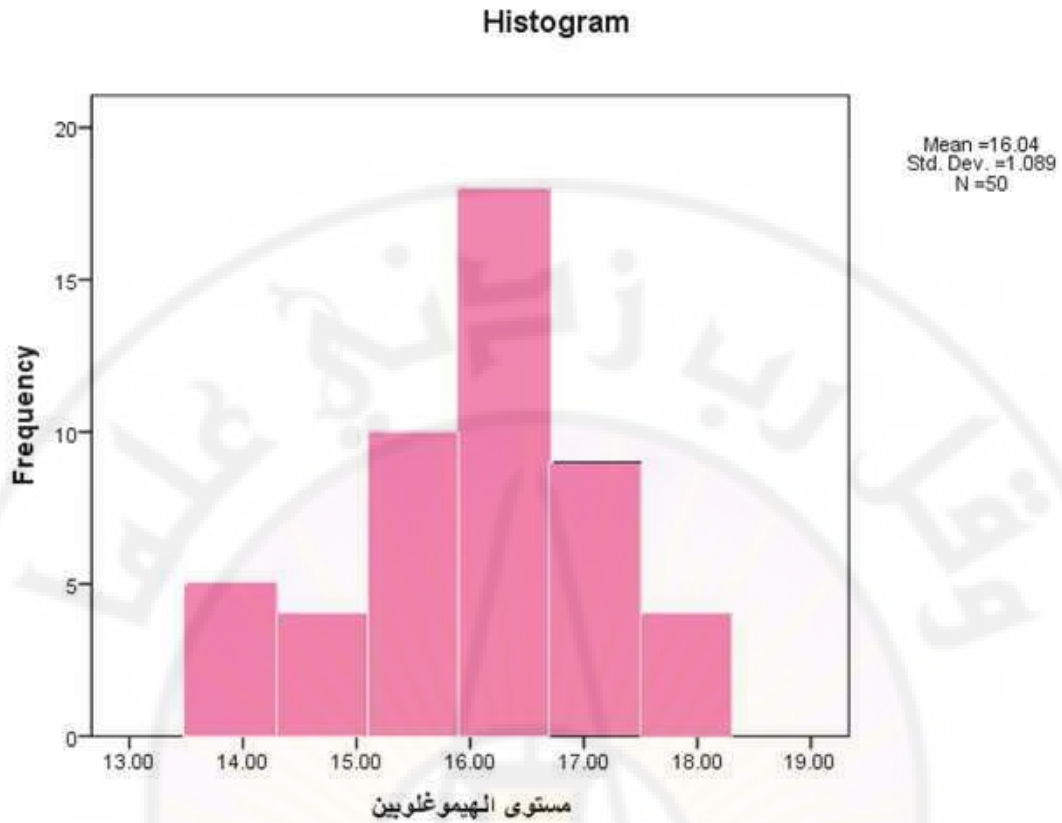
الشكل (4-2) المدرج التكراري لمستوى الهيموغلوبين
