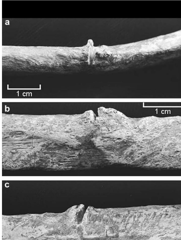
(الشكل ٨٢) الضلع التاسع من شانيدار ٣ ويظهر عليه آثار الجرح بثلاث صور مكبرة بثلاث وضعيات:
