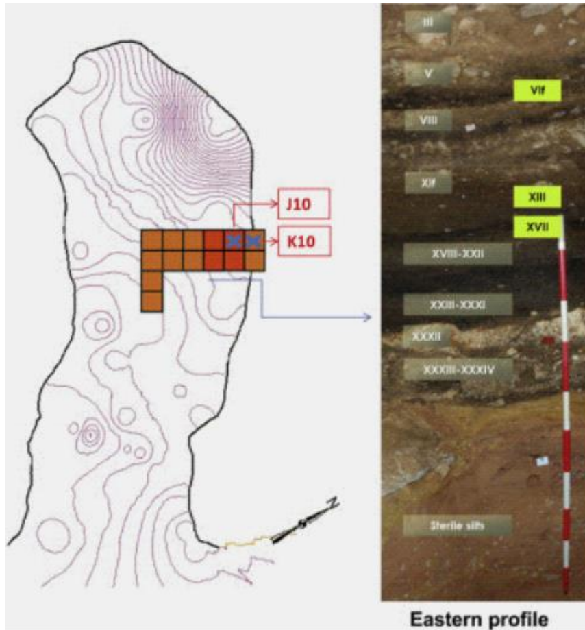
(الشكل ٢١) مخطط كهف أسكويلىو، ومكان التنقيبات وتسلسل الطبقات الأثرية فيه (الصفحة الرسمية للموقع على الأنترنت)
