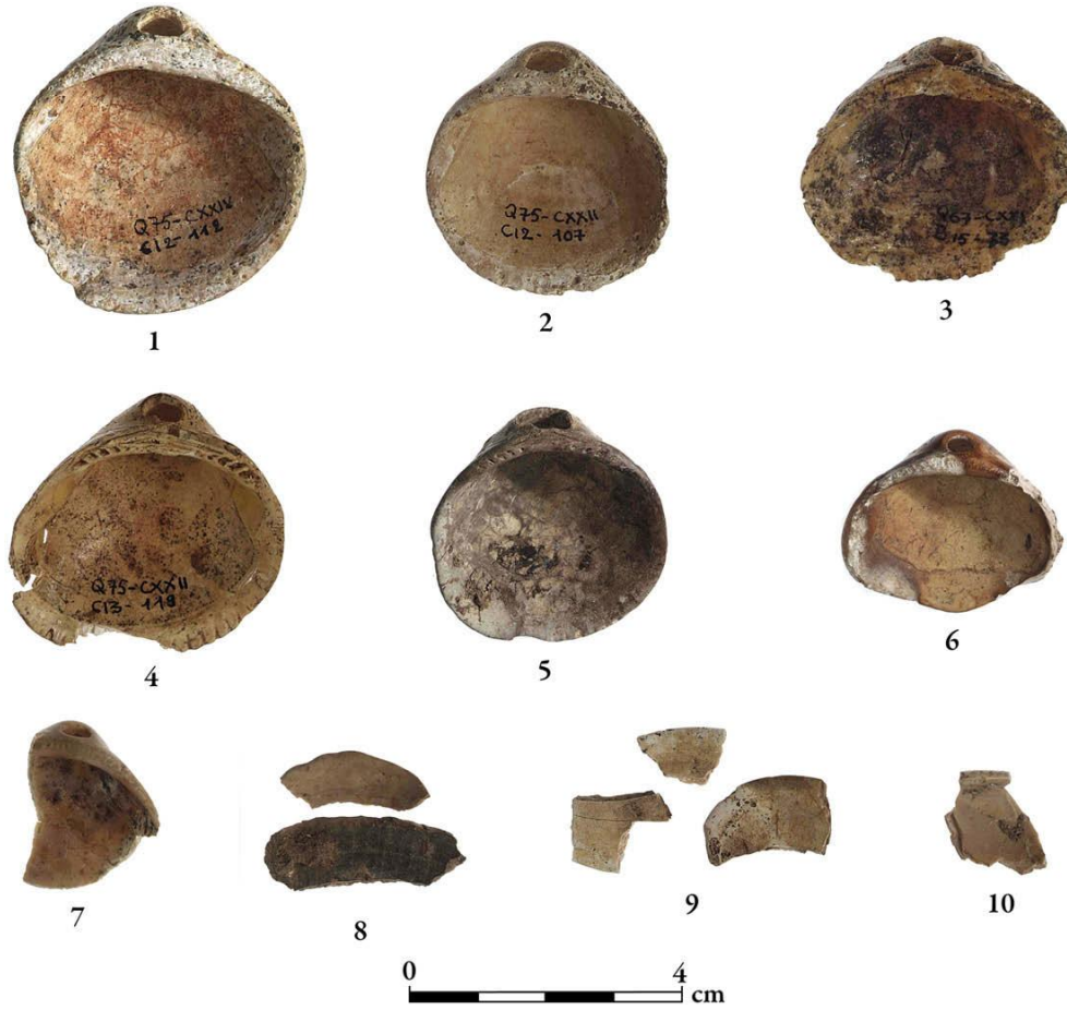
(الشكل ١٠٧) أصداف كهف قفزة من نوع Glycymeris insubrica ويتراوح قطرها ما بين ٤ - ٧ سم
