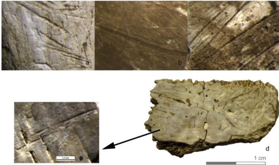
(الشكل ٨٨) علامات قطع على الجانب الداخلي من قوقعة سلحفاة، من موقع لاكويبرادا تبين استهلاك النياندرتال للزواحف، نقلا عن:
