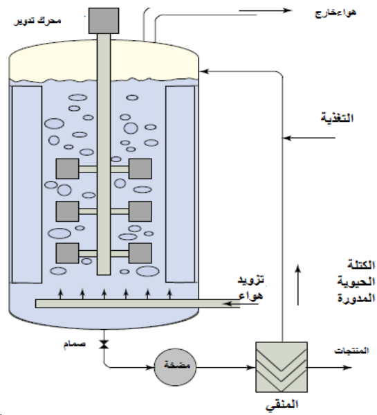
الشكل-7 . المخمر الحيوي:
