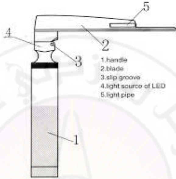
الشكل 5-24 منظار الحنجرة ذو النصلة المستقيمة (ميللر) .
