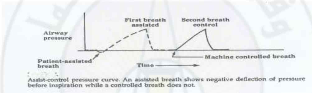
الشكل 22- 33 (منحنى ضغط التهوية الإجبارية- المساعدة )
