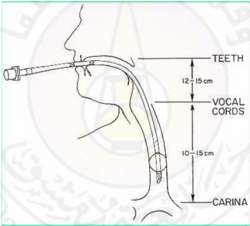
الشكل 5-40 أبعاد الأنبوب الرغامي الفموي عن تفرع القصبتين .
