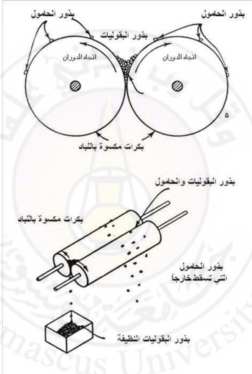
صورة. مخطط لجهاز البكرات متعكسة الدوران.
