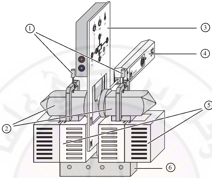
الشكل (5) : إعداد تجربة أثر هول في أنصاف النواقل
