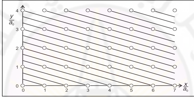
الشكل ( 5 ) : تمثيل ثنائي البعد لمجموعة المستويات البلورية (1 \ 3 \ 0) .
