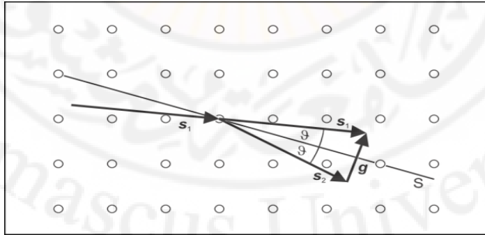
الشكل (3) : العلاقة الهندسية بين شعاعي الوحدة S_1 و S_2 ، والشعاع \vec{G} = \lambda \vec{g}
