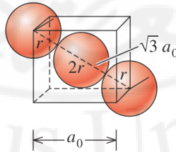
الشكل ( 2 ) : الارتصاص في النماذج المكعبة .
