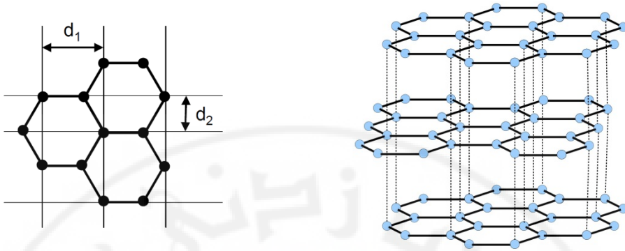
الشكل ( 4 ) بنية الغرافيت .
