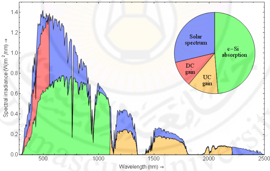
الشكل ( 4 ) : طيف الإشعاع الشمسي وطيف امتصاص السيلكون
