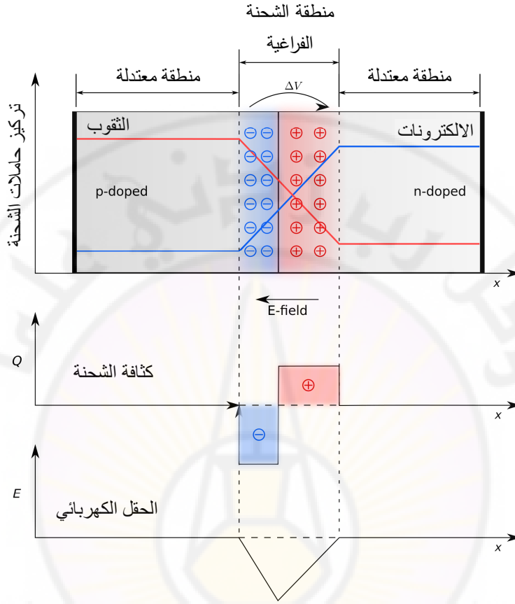
الشكل ( 2 ) : تركيز حاملات الشحنة وكثافة الشحنة والحقل الكهربائي في الوصلة .
