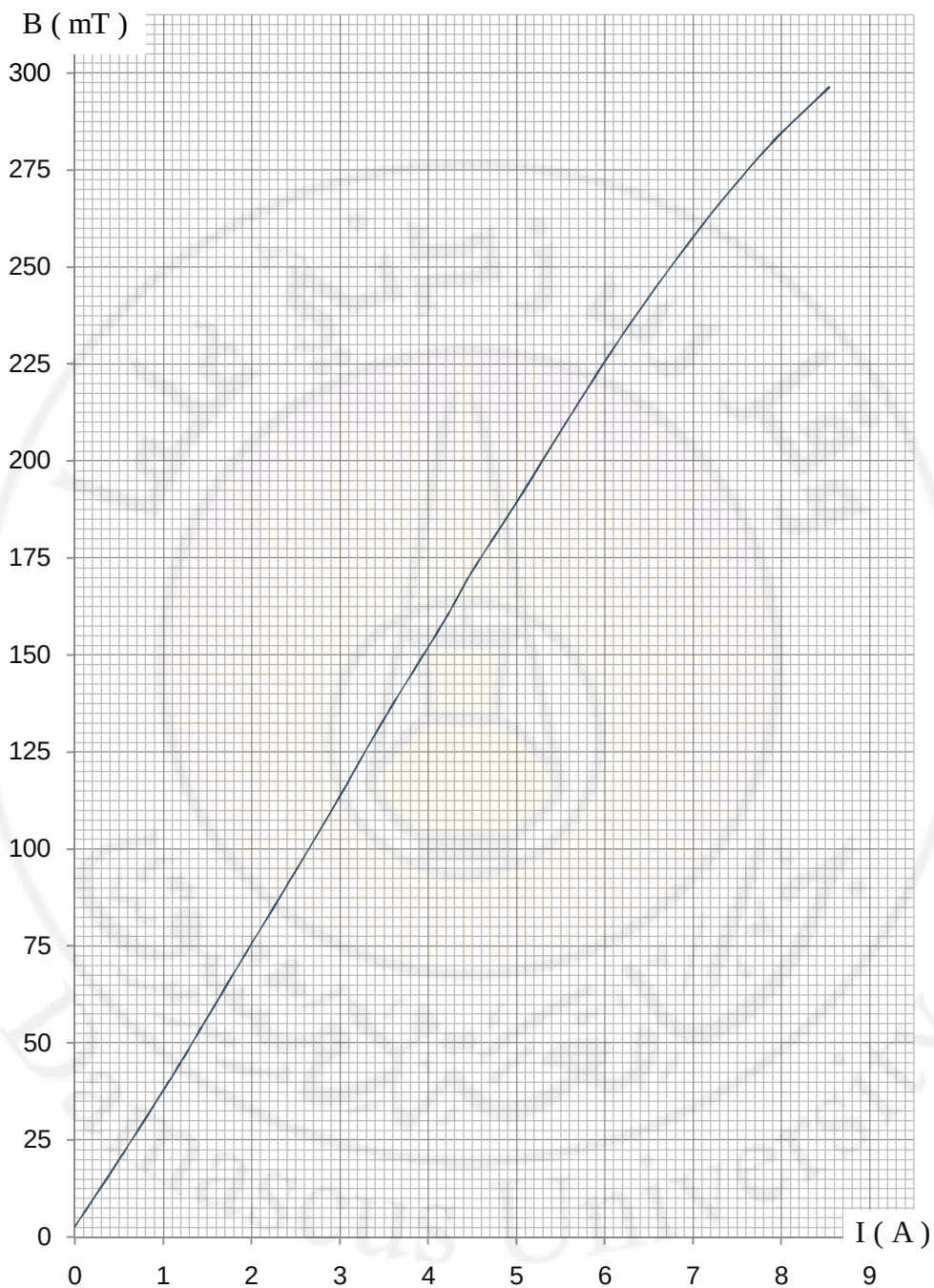
الشكل ( 4 ) : منحنى تغيرات B بدلالة I من أجل المسافة 16 mm بين القطبين المغناطيسيين
