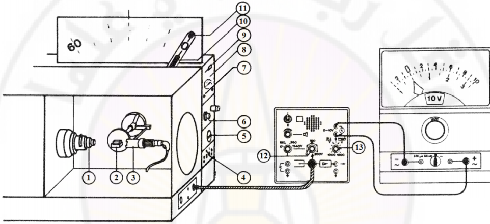
الشكل ( 8 ) : مطياف الأشعة السينية 554 90 وملحقاته
