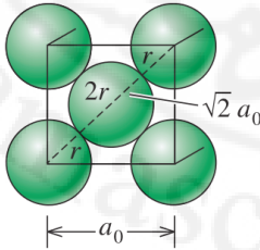
الشكل ( 2 ) : الارتصاص في النماذج المكعبة .
