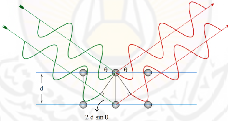
الشكل ( 1 ) : انعكاس الأشعة السينية عن المستويات البلورية .
