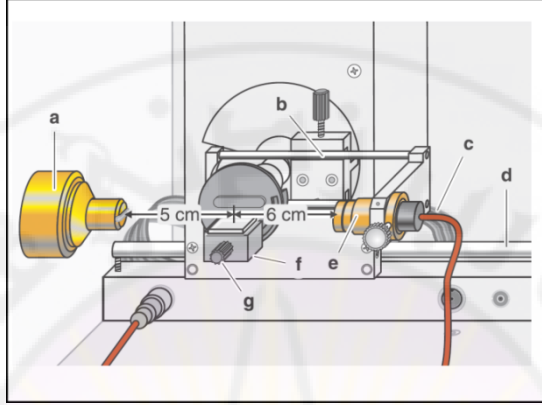
الشكل ( 6 ) الإعداد التجريبي لجهاز أشعة X- لاستخدامه بطريقة براغ .
