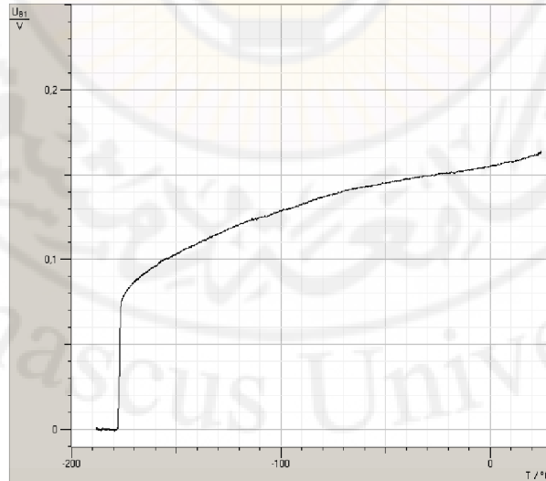
الشكل ( 1 ) : تغير مقاومة الناقل الفائق باعتبارها تابعاً لدرجة الحرارة .
