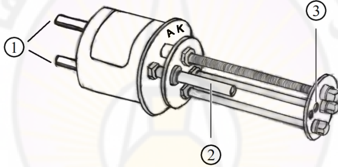
الشكل ( 1 ) : العينة المدروسة . 1: مربط العينة ، 2: أسطوانة تحوي العينة 3: فجوة لإدخال حساس درجة الحرارة .
