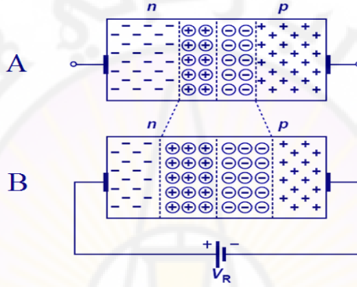
الشكل ( 4 ) : أثر الوصل العكسي على عرض منطقة النفاد .
