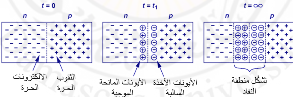
الشكل ( 1 ) : بدء تشكل منطقة النفاد .
