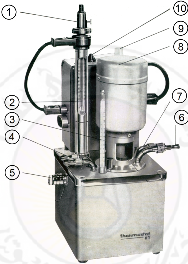
الشكل ( 5 ) : الأجزاء الرئيسية لجهاز تثبيت درجة الحرارة .
