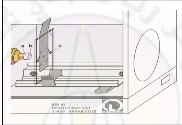
الشكل ( 10 ) الإعداد التجريبي : a: الحظار ، b: البلورة المدروسة ، c: الفيلم
