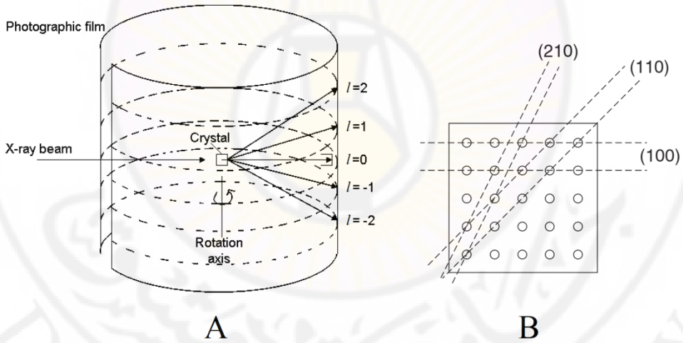
الشكل ( 2 ) A: طريقة البلورة الدوارة ، B: بعض المستويات البلورية المدروسة .
