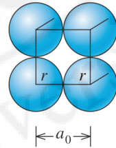
الشكل ( 2 ) : الارتصاص في النماذج المكعبة .
