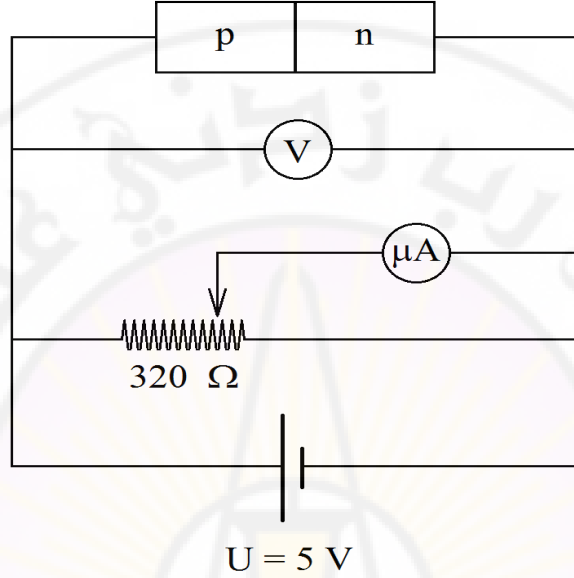
الشكل ( 6 ) : توصيل التجربة من أجل التغذية الأمامية .
