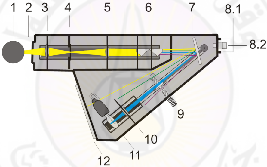
الشكل ( 1 ) : المطياف والحجرة الكهروضوئية .
