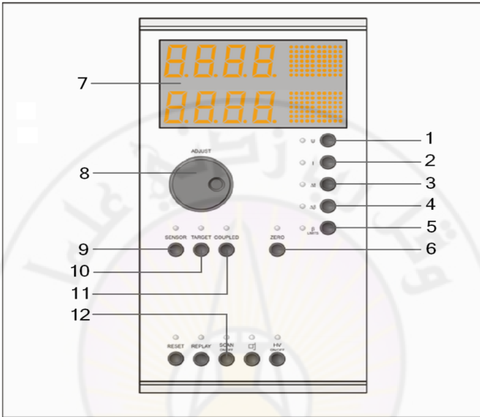
الشكل ( 5 ) : واجهة التحكم في منبع الأشعة السينية ( X-Ray apparatus ) .
